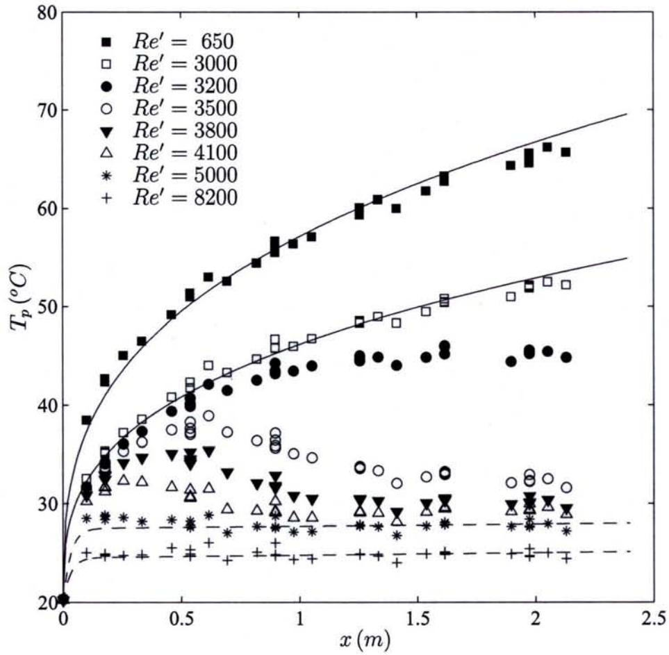
FIG. 5.9 – Evolution de la température de paroi en fonction de la distance à l'entrée pour une solution de Carbopol à 0,2% ( \tau_0 = 1 \text{ Pa} , K = 0,53 \text{ Pa}\cdot\text{s}^{-n} et n = 0,6 ) en écoulement dans une conduite cylindrique soumise à une densité de flux de chaleur constante ( \phi_p = 21,3 \text{ kW}\cdot\text{m}^{-2} ) à différents nombres de Reynolds ( 650 < Re' < 8200 )
