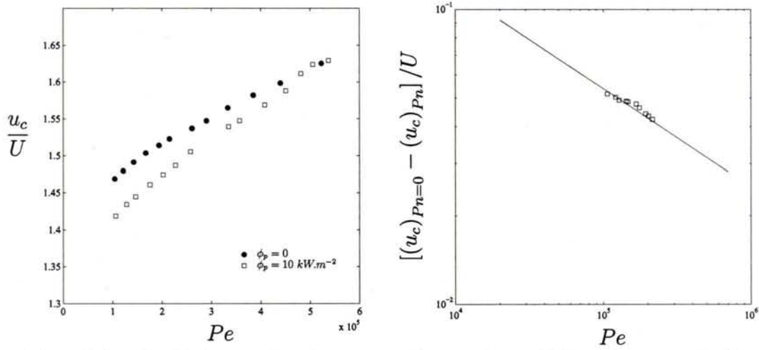
FIG. 5.4 – Evolution de la vitesse sur l'axe : (a) u_c/U en fonction de Pe pour \phi_p = 0 et \phi_p = 10 \text{ kW.m}^{-2} et (b) [(u_c)_{Pn=0} - (u_c)_{Pn}]/U en fonction de Pe , pour une solution de Carbopol à 0,2% ( \tau_0 = 16,3 \text{ Pa} , K = 9,2 \text{ Pa.s}^{-n} , n = 0.41 et b = 0,009^\circ\text{C}^{-1} )
