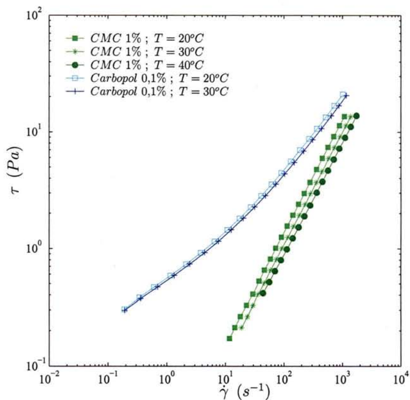
FIG. 1.5 - \tau(\dot{\gamma}) pour (i) une solution de Carbopol à 0,1% à T = 20 et 30^\circ\text{C} dont le comportement peut être décrit par le modèle de Herschel-Bulkley ( \tau_0 = 0,4 \text{ Pa} , K = 0,14 \text{ Pa}\cdot\text{s}^n , n = 0,7 et b \simeq 0,02^\circ\text{C}^{-1} ) et (ii) une solution de CMC à 1% à T = 20, 30 et 40^\circ\text{C} dont le comportement peut être décrit par le modèle de Ostwald-de Waele ( k = 63 \text{ mPa}\cdot\text{s} et n = 0,9 et b \simeq 0,02^\circ\text{C}^{-1} )
