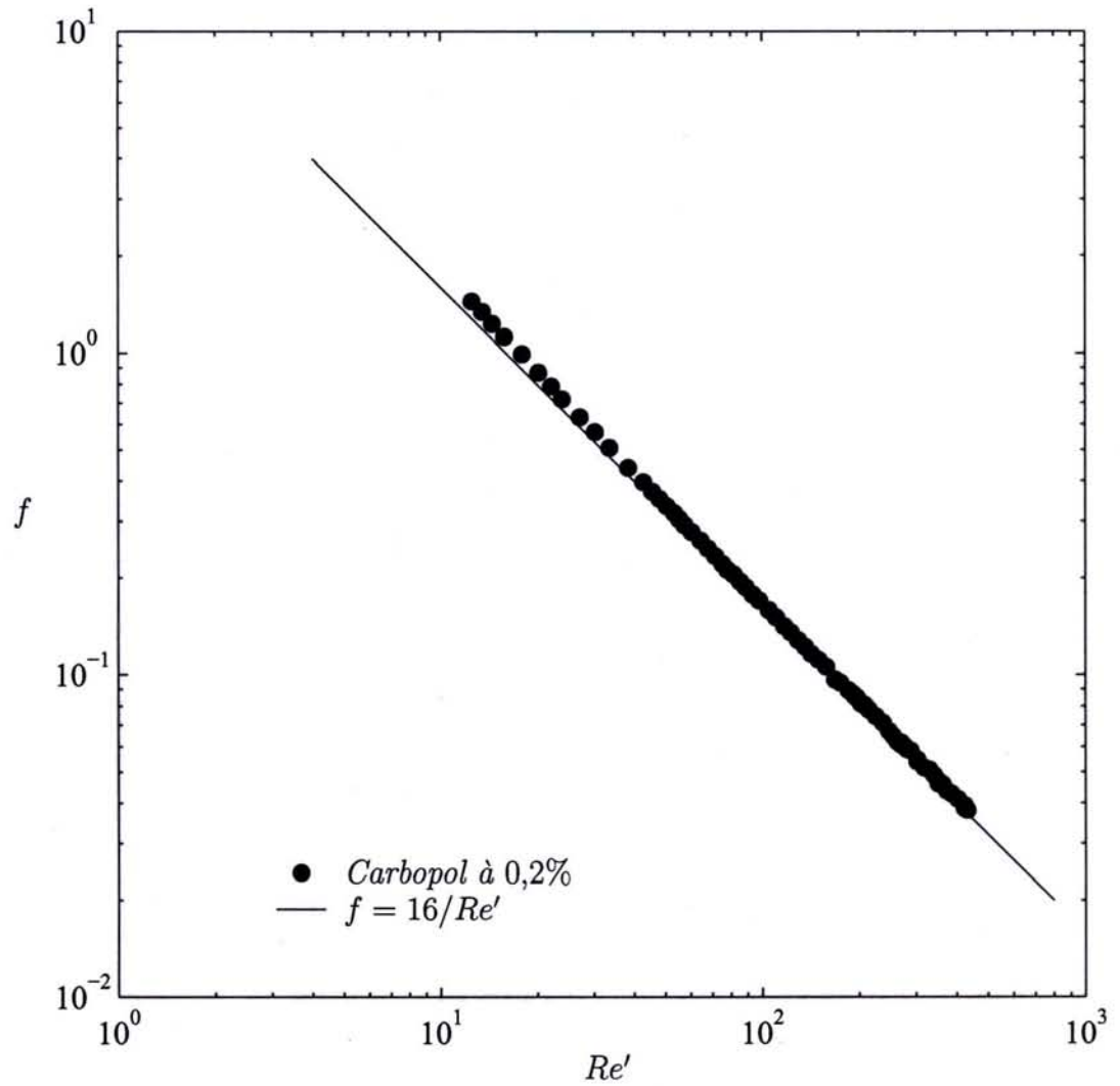
FIG. 2.10 – Coefficient de frottement en fonction du nombre de Reynolds pour une solution de Carbopol à 0,2% dont le comportement est décrit par le modèle de Herschel-Bulkley ( \tau_0 = 15 \text{ Pa} , K = 3,7 \text{ Pa}\cdot\text{s}^n et n = 0,34 ) en écoulement dans une conduite annulaire
