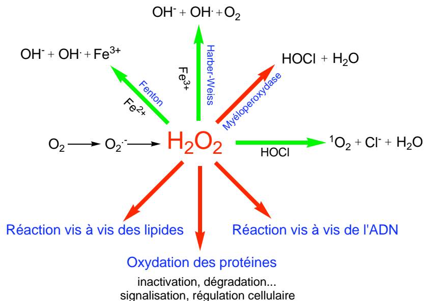
Figure 1 : Principales réactions issues de H_2O_2 .
