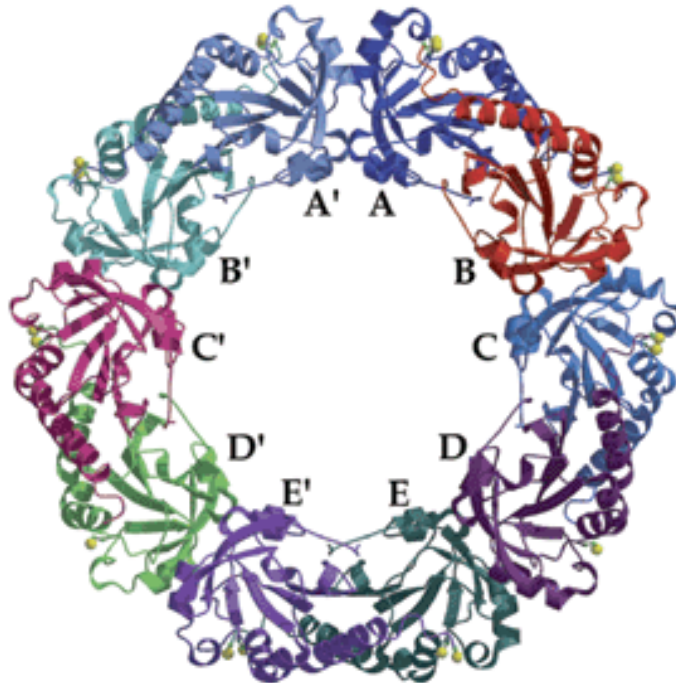
Figure 22 : Structure tridimensionnelle d'un décimère de 2-Cys Prx typiques, celle de AhpC de Salmonella typhimurium (d'après Wood et al. , 2002).
