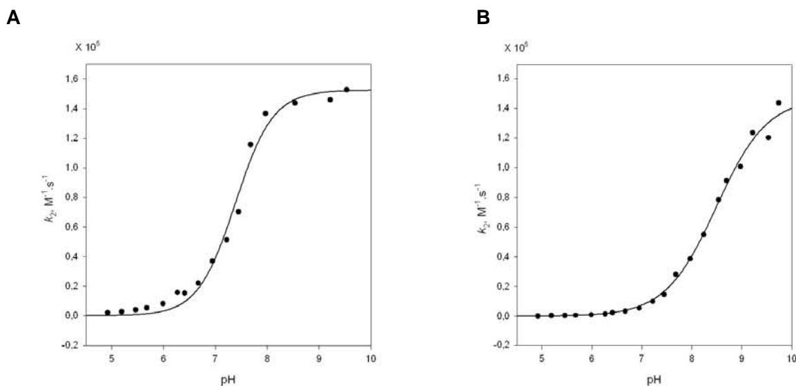
Figure 53 : Variation de la constante de second-ordre k_2 de la réaction des groupements thiols des variants C48A (A) et C84A (B) de scSrx avec le 2PDS, en fonction du pH.
