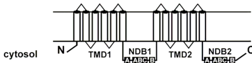
Figure 17 : Structure en 2 dimensions du transporteur ABCB1 [62].
