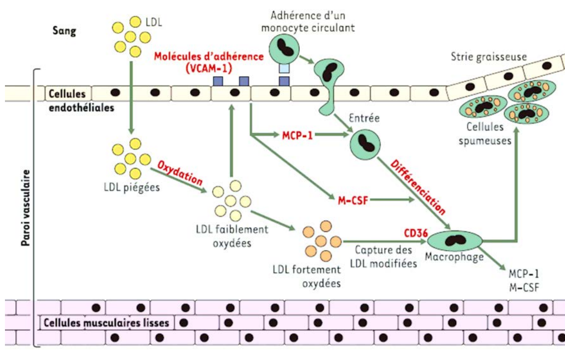
Figure 8 : Evolution de la formation de la plaque athérosclérotique [11].
