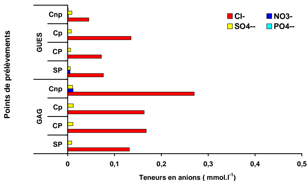
Figure 3.7: Teneurs en anions majeurs (mmol.l -1 ) des eaux prélevées aux différents: Source principale (SP) ; Canal principal (CP) ; Casier planté en riz (Cp) ; Casier non planté (Cnp) sur les sites de Gagnoa (GAG) et de Guéssihio (GUES)
