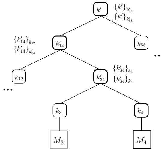
FIG. 2.3 – Ajout d'un membre M_4 par le protocole LKH
