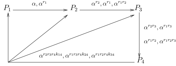
FIG. 3.4 – A-GDH.2 à quatre participants
