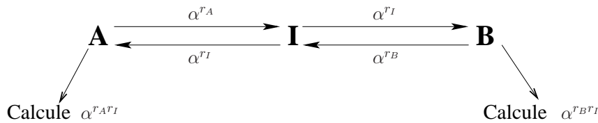
FIG. 4.2 – Attaque d'authentification sur le protocole DH
