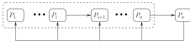
FIG. 5.1 – Protocoles de groupe : première situation
