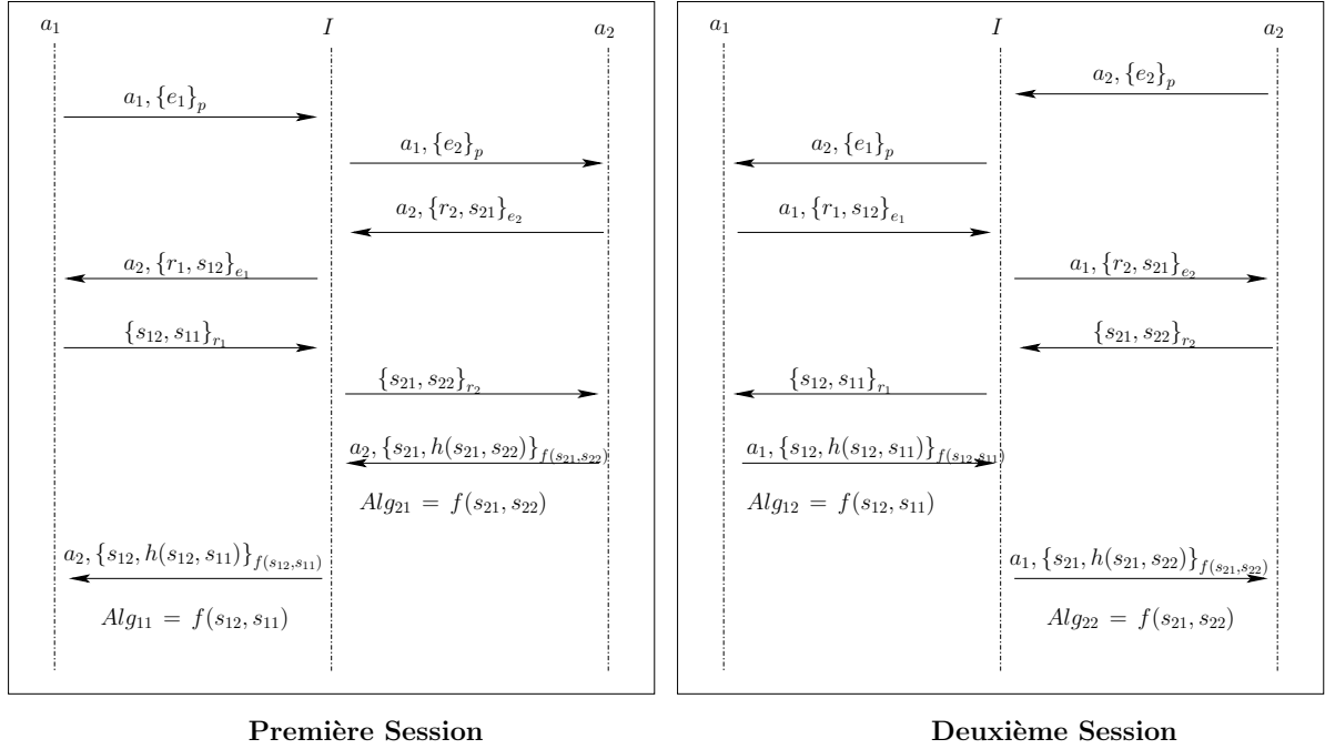
FIG. 4.8 – Attaque d'accord de clés sur le protocole Asokan-Ginzboorg
