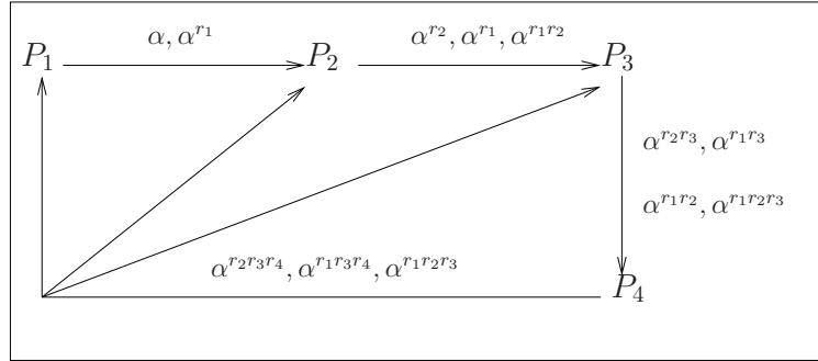
FIG. 4.9 – Le protocole GDH.2 avec 4 participants
