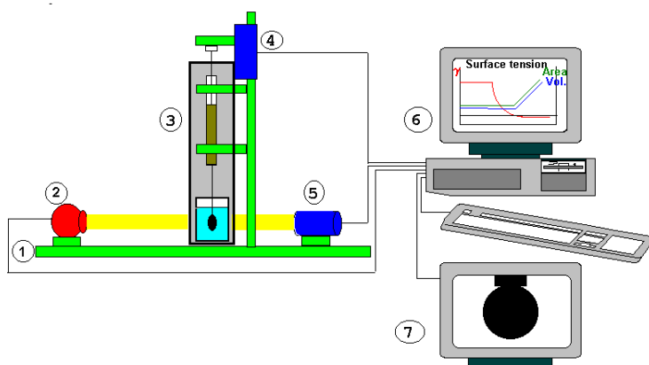
Figure II. 6 : Schéma du tensiomètre à goutte pendante (1 - Banc d'optique, 2 - Source lumineuse, 3 - Cellule de mesure thermostatée et/ou pressurisée, 4 - Pousse seringue, 5 - Optique et caméra, 6 - Ordinateur, 7 - Ecran de contrôle.)
