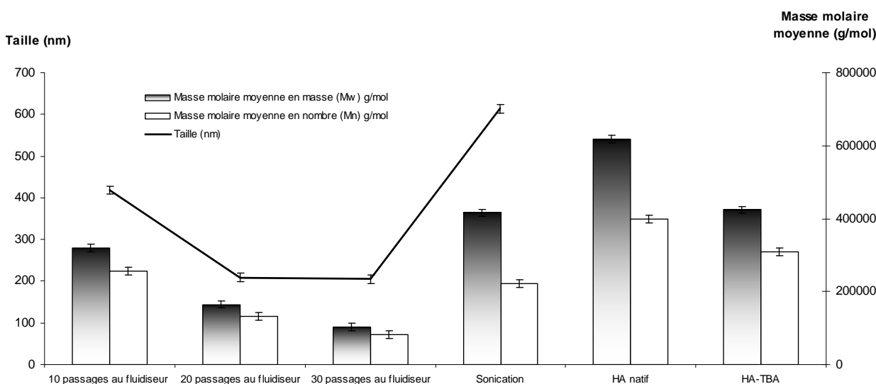
Figure III. 10 : Comparaison de l'effet des techniques d'émulsification (sonication et microfluidiseur à n passages) sur les masses molaires moyennes en nombre et en masse du HA-TBA et sur la taille finale de l'émulsion préparée en présence de HAC 6 . Les masses molaires moyennes du HA-TBA sont celles du polymère n'ayant pas subi l'étape d'émulsification. (A titre indicatif, on rappelle les valeurs de \overline{M}_n et \overline{M}_w du HA natif).
