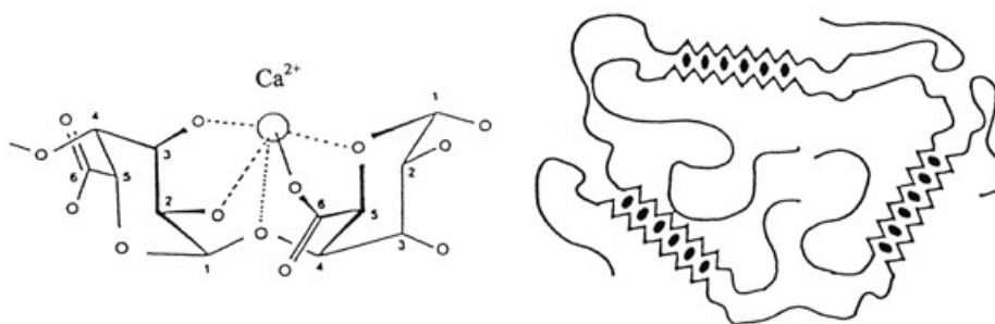
Figure IV. 1 : A gauche : Chélation des résidus guluronates de l'alginate par le calcium, à droite : représentation schématique du modèle « boîte à œufs »
