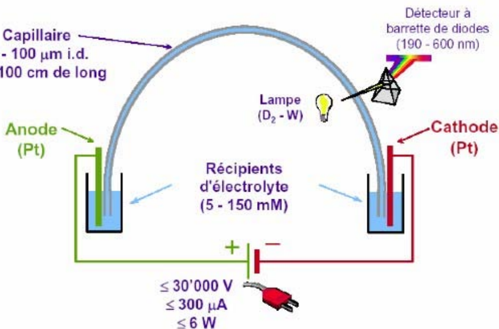
Figure III. 3 : Un appareil d'électrophorèse se compose d'un générateur, de deux électrodes, de deux réservoirs de solution tampon de part et d'autre d'un capillaire en silice et d'un détecteur.
