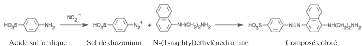
Fig. 22 : Principe du dosage des nitrites par le réactif de Griess. La formation du composé coloré est détectée à 570 nm.
