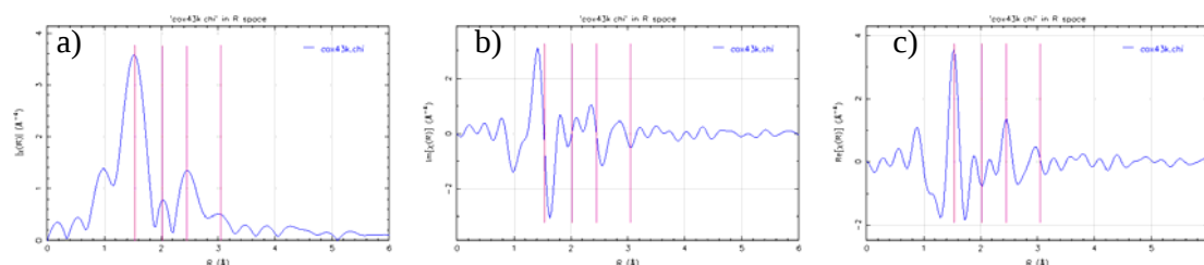
Figure 3.20 : Amplitude (a), partie imaginaire (b) et partie réelle (c) du spectre expérimental. Les positions des pics sont repérées par les traits verticaux.
