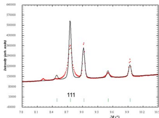
Figure 4.23 : Elargissement du pic 111, mal modélisé avec un modèle isotrope; Y_{\text{obs}} en rouge, Y_{\text{calc}} en noir.
