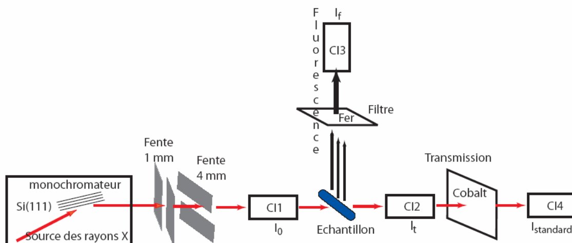
Figure B.4: Dispositif expérimental de mesure de spectre EXAFS sur la ligne BL17C1 (NSRRC, Taïwan).
