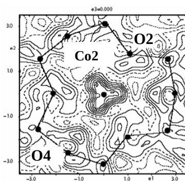
Figure 3.5: Densité résiduelle dans un plan perpendiculaire à l'axe 3 et passant par le site II. Contour de 0,1 \text{ e}^-/\text{\AA}^3 .
