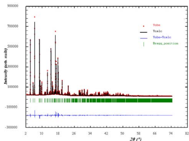
Figure 4.15 Affinement Rietveld du diffratogramme à 300 K ; Y_{\text{obs}} en rouge, Y_{\text{calc}} en noir, Y_{\text{obs}} - Y_{\text{calc}} en bleu et positions des pics de Bragg en vert.
