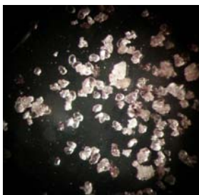
Figure 2.21: Cristaux du composite (thio-indigo@mordanite) (type 4, la longueur maximale des cristaux est \sim 100 \mu\text{m} selon [010]).
