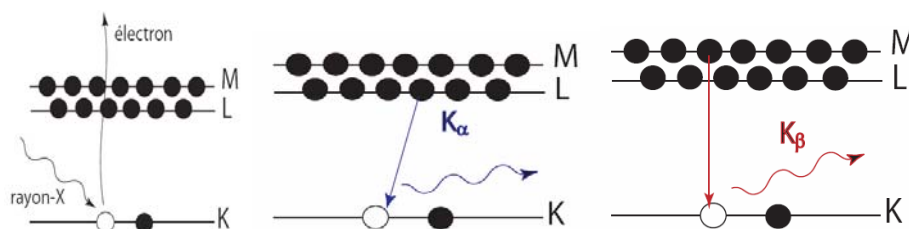
Figure B5 : Schéma du processus d'absorption des rayons X (à gauche) avec la fluorescence (à droite).
