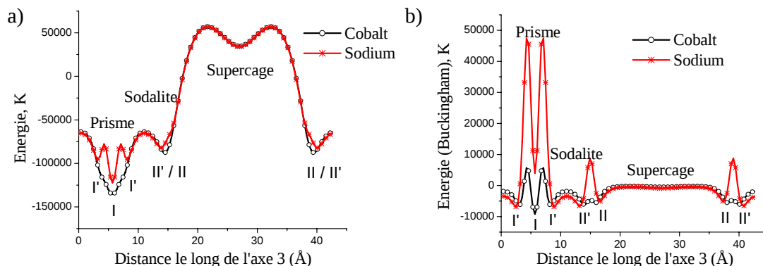
Figure 3.36 : Coupe d'énergie le long de l'axe 3 pour les cations Co 2+ et Na + dans une zéolithe déshydratée: a) contributions des énergies de Buckingham et Electrostatique; b) énergie d'interaction dispersion-répulsion (Buckingham).
