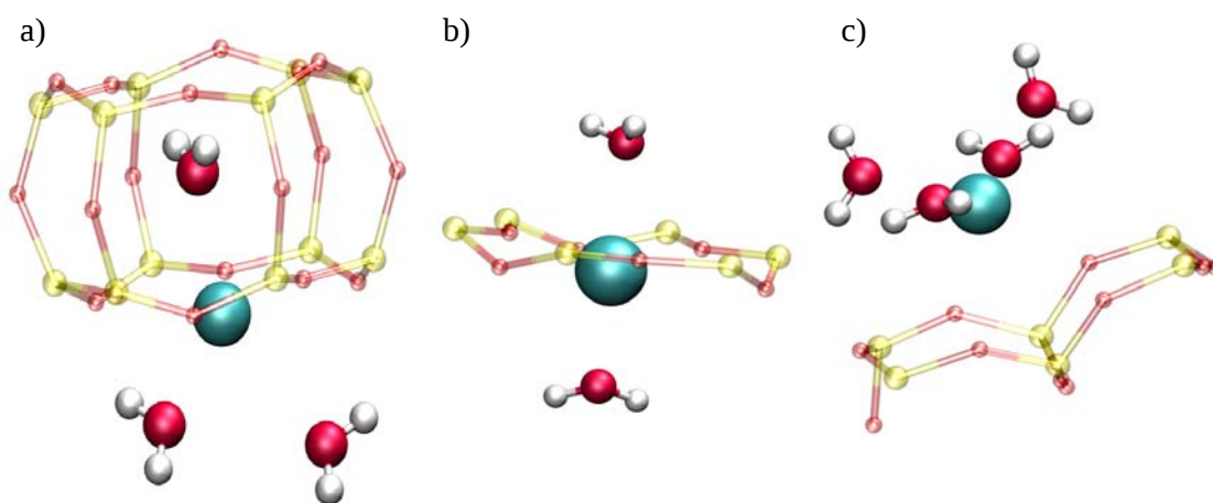
Figure 3.38 : Coordination des \text{Co}^{2+} (en bleu) en site I' (a), II (b), III' (c) dans une structure hydratée calculée ( \sim 243 \text{ H}_2\text{O}/\text{maille} )
