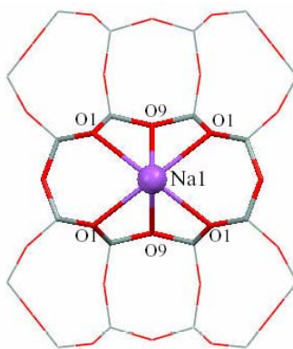
Figure 4.17 : Coordination de Na1 ; vue perpendiculaire à l'axe c
