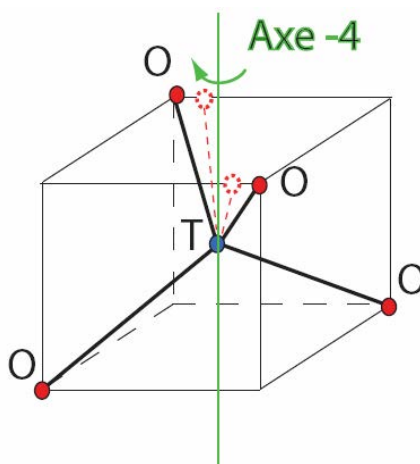
Figure 3.13 : T tétraèdre TO_4 régulier ( \bar{4}3m ) où toutes les distances T-O sont égales.
