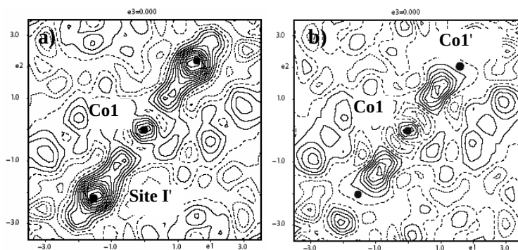
Figure 3.4: Cartes de Fourier-différence avant (a) et après (b) la modélisation de la densité résiduelle sur le site I' par un cation \text{Co}^{2+} . Contour de 0,1 \text{ e}^-/\text{\AA}^3
