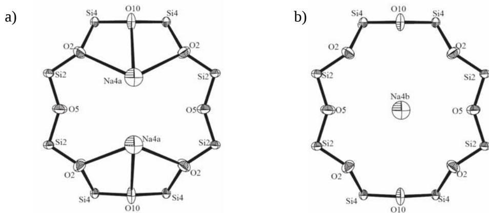
Figure 4.6 : Environnement de Na4a (a) et Na4b (b) ; vue perpendiculaire à l'axe b .
