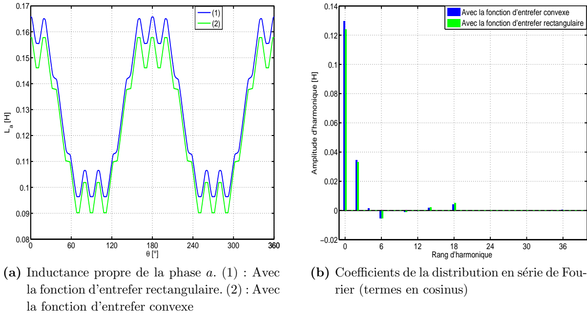
Figure II.10 – Inductance propre L_a(\theta) et sa distribution en série de Fourier
