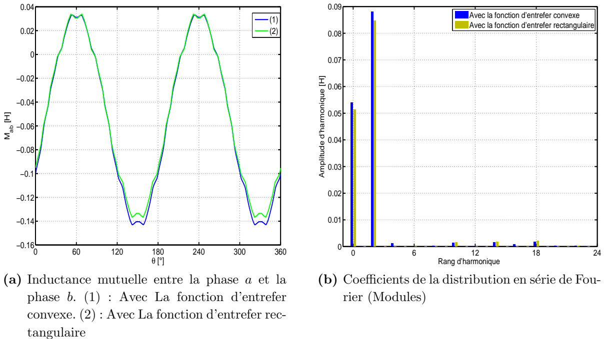
Figure II.11 – Inductance mutuelle M_{ab}(\theta) et sa distribution en série de Fourier
