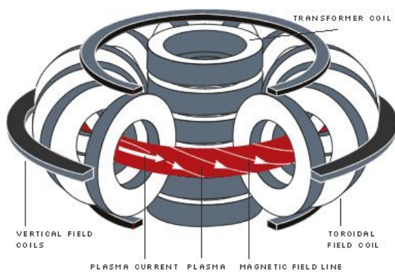
Fig. 1.1 – Schéma de principe de la configuration tokamak : bobines toroïdales et poloïdales, solénoïde central.
