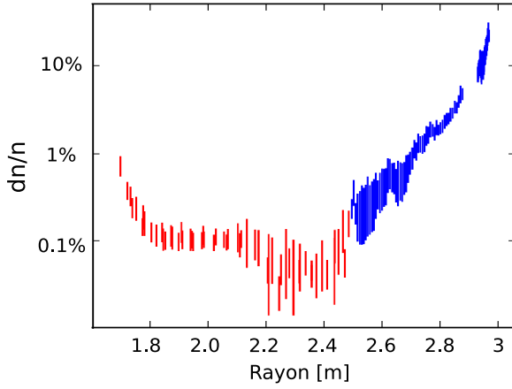
Fig. 5.6 – Profils radiaux du niveau de fluctuations de densité mesurés sur le même choc (TS #32398), par réflectométrie à balayage mode X (bleu), et par réflectométrie à fréquences fixes (rouge).
