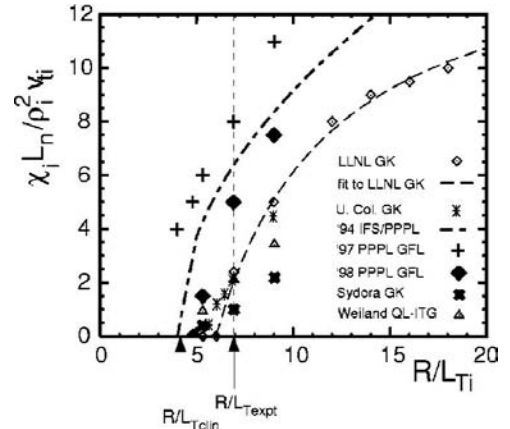
Fig. 5.19 – Mise en évidence numérique de seuils en L_{T_i} sur la diffusivité ionique pour des codes de simulation gyro-fluides et gyro-cinétiques, avec L_n fixés, [Dimits 00].
