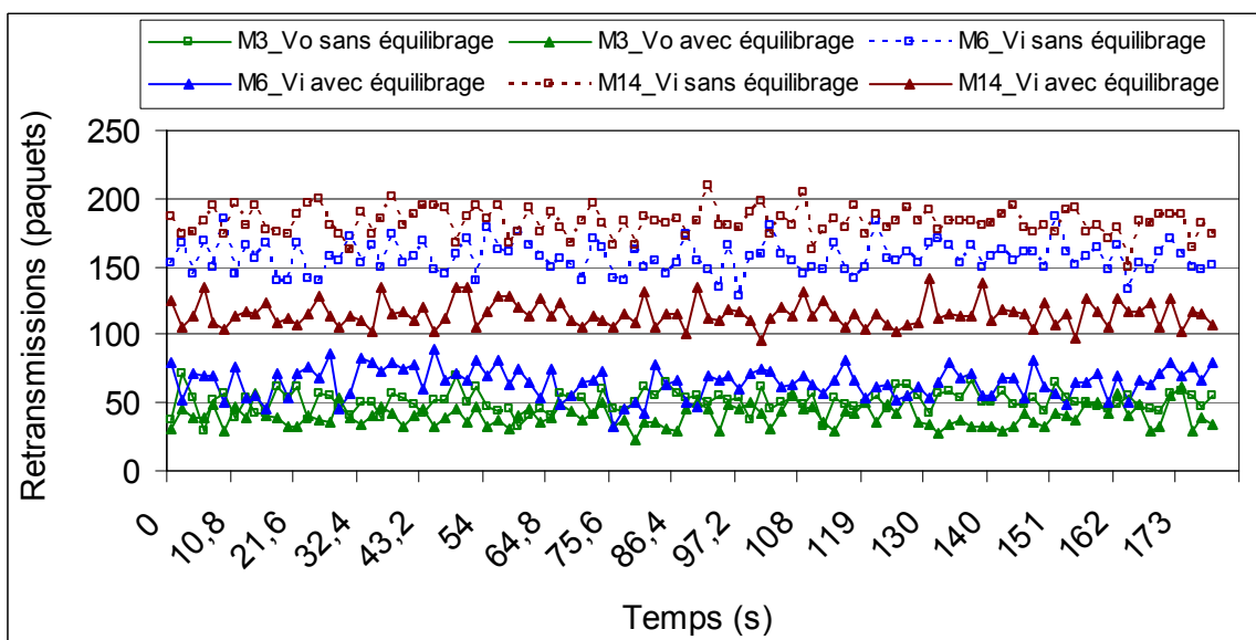
Fig. 4.18 Paquets retransmis
