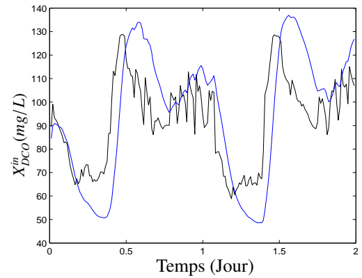
(d) La concentration X_{DCO}^in(mg/L)
