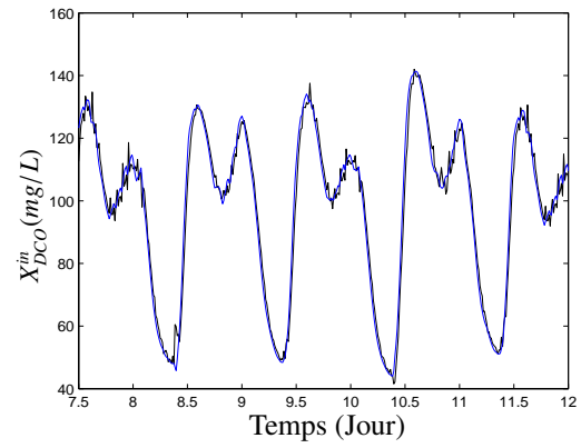
(d) La concentration de l'entrée inconnue X_{DCO}^in(mg/L)
