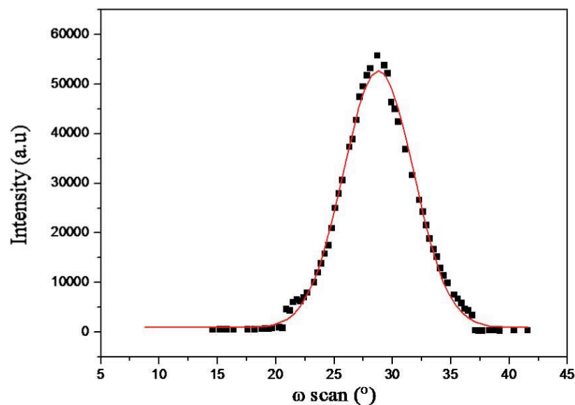
Figure 5.12 : La rocking curve du film d'AlN a axe c incline ( 10^\circ )
