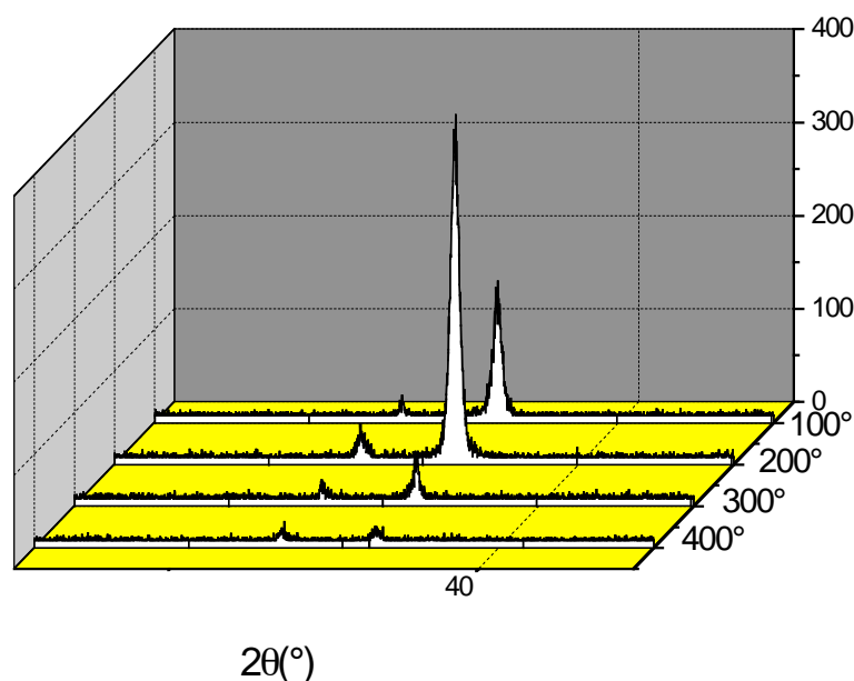
Figure 4.21 : Clichés de diffraction des échantillons déposés à différentes températures
