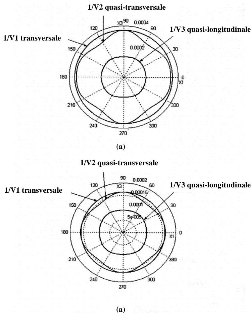
Figure 1.12 : Surface des lenteurs dans le plan (x_1x_3) : (a) cas du ZnO, (b) cas de l'AlN.
