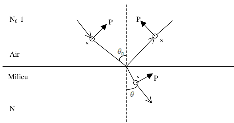
Figure 3.11 : Modèle d'un substrat nu
