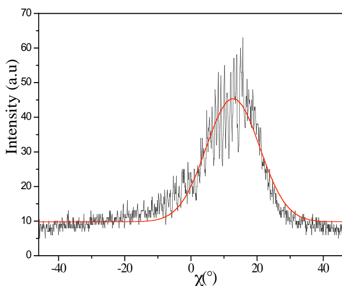
Figure 4.23 : Allure de la courbe typique de diffraction en mode \chi du film d'AlN présentant une inclinaison de 13^\circ \pm 2^\circ .
