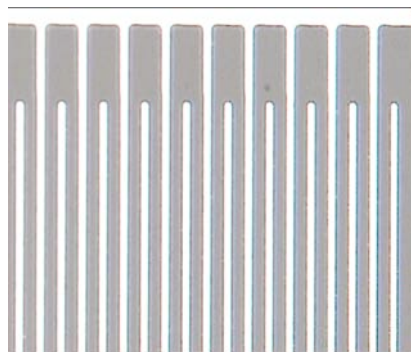
Figure 2.18: Image FESEM du transducteur interdigité
