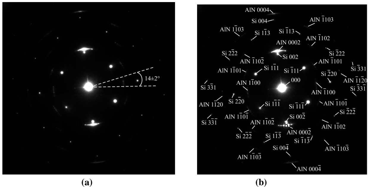
Figure 5.2 : Diffraction électronique : (a) sans indexation, (b) avec indexation
