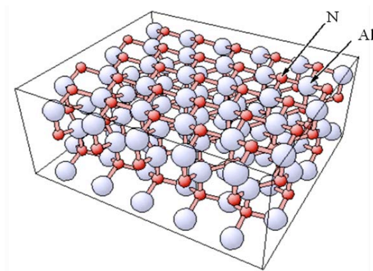
Figure 4.1 : Disposition des plans atomiques dans la structure hexagonale de l'AlN [20]
