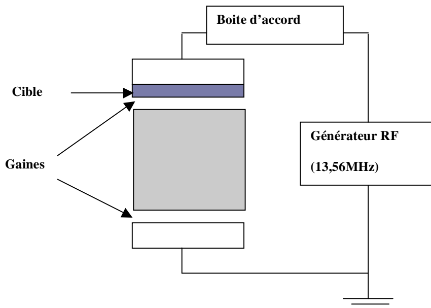
Figure 2.5 : Principe de la pulvérisation radio fréquence
