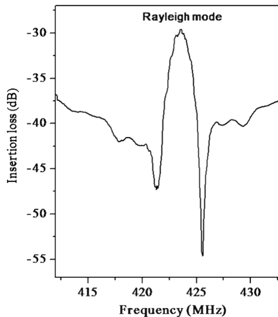
Figure 5.19 : Réponse fréquentielle d'un dispositif à base d'AlN à axe c perpendiculaire à la surface provenant de la zone 1 du wafer.
