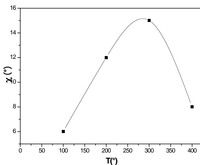
Figure 4.22 : Variation de l'inclinaison en fonction de la température
