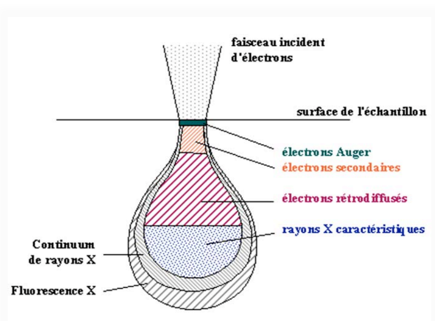
Figure 3.6 : Poire d'interaction électrons-matière expliquant le rôle de chaque type d'électrons dans le processus [17]
