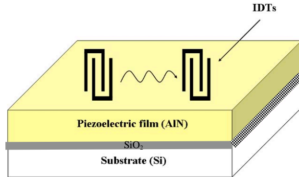
Figure 5.17 : Schéma d'un dispositif à onde acoustique de surface
