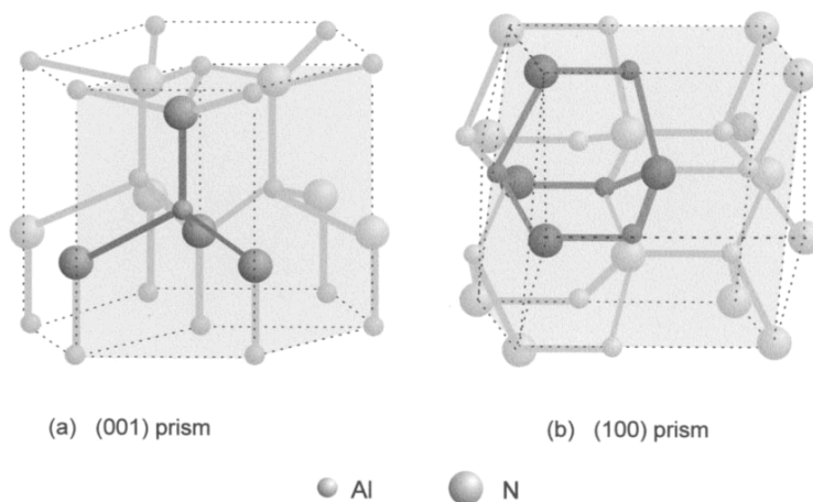
Figure 4.10 : Schéma de croissance des films d'AlN de type (001) et (100).
