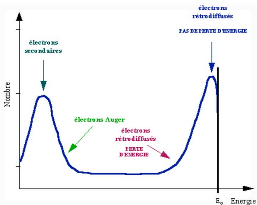
Figure 3.7 : Représentation schématique de l'énergie de distribution des électrons émis par un échantillon [17]
