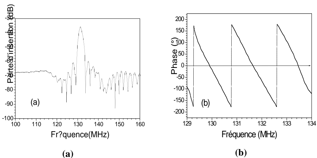
Figure 5.15 : Réponse fréquentielle d'un filtre SAW à base de quartz Y-X : (a)gain, (b) phase dans la bande passante
