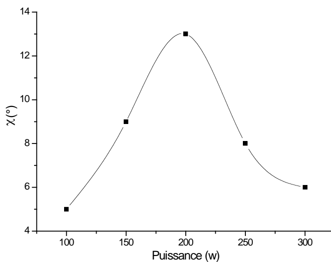
Figure 4.26 : Variation de l'inclinaison de l'axe c en fonction de la puissance de décharge obtenues par diffraction X en mode \chi .
