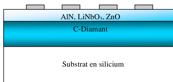
Figure 1.7 : Les différentes couches d'un dispositif à onde acoustique de surface en multicouches
