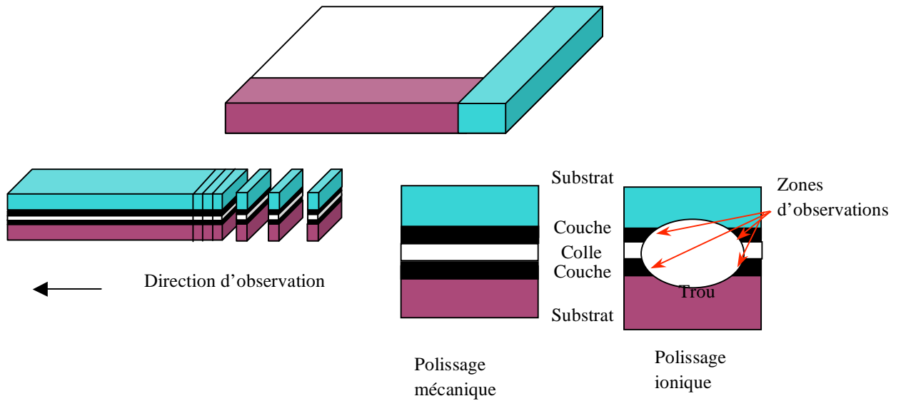
Figure 5.1 : Mode de préparation des échantillons d'AlN caractérisés par TEM
