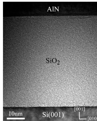
Figure 5.9: Cliché haute-résolution montrant les interfaces AlN/ SiO 2 et SiO 2 /Si(001).
