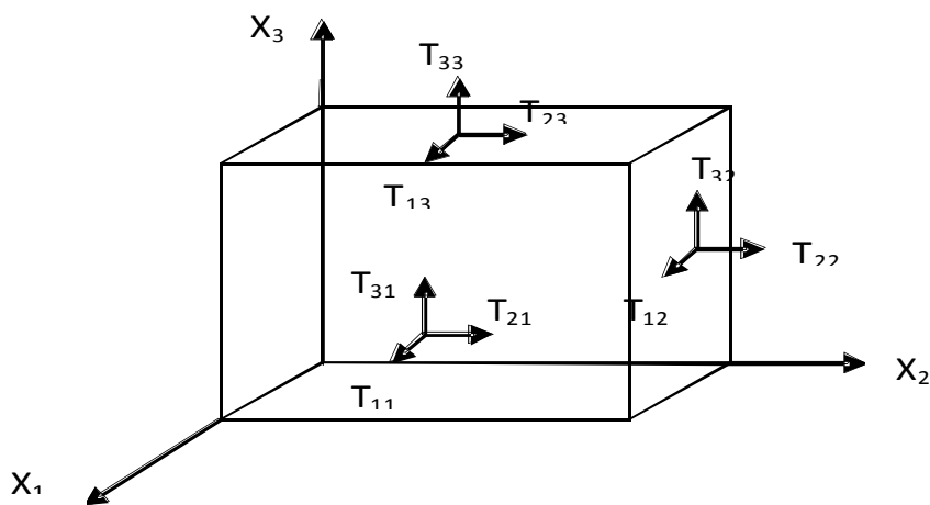
Figure 1.10 : Représentation des contraintes $T_{ij}$.
