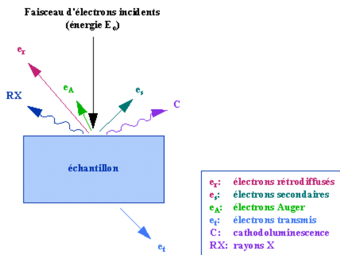
Figure 3.5 : Représentations schématique de l'interaction entre un faisceau d'électrons et la surface d'un échantillon.
