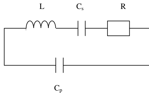
Figure 1.15 : Schéma électrique équivalent d'un résonateur FBAR
