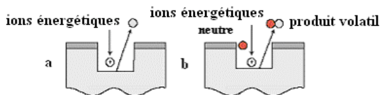
Figure 2.17 : illustration des mécanismes de gravure dans le cas de gravure sèche:
