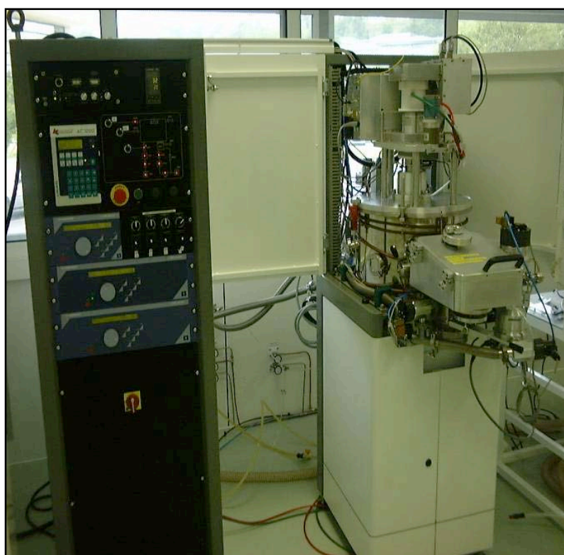
Figure 4.3 : Système de pulvérisation magnétron (ac450)
