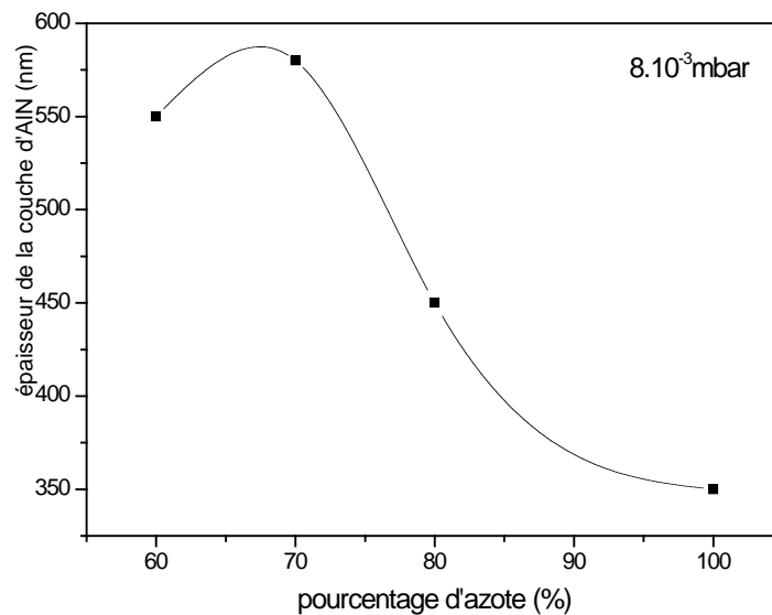
Figure 4.20 : Variation de l'épaisseur des couches en fonction du pourcentage d'azote
