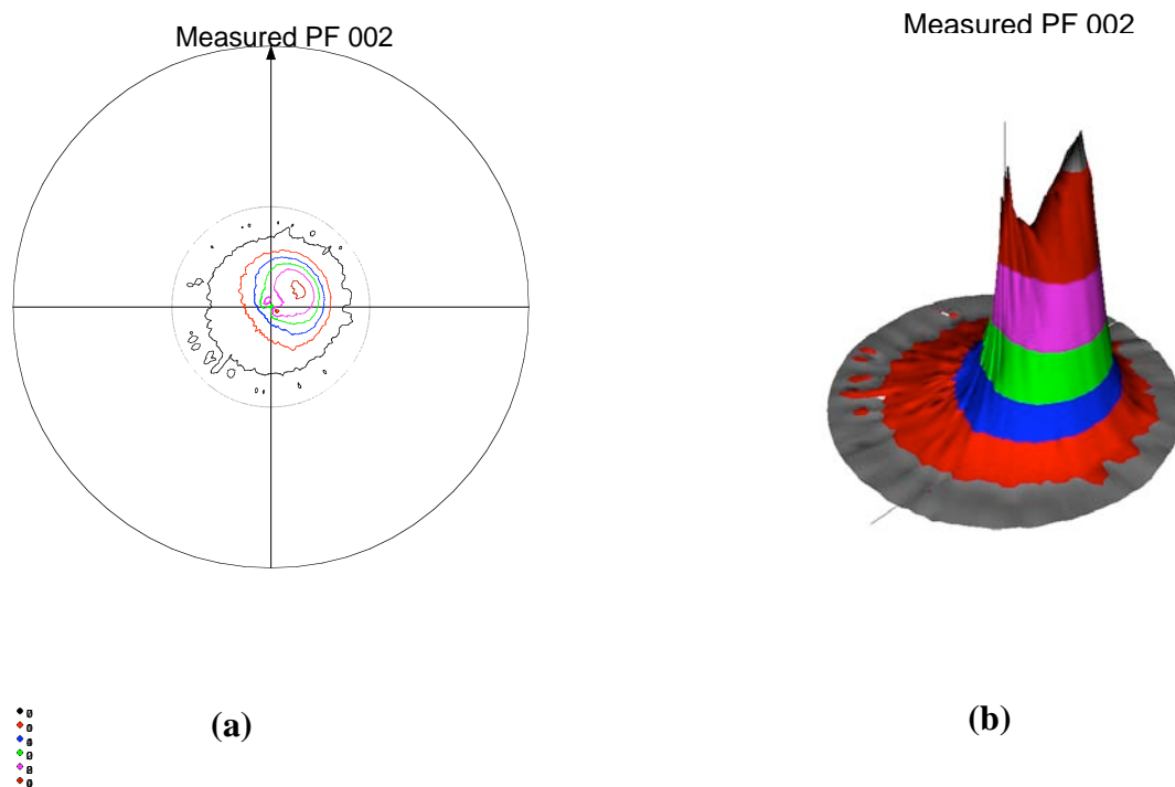
Figure 4.24 (a, b) : Figures de pôles en 2D et 3D de l'échantillon ayant présenté une inclinaison de 13^\circ \pm 2^\circ .
