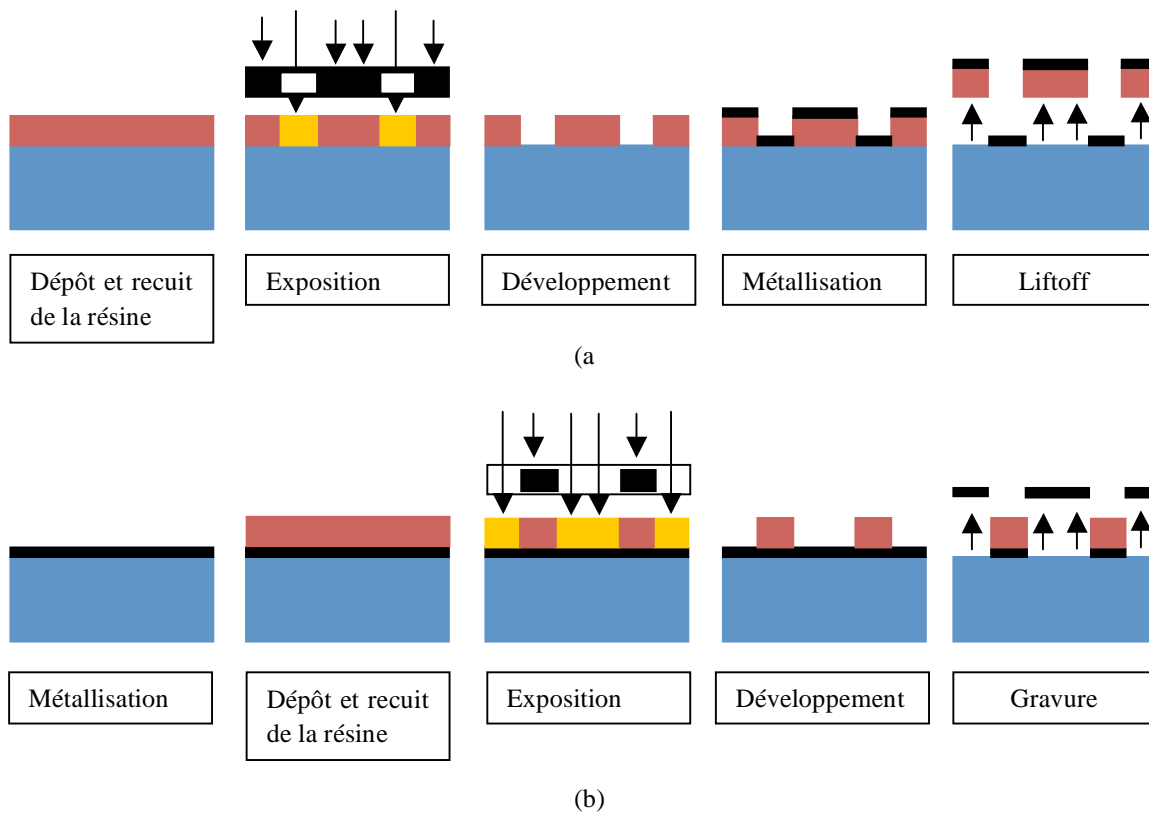
Figure 2.15 : Procédé de photolithographie. (a) Liftoff. (b) gravure.
