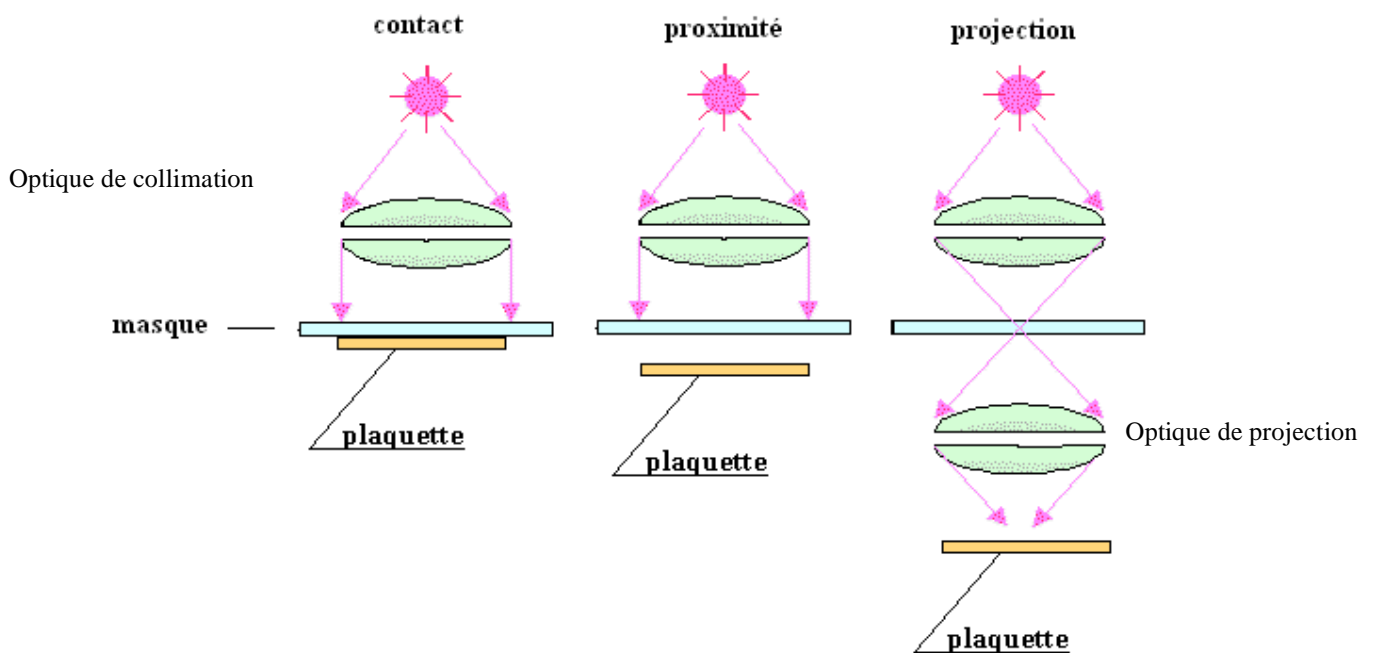
Figure 2.10.a : Différentes techniques d'insolation par contact, par proximité et projection.
