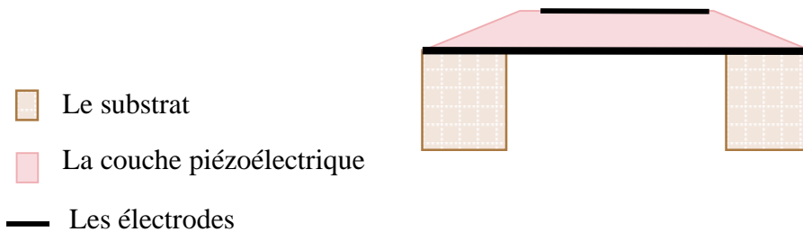
Figure 1.8.a : Dispositif à ondes acoustiques de volume de type FBAR (Film Bulk Acoustic Resonator)
