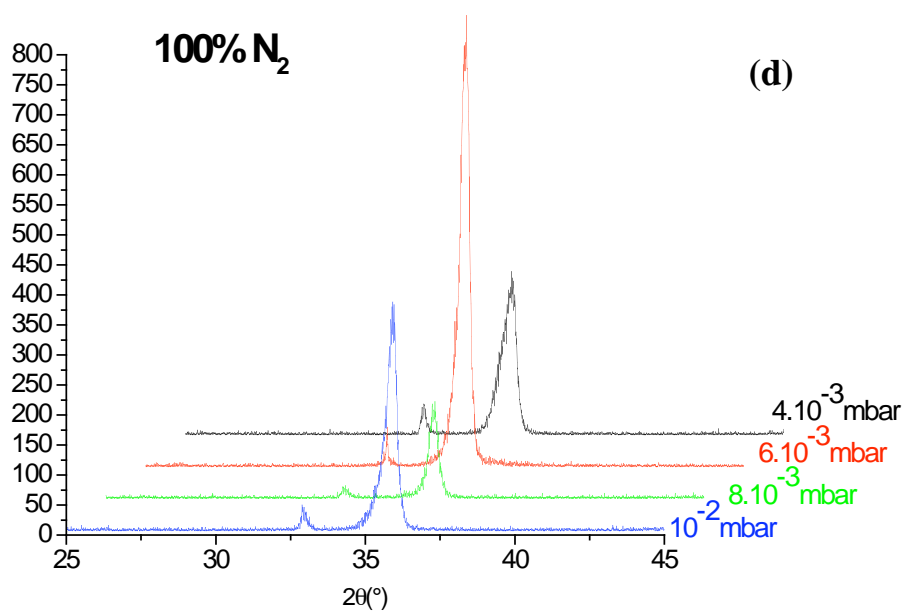
Figure 4.9 (a, b, c, d) : Clichés de diffraction X des échantillons déposés à des pressions variables avec une puissance de 200W et une température de 200°C à 60%, 70%, 80% et 100% N 2 .
