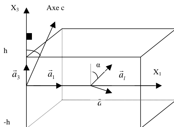
Figure 1.13 : FBAR simple avec AlN à axe c incliné d'épaisseur 2h avec des électrodes d'épaisseurs infinitésimales
