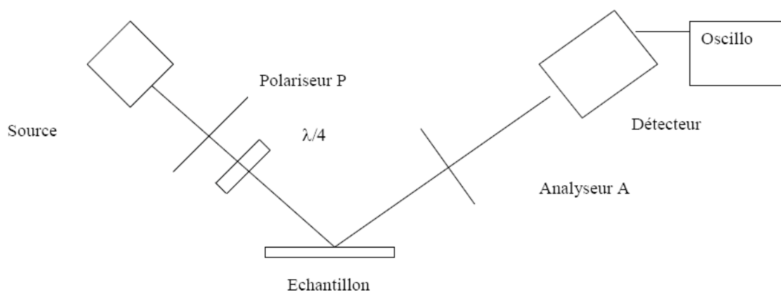
Figure 3.12: Les différents composants du système d'ellipsométrie spectroscopique
