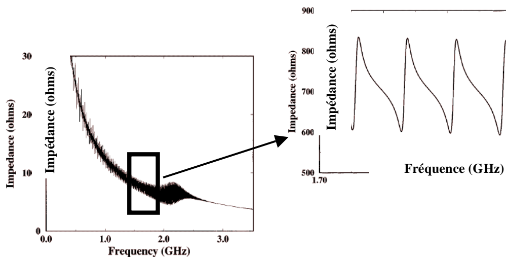
Figure 1.17 : Réponse fréquentielle dans les résonateurs à mode supérieur.
