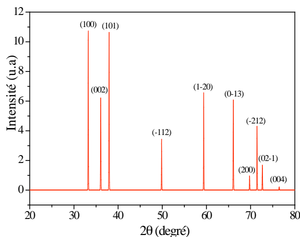
Figure 4.2.a: Phase hexagonale wurtzite du nitrure d'aluminium.
