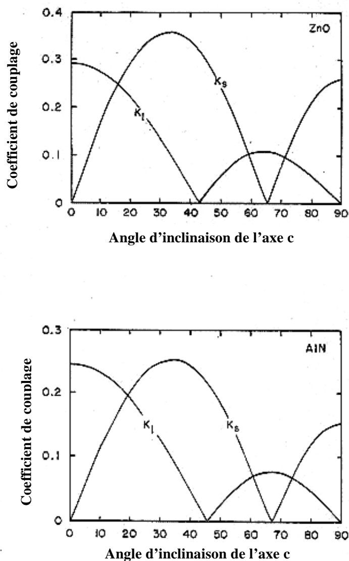
Figure 1.14 : Variation du couplage électromécanique en fonction de l'angle d'inclinaison de l'axe c [25].
