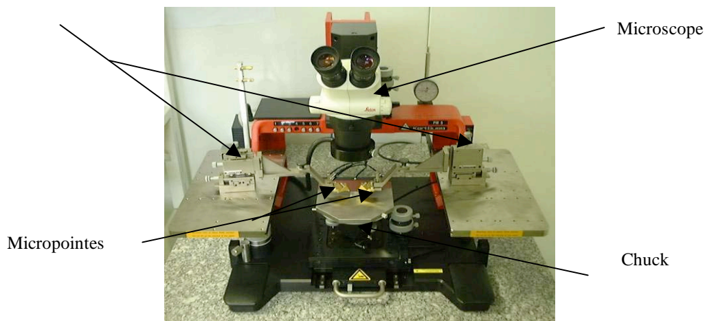
Figure 5.14 : Testeur sous pointes Karl Suss PM 5
