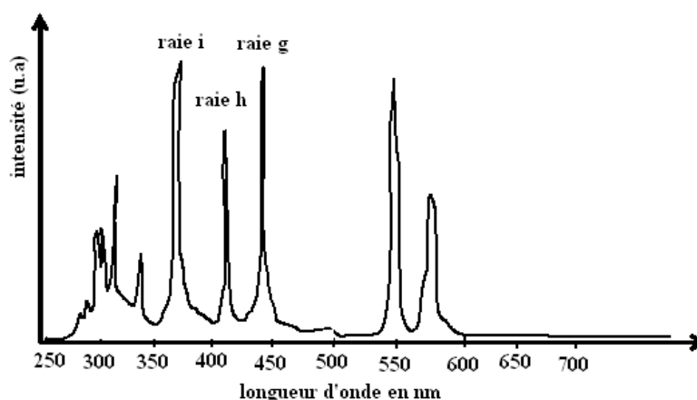
Figure 2.12 : Spectre d'une lampe UV à vapeur de mercure : les raies i, h et g ([19]).
