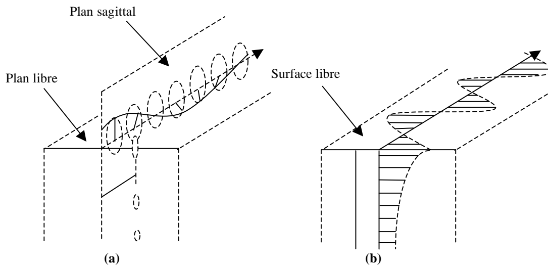
Figure 1 (a) : Onde de Rayleigh (longitudinale) se propageant à la surface d'un matériau isotrope [10],
