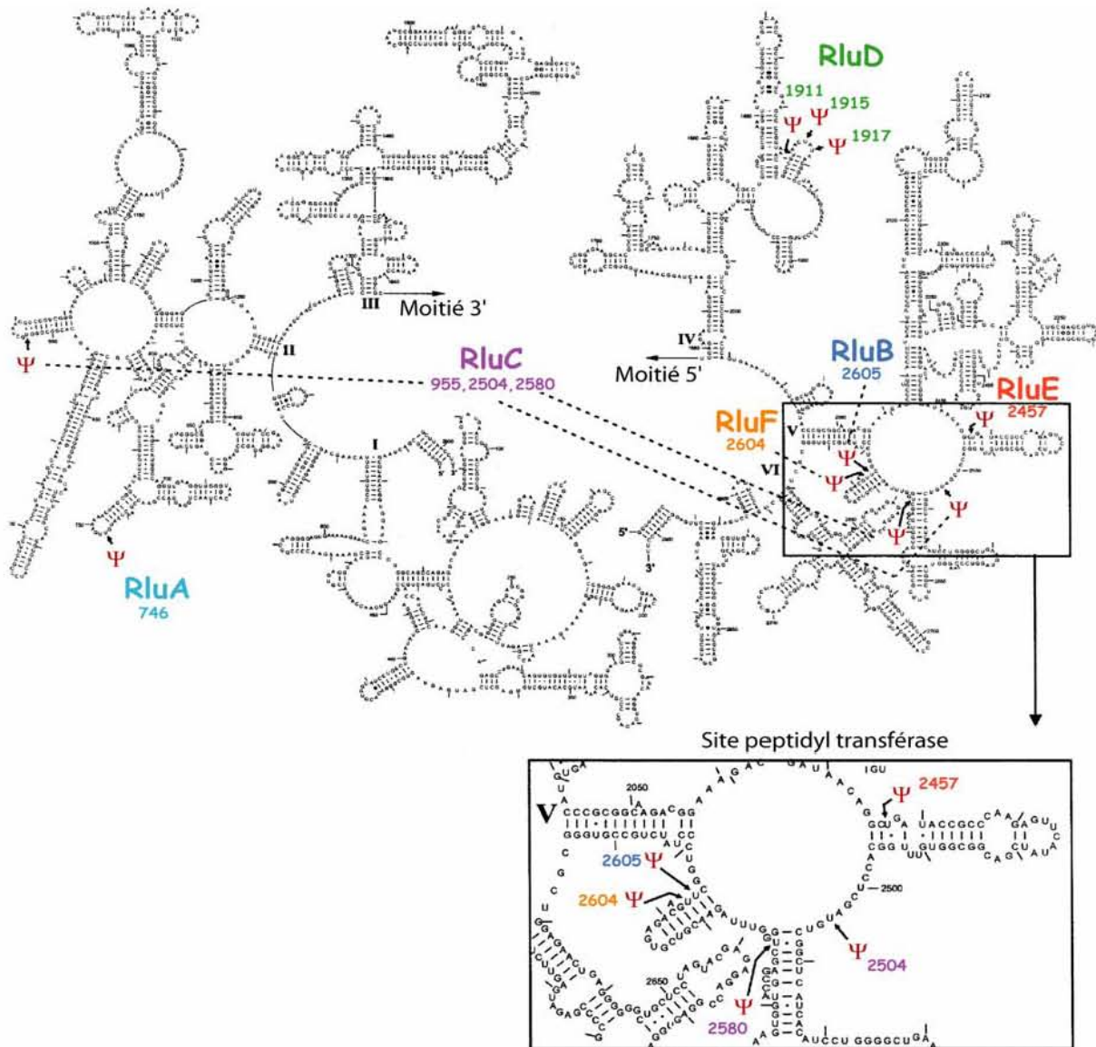
Figure 40 : Les cibles des ARN:Ψ-synthases d' E. coli au sein de l'ARNr 23S (d'après (Del Campo et al., 2001)).
