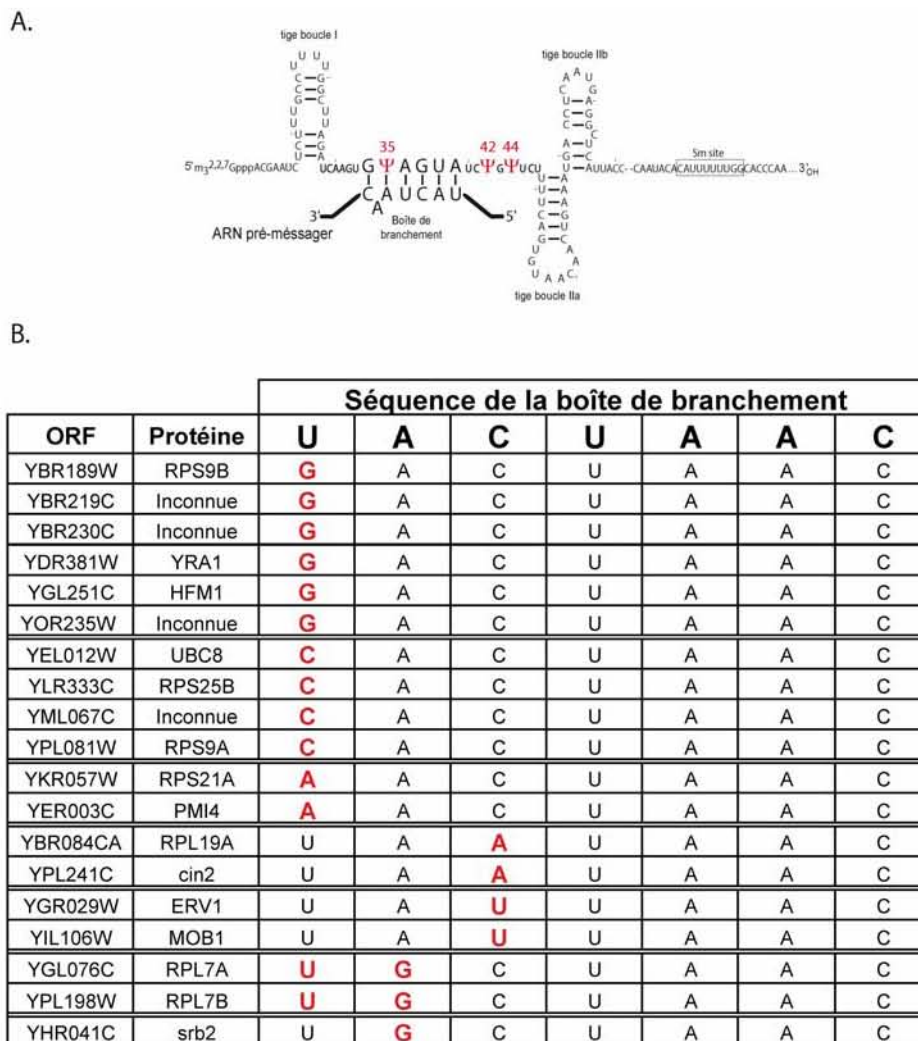
Figure 85 : Lien possible entre la présence de résidus \Psi dans le snRNA U2 et la stabilité de son appariement avec la boîte de branchement des introns de S. cerevisiae .
