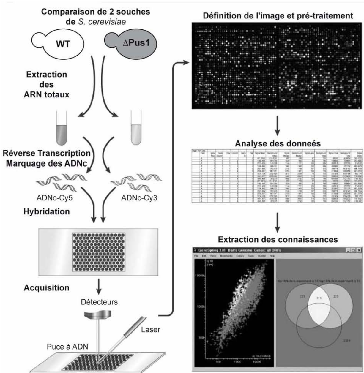
Figure 93 : Schéma de principe des expériences à base de puces à ADN.
