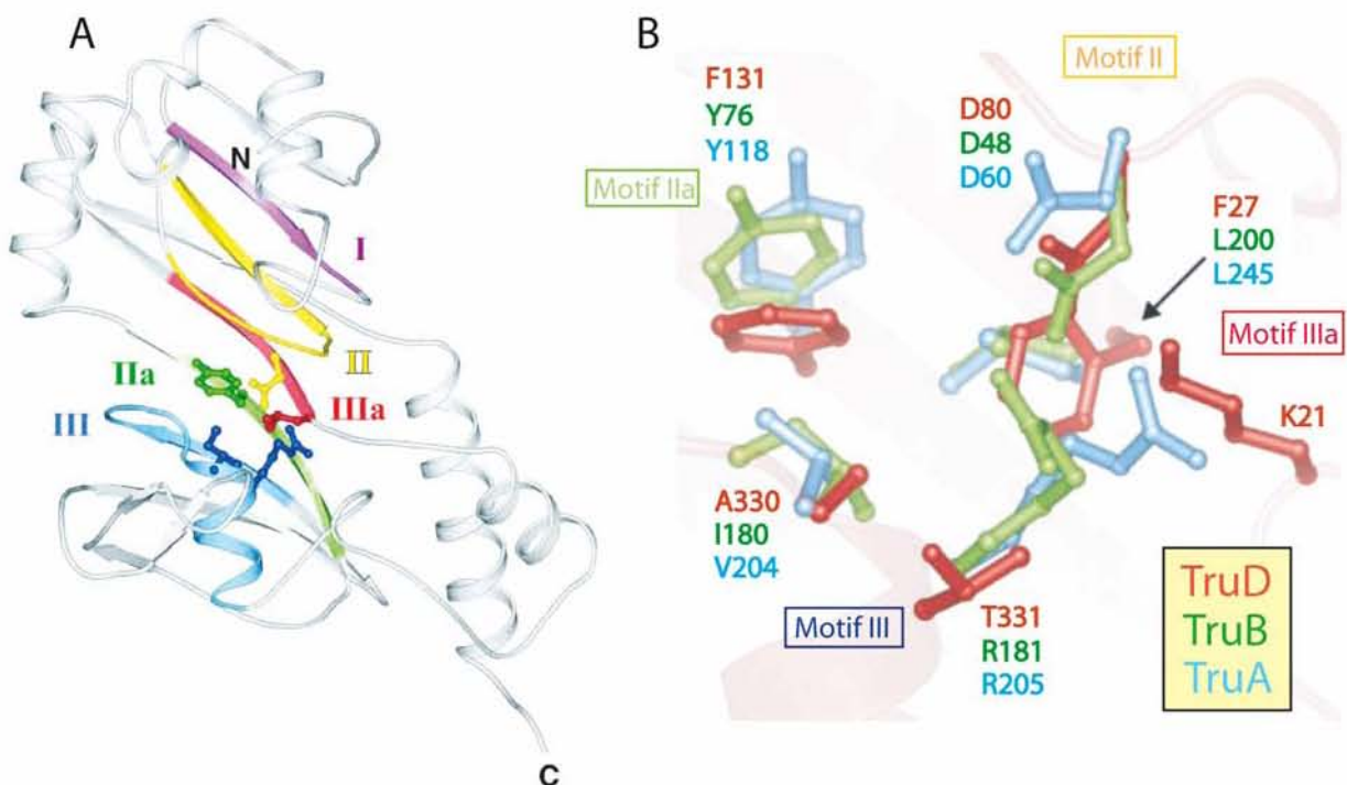
Figure 35 : Caractéristiques structurales communes à l'ensemble des ARN:Ψ-synthases.
