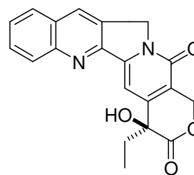
Camptothecin
