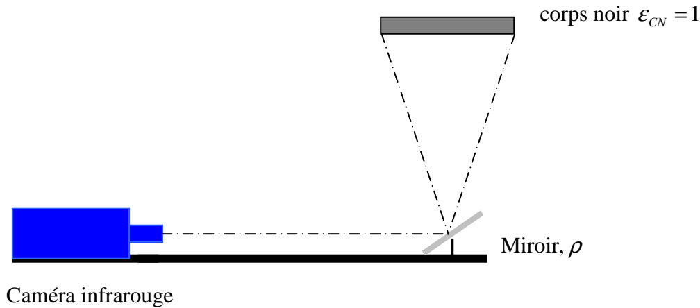
Figure 2.8 : Schéma de la configuration.
