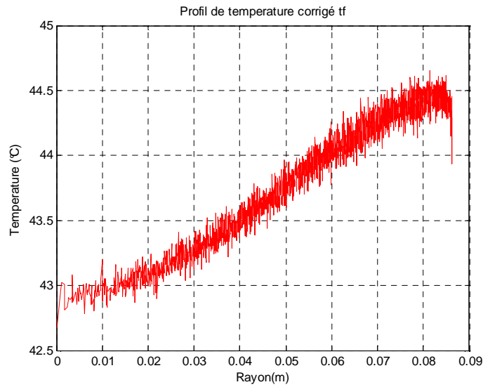
Figure 4.15: Profil de température corrigée à t_f = 7600 s .
