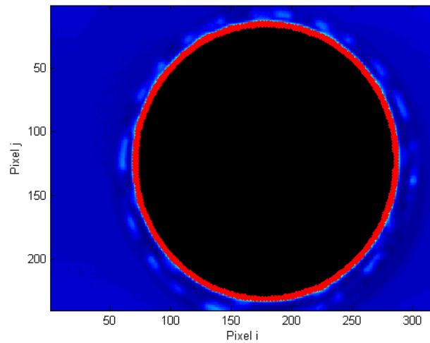
Figure 4.8 : Image thermographique de la rondelle après le second seuillage.
