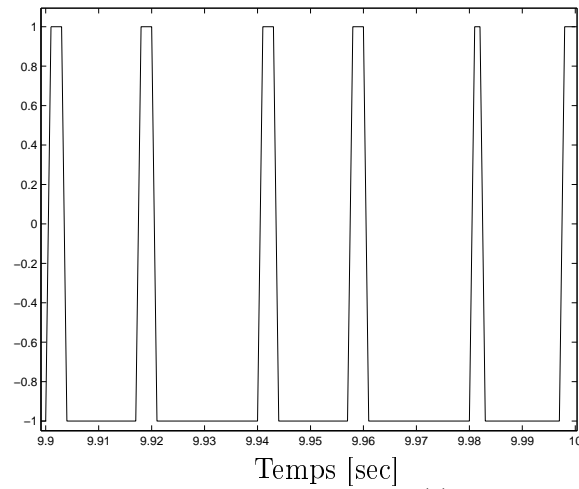
FIG. 3.1: Entrée u_1(t)
