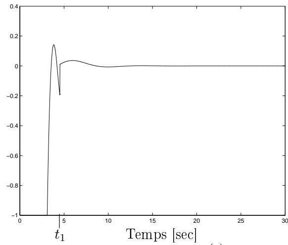
FIG. 3.33: Entrée u(t)
