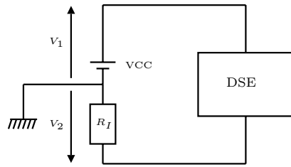
(a) Mod ele de base du banc d'essai.
