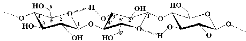
Figure 5. Formation de liaisons hydrogène intramolécules dans la cellulose
