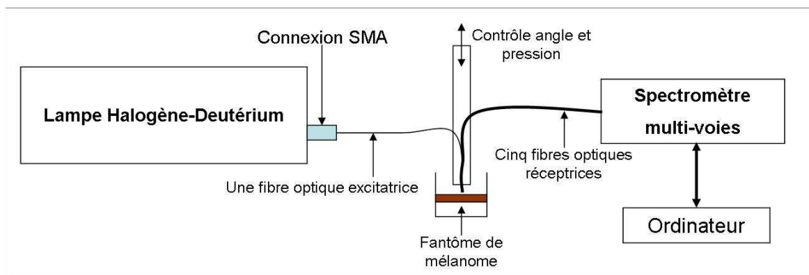
Figure 29 : Schéma bloc de l'instrumentation utilisée pour la spectroscopie de réflectance diffuse résolue spatialement pour la détermination non invasive de l'indice de Breslow du mélanome simulé par fantôme
