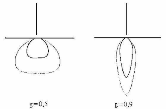
Figure 18 : Distribution angulaire de la diffusion en fonction de la valeur du paramètre d'anisotropie g .
