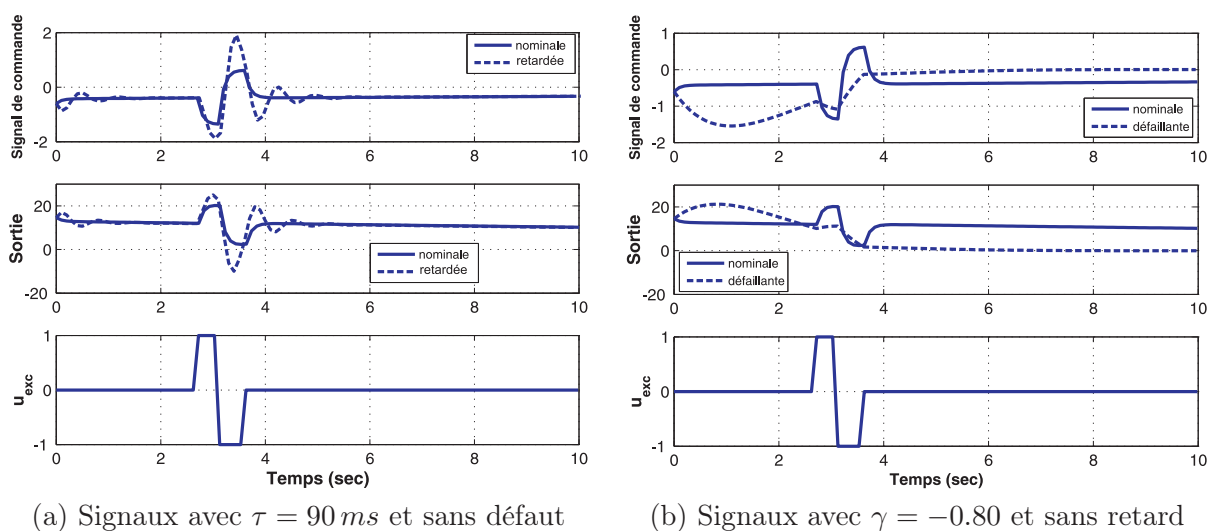
FIG. 2.12 – Réponse du système avec retard et défaut : effets séparés
