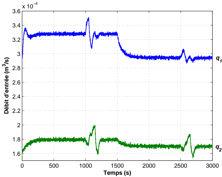
FIG. 4.10 – Signaux de commande : scénario 6 et changement de la référence pour calculer l'ISO
