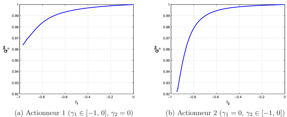
FIG. 4.3 – Indice basé sur la reconfigurabilité en BO pour chaque actionneur dont un sain
