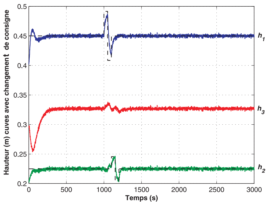
FIG. 4.8 – Signaux de sortie sans défaut avec changement de la référence pour calculer l'ISO
