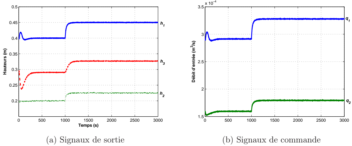
FIG. 4.5 – Réponse du système à une variation de la référence à [0.45, 0.225]^T à 1000 s
