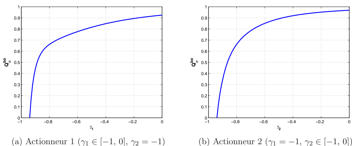
FIG. 4.2 – Indice basé sur la reconfigurabilité en BO pour chaque actionneur étant un perdu
