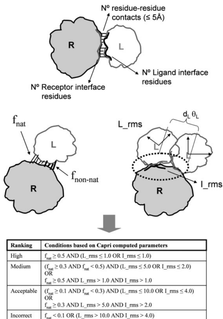
FIG. 1.14 – Illustrations du calcul des RMSD de l'interface et du ligand. L_{rmsd} : RMSD de l'interface ; L_{rmsd} : RMSD du ligand ; f_{nat} : fraction de contacts natifs ; f_{non-nat} : fraction de contacts non natifs. Tableau présentant le classement des modèles en fonction de L_{rmsd} , L_{rmsd} et f_{nat} . Reproduit de Méndez et al. (2005)
