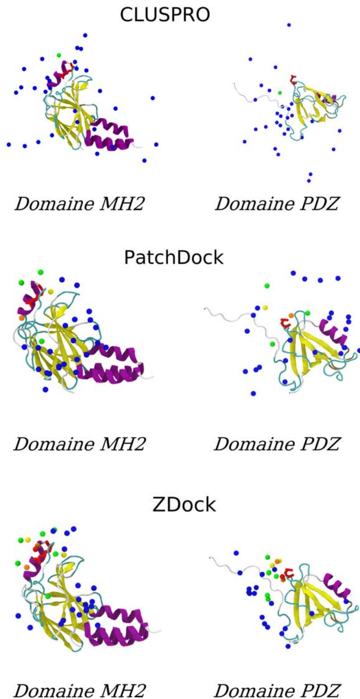
FIG. 2.20 – Graphique montrant la répartition du ligand par rapport au récepteur et inversement dans le cas où l'on donne R 279 en contact avec E 1321 comme information aux serveurs. Les sphères représentent les positions du résidu R 279 ou E 1321 pour chaque solution. Les sphères sont colorées en fonction de la distance R 279 -E 1321 : bleu pour une distance supérieure à 15 Å ; vert : pour une distance comprise entre 10 et 15 Å ; jaune : pour une distance comprise entre 7,5 et 10 Å ; orange : pour une distance comprise entre 5 et 7,5 Å et rouge : pour une distance inférieure à 5 Å. En rouge, le résidu R 279 au niveau de Smad3 et E 1321 au niveau d'Erbin.
