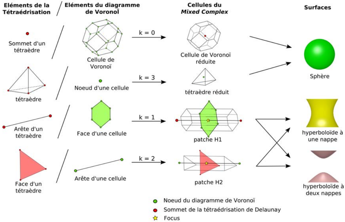
FIG. 3.8 – En mixant les éléments de la tétraédration de Delaunay et du diagramme de Voronoï, il est possible d'obtenir de nouvelles cellules : les cellules du Mixed Complex . Chaque type de cellule peut couper un morceau de surface, soit de sphère soit d'hyperboloïdes à une ou deux nappes.
