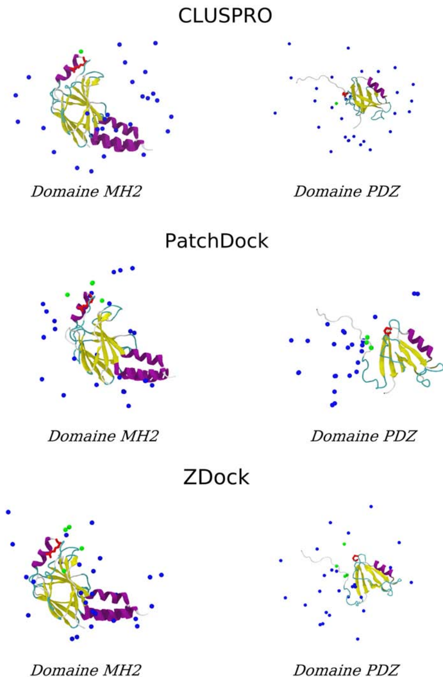
FIG. 2.19 – Graphique montrant la répartition du ligand par rapport au récepteur et inversement dans le cas où aucune information n'est donnée aux serveurs. Les sphères représentent les positions du résidu R 279 ou E 1321 pour chaque solution. Les sphères sont colorées en fonction de la distance R 279 -E 1321 : bleu pour une distance supérieure à 15 Å ; vert : pour une distance comprise entre 10 et 15 Å ; jaune : pour une distance comprise entre 7,5 et 10 Å ; orange : pour une distance comprise entre 5 et 7,5 Å et rouge : pour une distance inférieure à 5 Å. En rouge, le résidu R 279 au niveau de Smad3 et E 1321 au niveau d'Erbin.
