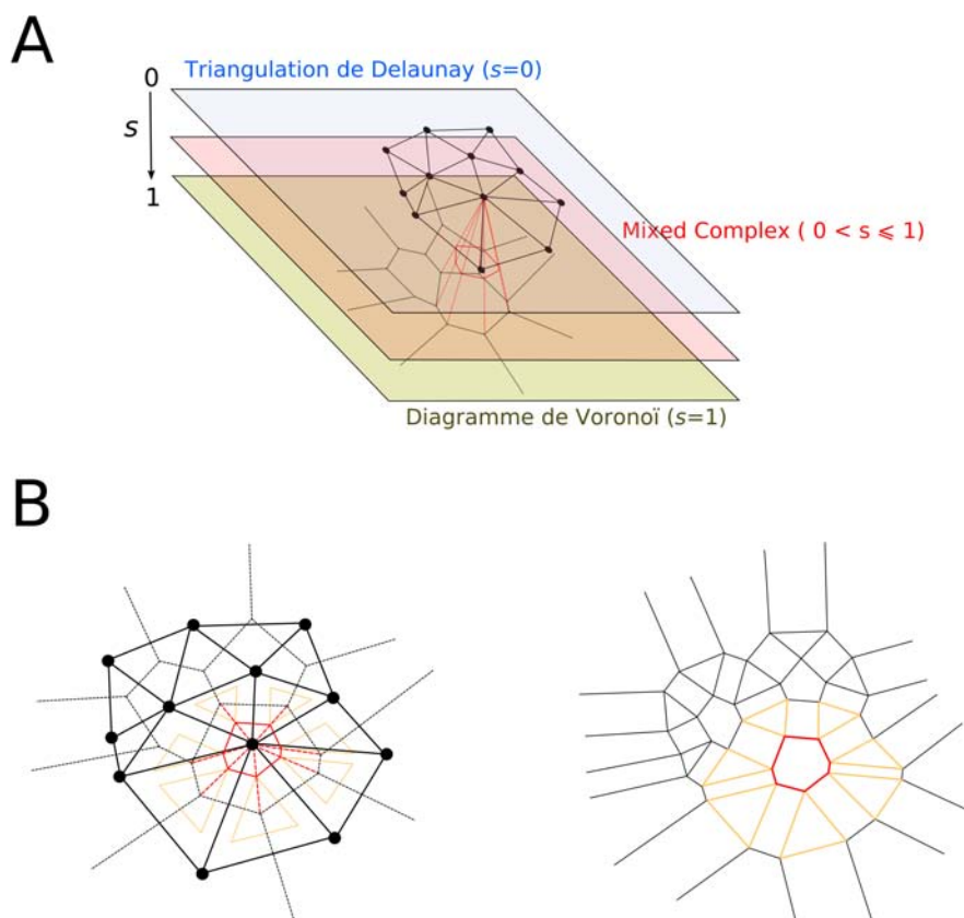
FIG. 3.7 – A- Création, en deux dimensions, d'une cellule du Mixed Complex à partir des cellules de Voronoï et de Delaunay associées : le sommet de la triangulation de Delaunay est relié aux noeuds du diagramme de Voronoï. La cellule du Mixed Complex est obtenue en faisant varier un plan, le plan du Mixed Complex , entre les plans de Voronoï et de Delaunay. B- Vue de dessus du résultat : en rouge, la cellule de Voronoï réduite résultant du mix entre une cellule de Voronoï et un sommet de Delaunay. En orange, les triangles réduits résultant du mix entre des triangles de Delaunay et des noeuds du diagramme de Voronoï.
