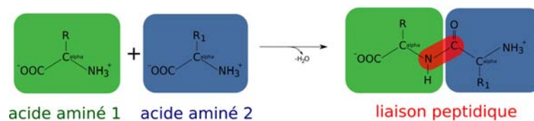
FIG. A.2 – Formation d’une liaison peptidique.
