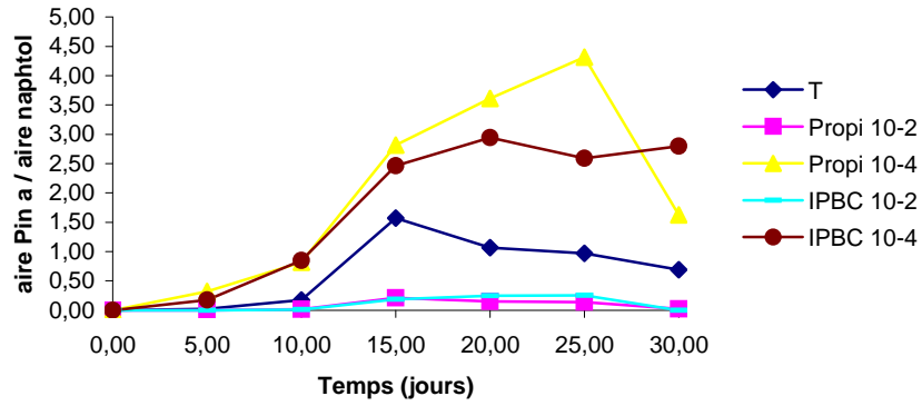
Figure 92: Evolution du facteur de réponse des composés: aire composé Pin a / aire naphhtol lors de la dégradation du bois de hêtre par P. placenta
