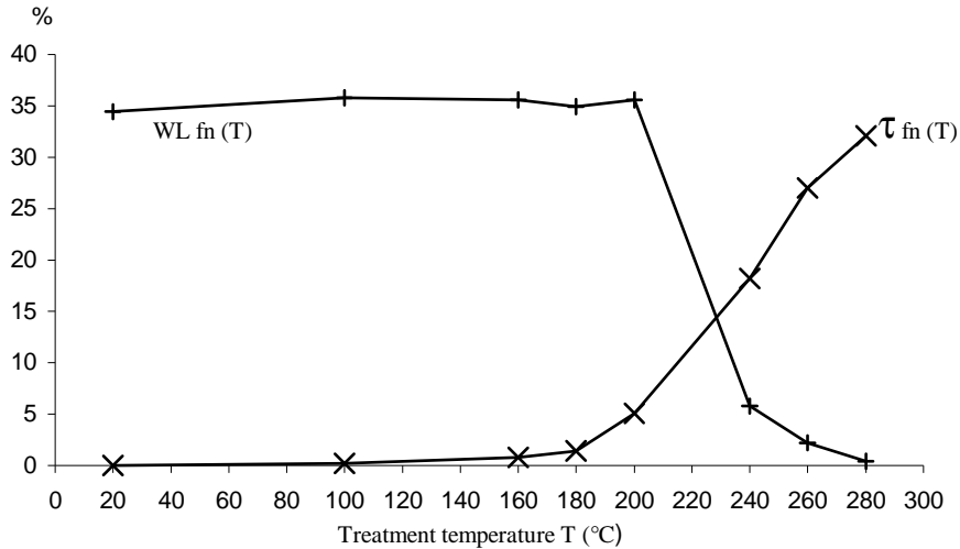
Figure 96. Corrélation entre les pertes de masse dues au traitement thermique ( \square ) et celles dues à l'action de Trametes versicolor (WL) (Hakkou, 2006)
