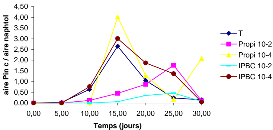
Figure 94: Evolution du facteur de réponse des composés: aire composé Pin c / aire naphhtol lors de la dégradation du bois de hêtre par P. placenta
