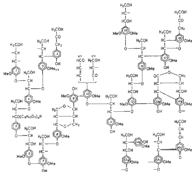
Figure 5 : Structure de la lignine proposée par ADLER (1977)
