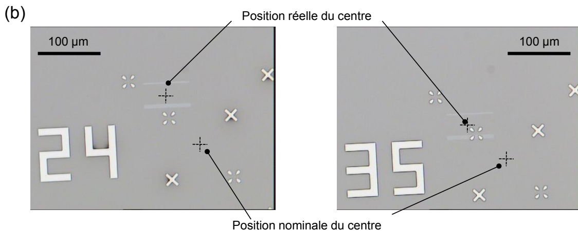
Figure 2.43c. a) Schéma du système de croix x. b) Images par microscopie optique montrant le décalage entre les positions réelles et nominales du writefield pour deux expositions différentes du même motif.
