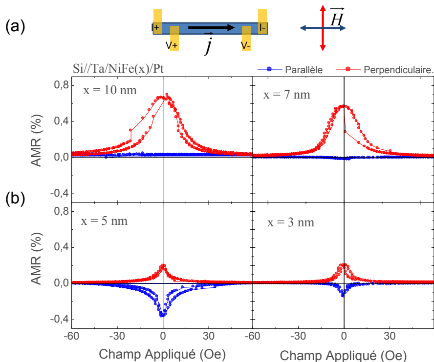
Cycles d'AMR obtenus pour les dispositifs ayant une composition Si//Ta/NiFe(x)/Pt, avec x = 3, 5, 7 et 10 nm. Pour de fins de comparaison, les courbes sont normalisées par rapport à la résistance en saturation.
