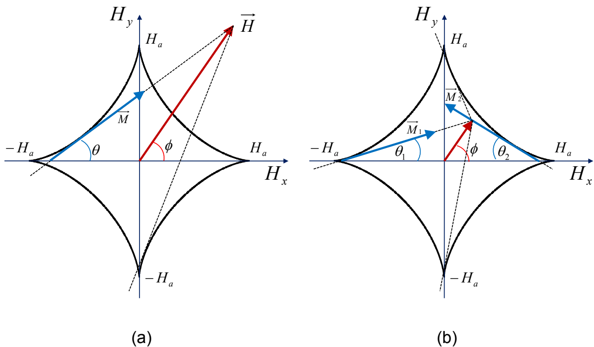
tangentes à l'astroïde de Stoner-Wohlfarth. a) Pour H > H_R il y a une seule position d'équilibre. b) Si H < H_R , deux positions d'équilibre sont possibles.
