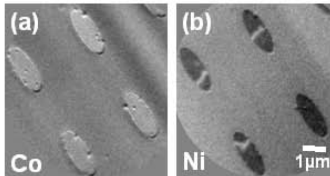
Fig. 5.4. Jonctions tunnel Co/Al 2 O 3 /NiFe sous forme d'ellipses. Image de microscopie de photo-électrons X obtenues au seuil d'absorption du Co (a) et au seuil d'absorption du Ni (b).
