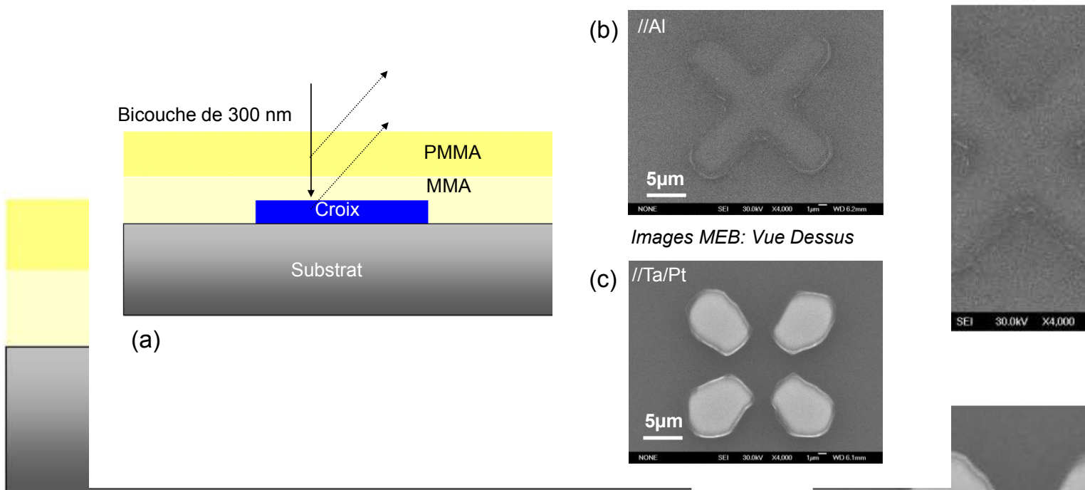
Fig. 2.42. a) Schéma illustrant l'observation des croix d'alignement à travers une bicouche de résine. b) Contraste obtenu pour des croix réalisées en Al. c) Contraste obtenu pour des croix réalisées en Ta/Pt.
