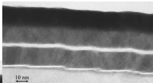
Fig. 5.1. Cliché de microscopie électronique en section transverse pour une jonction tunnel \text{Co}/\text{Al}_2\text{O}_3/\text{FeNi}/\text{Au} déposée sur un substrat à topologie modulée. La modulation du substrat de Si se transmet dans la couche de FeNi [2].
