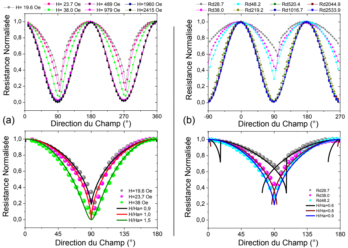
simulations. a) un dispositif ne pas ayant de modulation. b) dispositif à géométrie longitudinale de période 300 nm.
