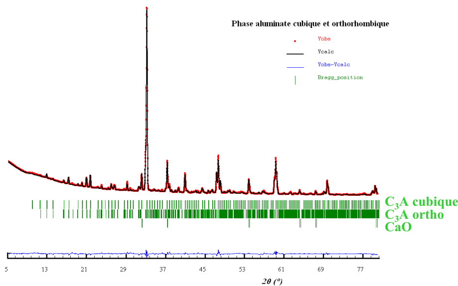
Figure 107 : Diffractogrammes mesurés et calculés de la phase aluminatée cubique et orthorhombique.
