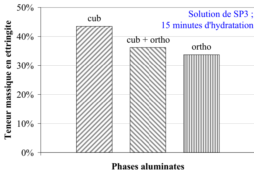
Figure 110 : Teneur massique en ettringite dans la phase solide en fonction de la variété de la phase aluminatée après 15 minutes d'hydratation dans une solution de superplastifiant SP3.
