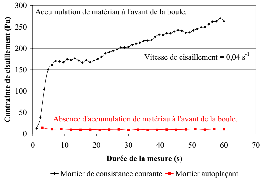
Figure 45 : Influence de la consistance du mortier sur l'évolution de la contrainte de cisaillement à vitesse de cisaillement constante au cours du déplacement du S.M.B.
