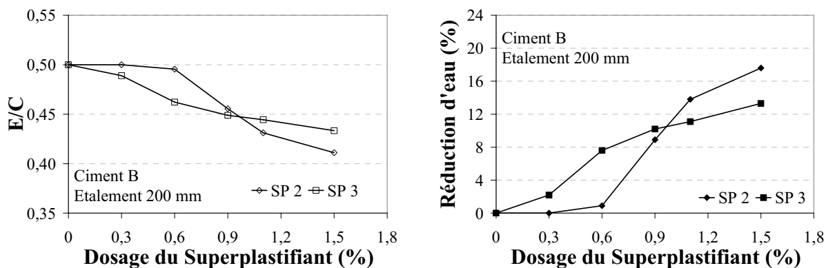
Figure 72 : Évolution du rapport E/C (gauche) et de la réduction de la teneur en eau (droite) avec le dosage en superplastifiants SP2 et SP3 dans des mortiers de ciment B de consistance courante.
