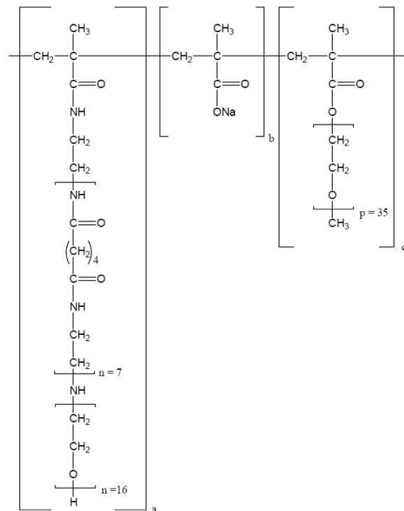
Figure 20 : Structure chimique d'un polycarboxylate de troisième génération [96].
