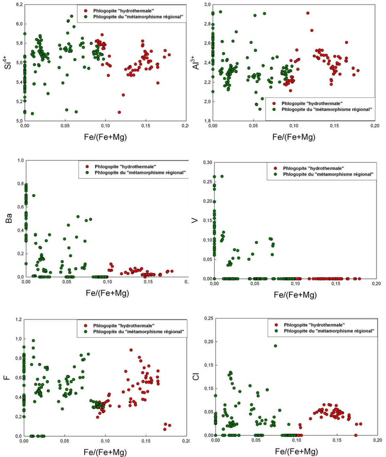
Figure I-84 : Variations des majeurs et des éléments mineurs en (pfu) en fonction du rapport Fe/(Fe+Mg) pour les phlogopites du district de Cage.
