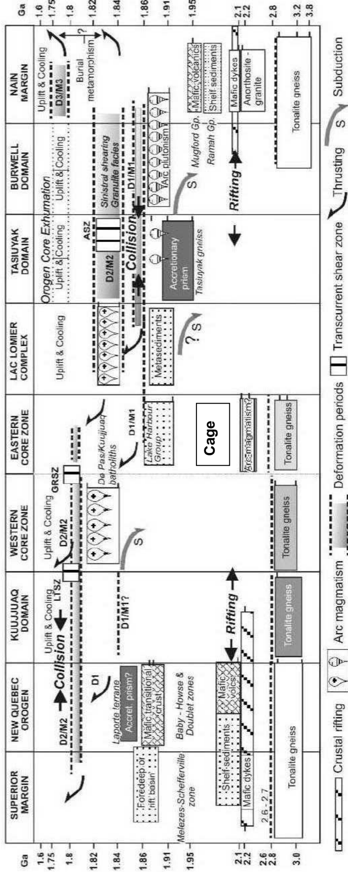
Figure 1-4 : Chronologie des événements dans la province du Churchill basée sur différentes datations U/Pb. L'épaisseur des boîtes indique la précision de la datation. ASZ, Abloviak shear zone; GRSZ, George River shear zone; LTSZ, Lac Tudor shear zone (d'après Wardle et al., 2002).
