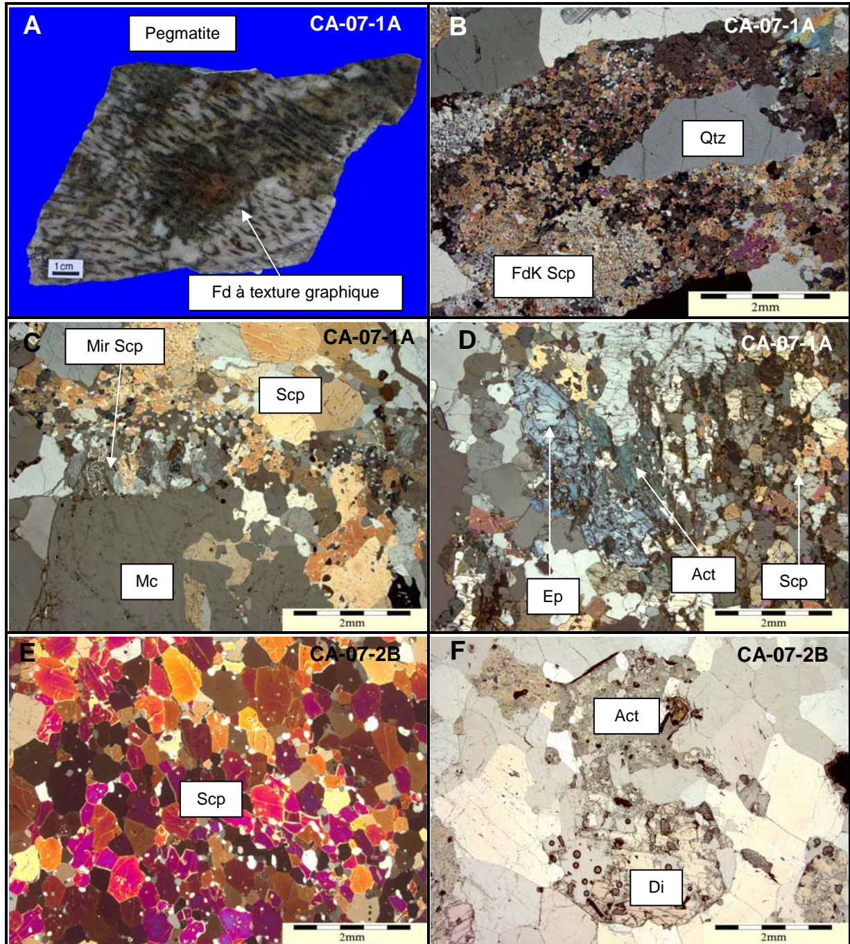
Figure I-79 : A. Pegmatite A à feldspath scapolitisé à texture graphique d'épaisseur au contact avec une pegmatite. B. LPA. Feldspath à texture graphique remplacé par de la scapolite finement cristallisée associé à du quartz (Qtz). C. LPA. Reliques de myrmékites scapolitisées (Mir Scp) au contact avec un cristal de microcline (Mc) partiellement scapolitisé. D. LPA. Cristal sub-automorphe d'épidote zonée associé à de l'actinolite (Act). E. LPA. Scapolite (Sca) à texture granoblastique. F. LN. Scapolite (Sca) à inclusions de diopside (Di) et d'actinolite (Act).
