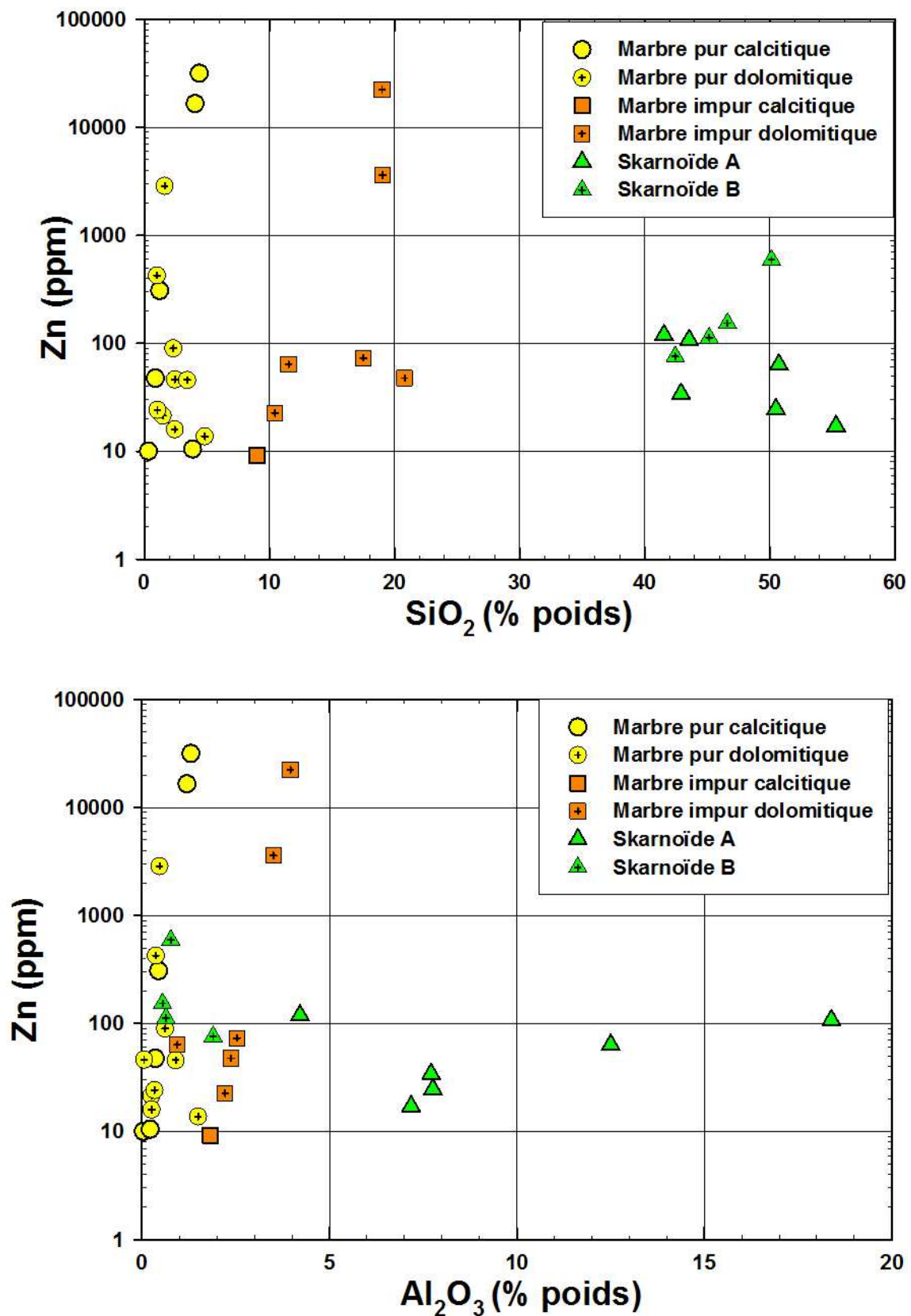
Figure II- 23 : Diagramme Zn (ppm) en fonction de SiO 2 et Al 2 O 3 (% poids).
