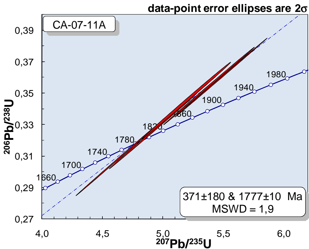
Figure I-59 : Datation U/Pb sur zircons des pegmatites B.
