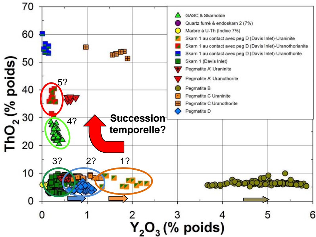
Figure III- 10 : Diagramme \text{ThO}_2 en fonction d' \text{Y}_2\text{O}_3 pour les minéraux d'uranium des skarns et des pegmatites.
