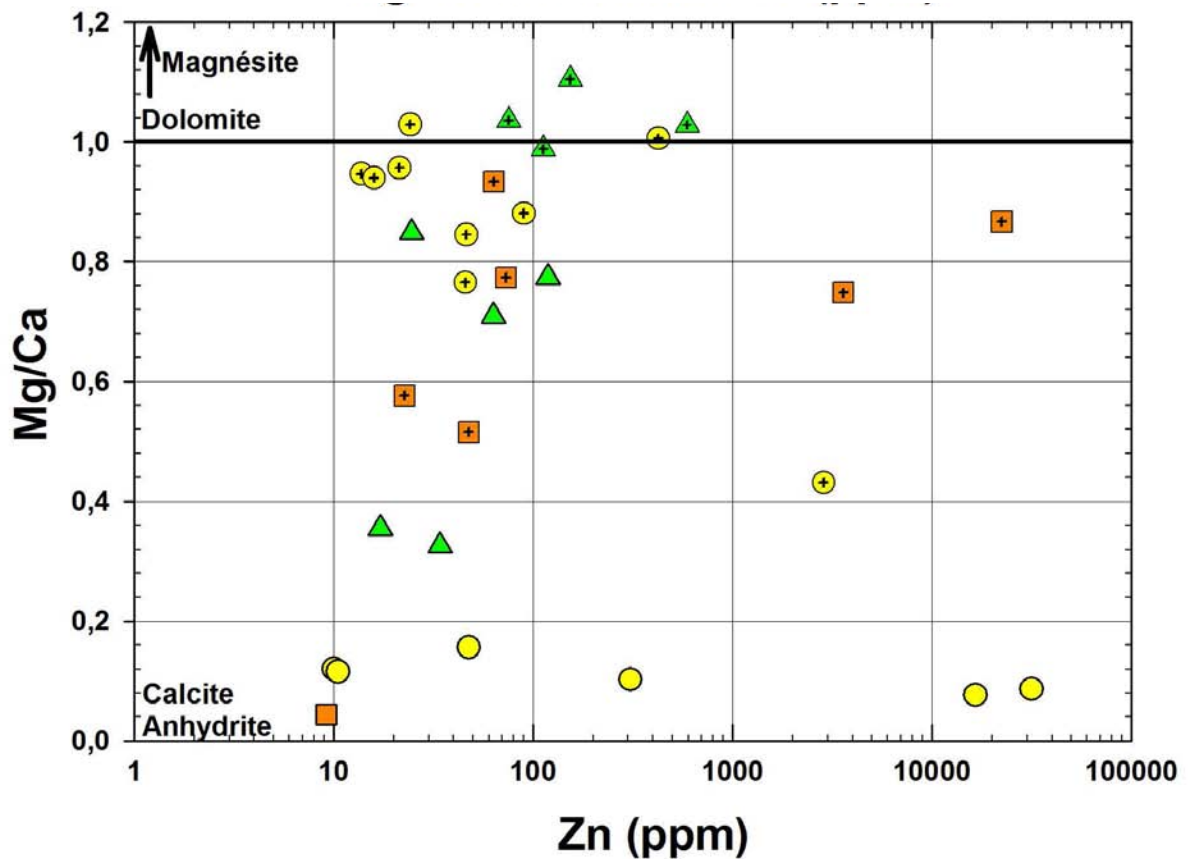
Figure II- 24 : Diagramme Mg/Ca (cationique) en fonction de la teneur en Zn (ppm).
