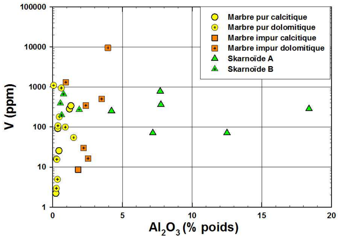
Figure II- 25 : Diagramme V (ppm) en fonction de \text{SiO}_2 et \text{Al}_2\text{O}_3 (% poids).
