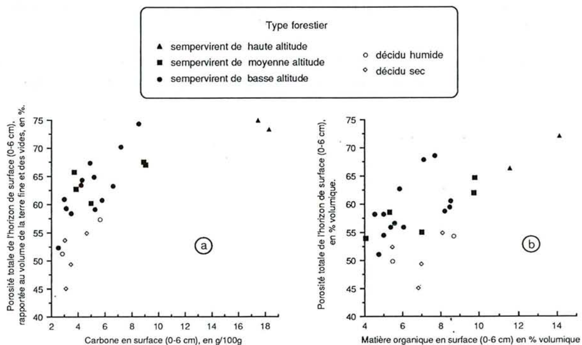
Figure 2-11. Porosité totale de l'horizon de surface rapportée (a) au volume de la terre fine et des vides, (b) au volume total, en fonction de la teneur en matière organique (a) pondérale, (b) volumique.
