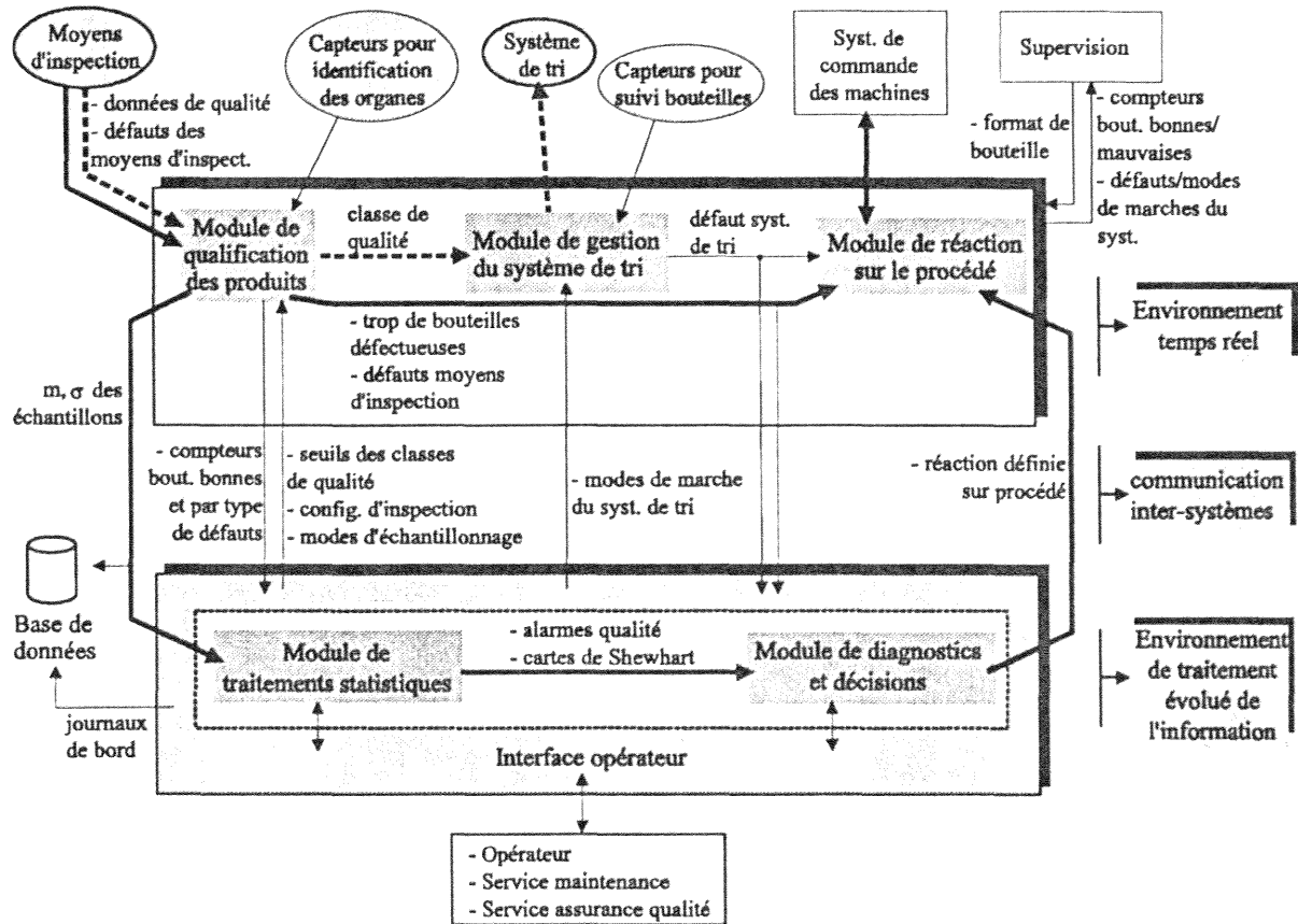
Figure III.16 : Architecture fonctionnelle d'un système de maîtrise de la qualité d'un procédé d'embouteillage
