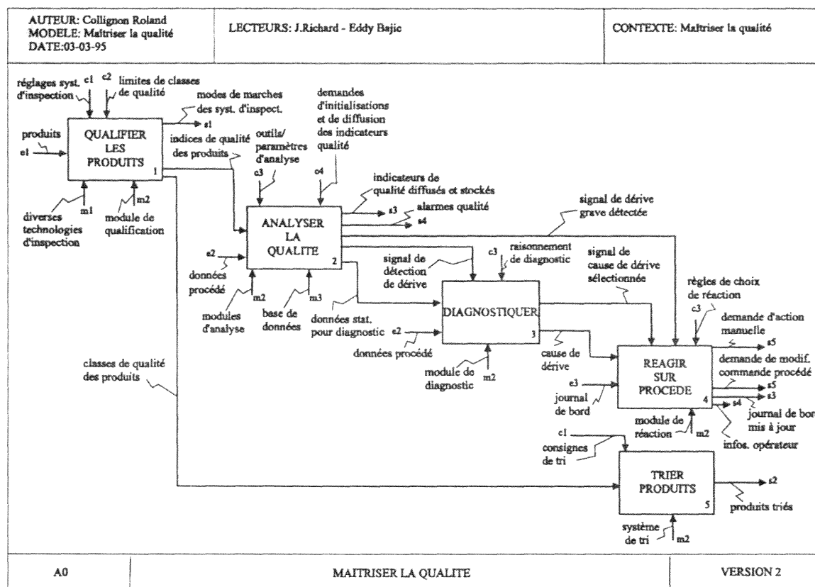
Figure III.2 : Diagramme SADT de l'activité « Maîtriser la qualité »
