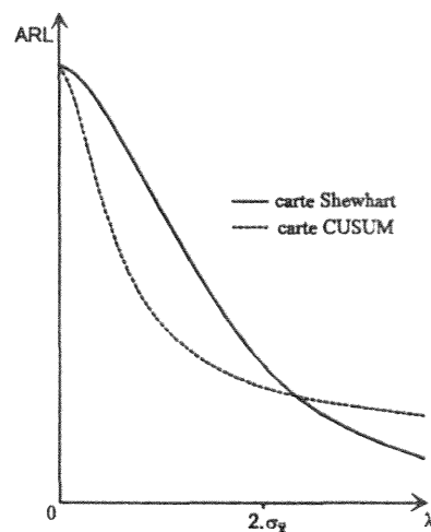
Figure II.13 : Exemple de courbes de comparaison d'efficacité des cartes Shewhart et CUSUM
