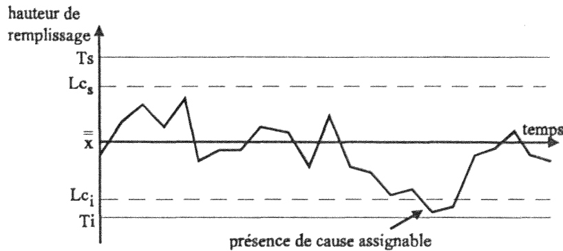
Figure II.5 : Exemple de carte de contrôle de Shewhart
