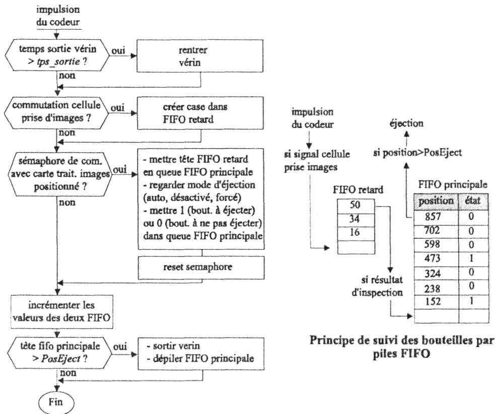
Figure IV.8 : Algorithme de suivi des bouteilles
