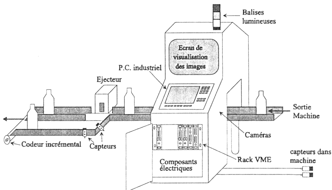
Figure IV.2 : Intégration du système dans la ligne de production
