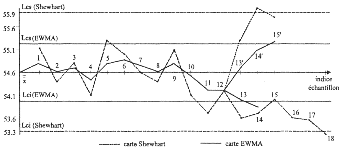
Figure II.23 : Carte de contrôle EWMA
