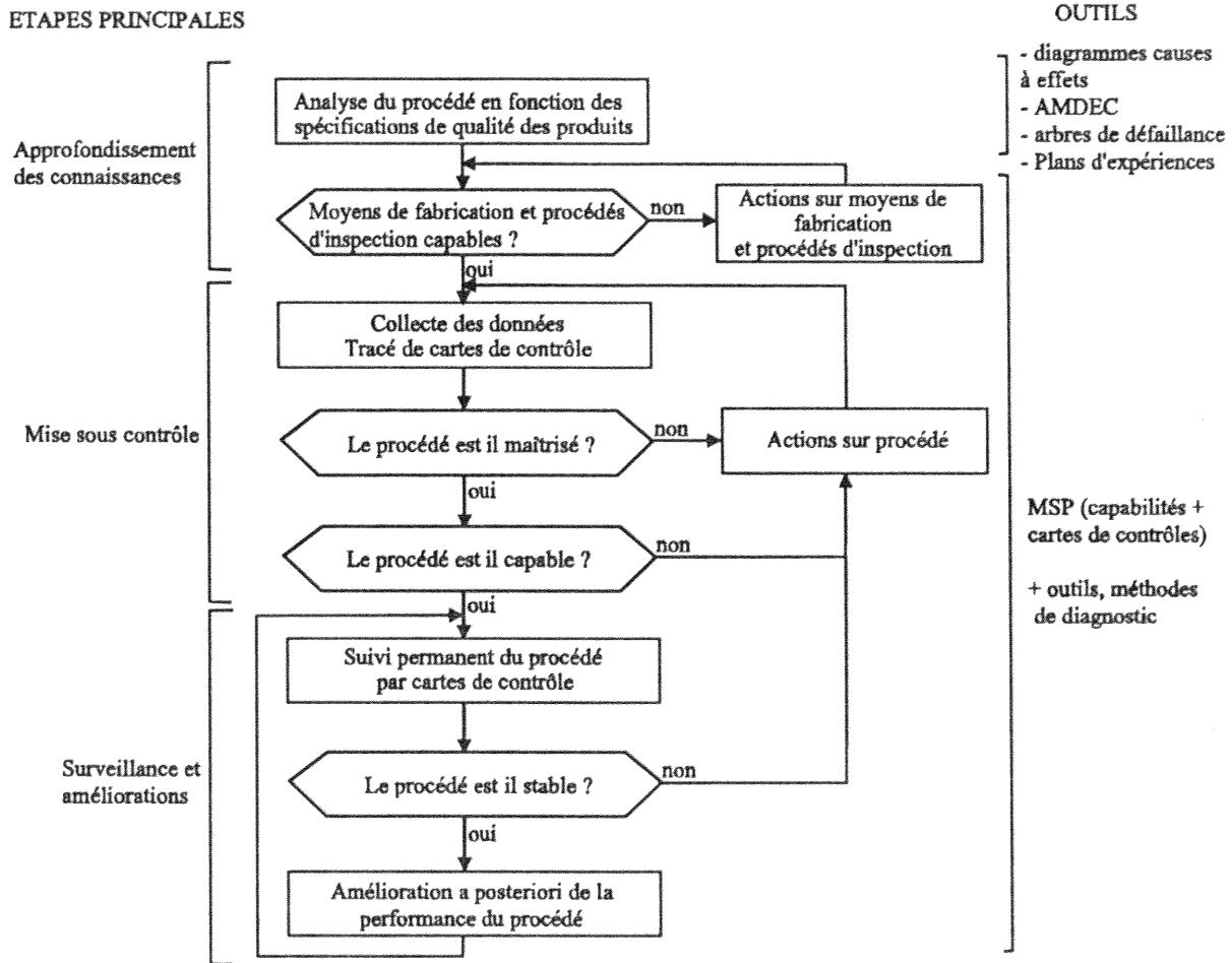
Figure II.3 : La démarche de maîtrise du procédé de fabrication
