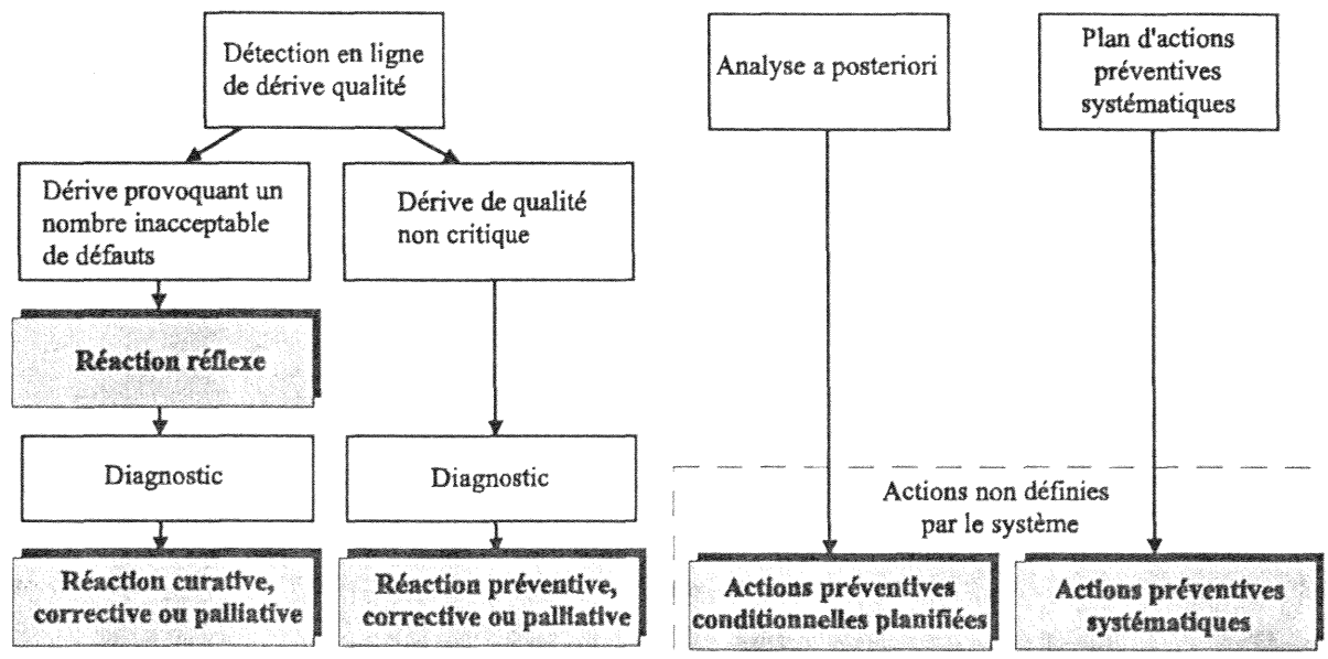
Figure III.10 : Les différents types d'actions sur le procédé
