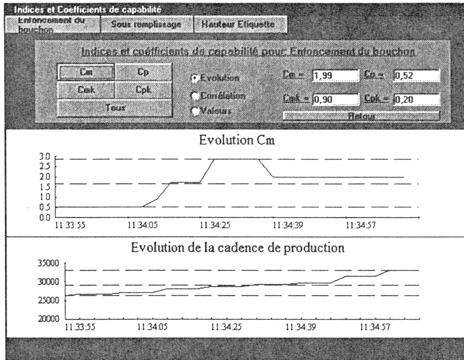
Figure IV.16 : Exemple d'écran de présentation des indices de capacité
