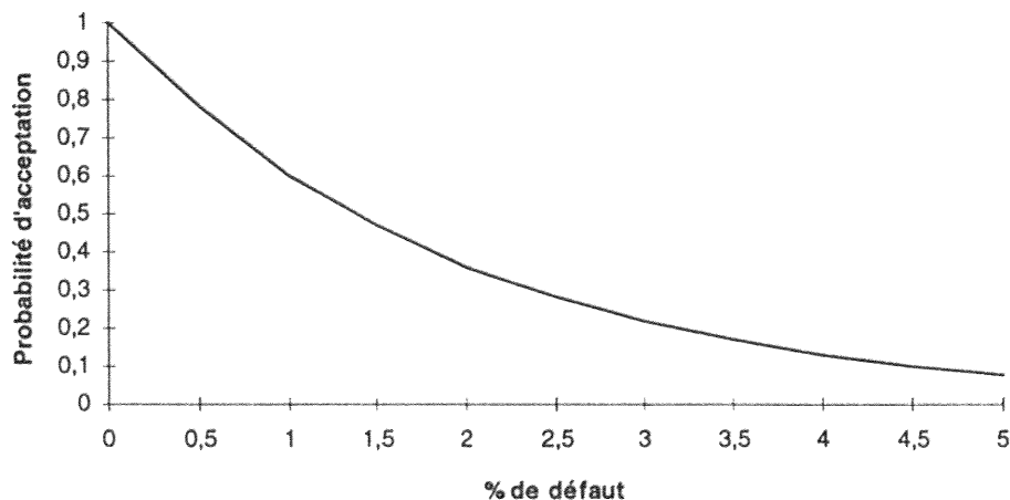
Figure I.4 : Exemple de courbe d'efficacité d'un plan de contrôle de réception
