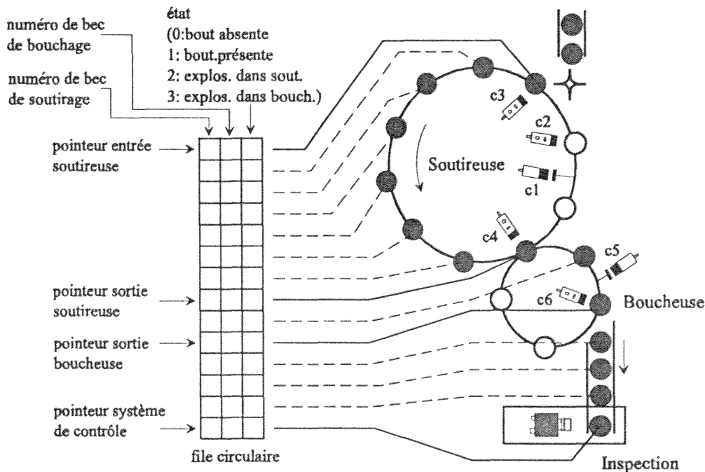
Figure IV.9 : Principe d'identification des organes
