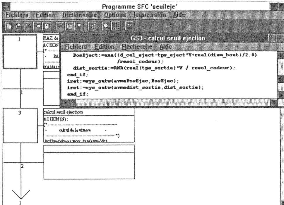
Figure IV.11 : Le Grafcet "SeuilEje" de calcul des paramètres de l'éjection
