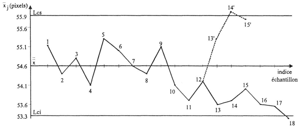
Figure II.21 : Carte de contrôle de Shewhart
