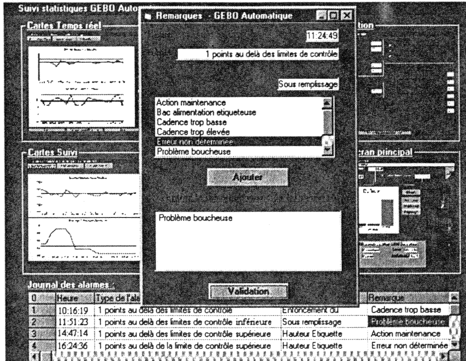
Figure IV.15 : Exemple de journal des alarmes et de saisie de cause assignable
