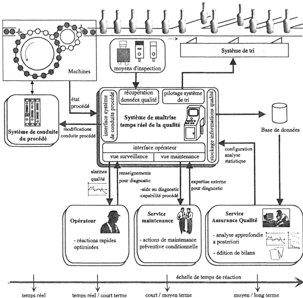
Figure III.11 : Interactions du système avec son environnement
