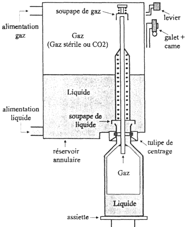
Figure I.12 : L'étape de remplissage réalisée par un organe de souflage
