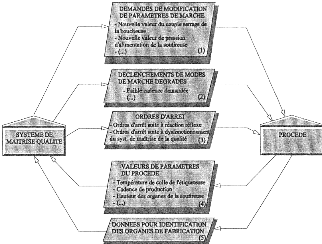
Figure III.13 : Modèle de communication entre le système et le procédé
