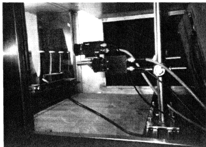
Figure IV.20 : Photo de l'implantation des caméras
