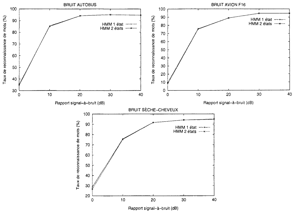
FIG. 9.2 - Influence du nombre d'états du HMM de bruit sur le taux de reconnaissance de 206 mots isolés.
