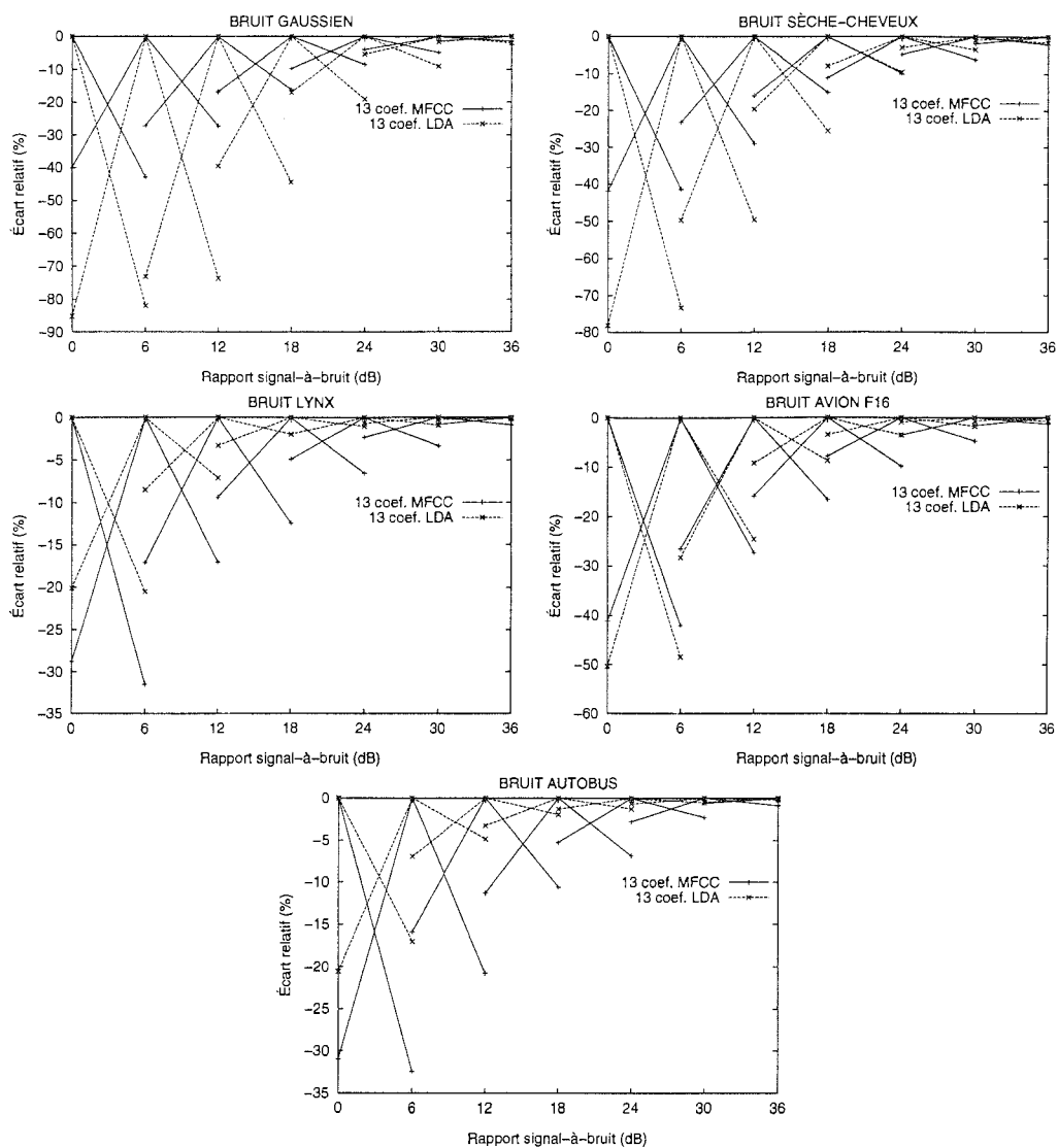
FIG. 10.3 - Robustesse relative des paramétrage LDA / MFCC aux variations du rapport signal-à-bruit SNR_{test} et SNR_{ref} . Écart relatif des taux d'évaluation phonétique par rapport à la configuration où SNR_{ref} = SNR_{test} . Moyenne sur tous les locuteurs.
