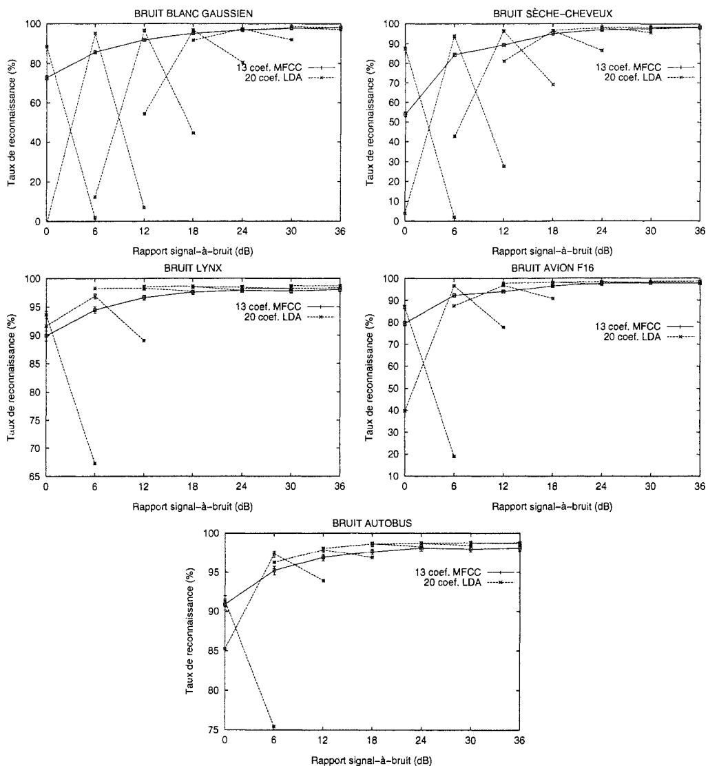
FIG. 10.4 - Robustesse du prétraitement par LDA aux variations du rapport signal-à-bruit entre le corpus utilisé pour déterminer la matrice de projection LDA et le corpus de test. Moyenne sur tous les locuteurs.
