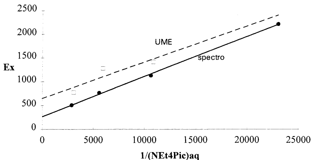
Fig.86 : Détermination graphique de la constante d'extraction E et de la constante de dissociation de \text{Et}_4\text{NPic} avec une UME de Pt et par spectrophotométrie.
