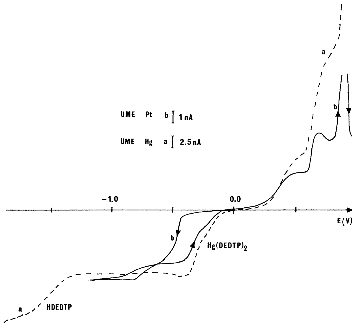
Fig.101 : Extraction de \text{Hg}(\text{NO}_3)_2 4 \cdot 10^{-4} M en milieu aqueux 7M par HDEDTP 1,5 \cdot 10^{-3} M. Analyse phase organique, ECS pont éthanol 50 \text{mV} \cdot \text{s}^{-1} , \text{N}_2 pdt 15 mn, \text{Hg}(\text{DETDP})_2 4 \cdot 10^{-4} M (si quantitatif), (a) UME Hg/Pt, (b) UME Pt
