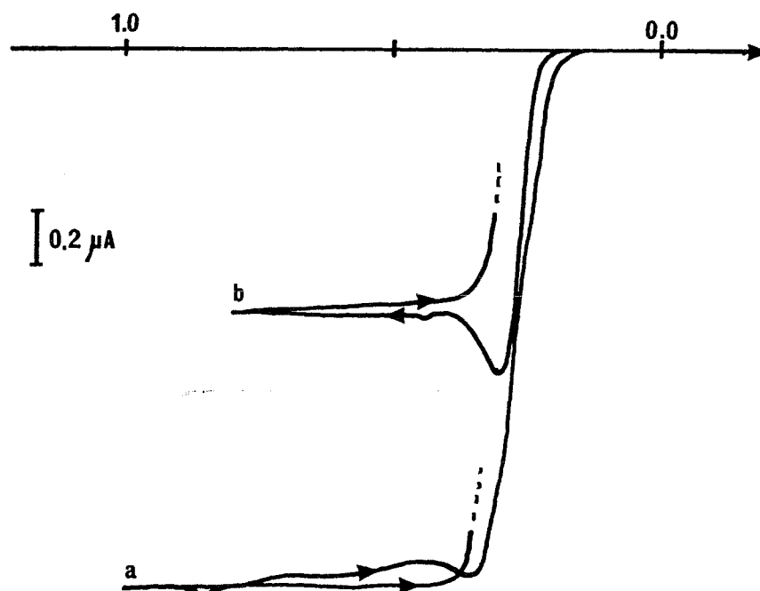
Fig.38 : tracé voltampérométrique de la réduction du \text{CuSO}_4 10^{-3} M dans \text{H}_2\text{O} à une électrode à goutte de mercure stationnaire, réf. ECS, 2 \text{ mV}\cdot\text{s}^{-1} , (a) sans électrolyte, (b) avec \text{NaClO}_4 10^{-1} M
