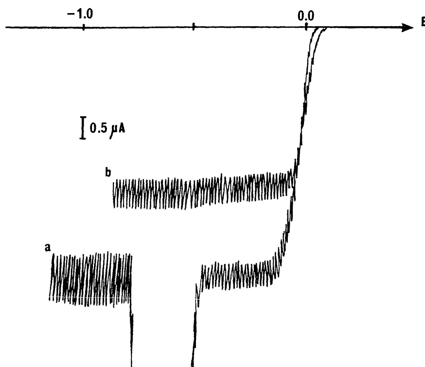
Fig.39 : tracé voltampérométrique de la réduction du \text{CuSO}_4 10^{-3} M dans \text{H}_2\text{O} à une électrode à goutte de mercure tombante, réf. ECS, 2 \text{ mV}\cdot\text{s}^{-1} , (a) sans électrolyte, (b) avec \text{NaClO}_4 10^{-1} M,
