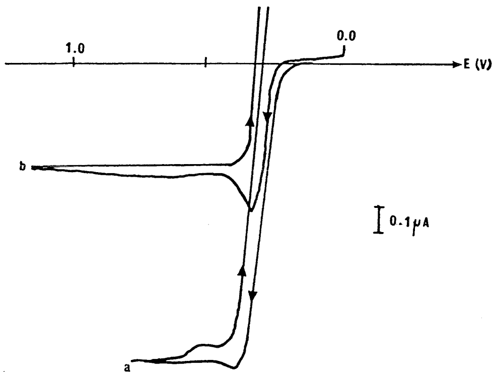
Fig.43 : courbes i-E de la réduction du \text{CuClO}_4 2 \cdot 10^{-3} M dans \text{CH}_3\text{CN} 50%, Hg goutte stationnaire, réf. ECS, (a) sans électrolyte, (b) avec \text{NaClO}_4 10^{-1} M
