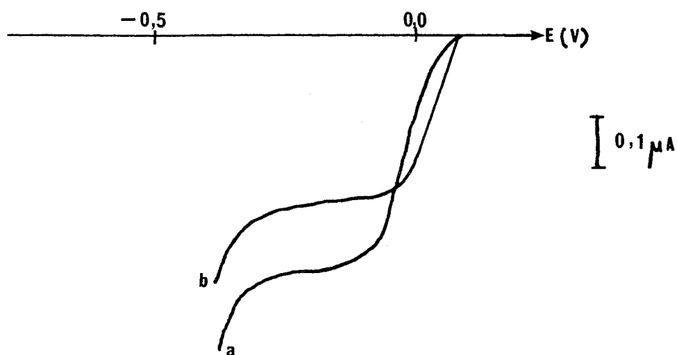
Fig. 35 : tracé voltampérométrique de la première vague de réduction du \text{Cu}(\text{ClO}_4)_2 5 \cdot 10^{-4} M dans le \text{CH}_3\text{CN} 2% à une électrode à goutte de Hg stationnaire, réf. ECS, 5 \text{ mV} \cdot \text{s}^{-1} , (a) sans électrolyte, (b) avec \text{NaClO}_4 0,1M
