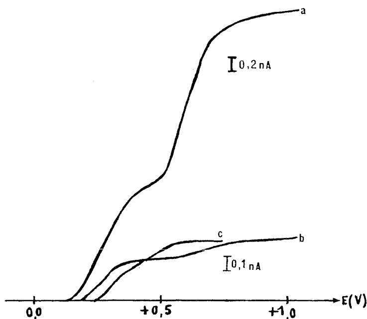
Fig.87 : Réaction d'échange \text{I}^- / \text{ClO}_4^- , UME Pt, 10 \text{ mV} \cdot \text{s}^{-1} , réf. ECS pont éthanol, (a) \text{Hex}_4\text{NI} 5,4 \cdot 10^{-4} \text{ M} , (b) après la réaction d'échange avec \text{KClO}_4 5,5 \cdot 10^{-4} \text{ M} , (c) = (b) + \text{Hex}_4\text{NClO}_4 4,5 \cdot 10^{-4} \text{ M}
