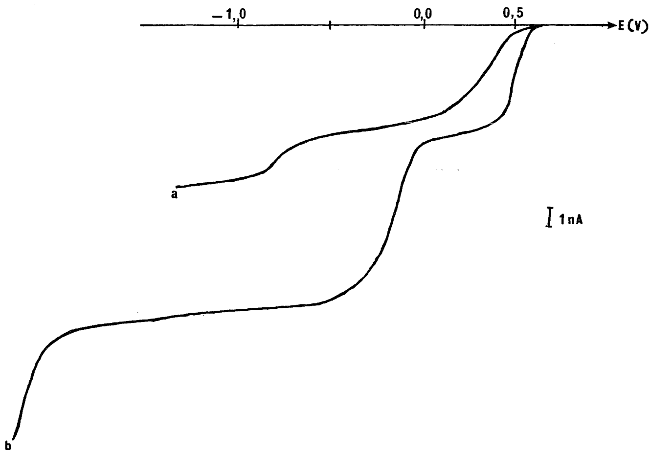
Fig.64 : Réduction de l'iode en présence d'électrolyte support dans \text{CH}_2\text{Cl}_2 sat. \text{H}_2\text{O} , UME Pt, 20 \text{ mV}\cdot\text{s}^{-1} , \text{I}_2 1,9 \cdot 10^{-4} \text{ M} , (a) en absence d'électrolyte, (b) avec \text{NBU}_4\text{ClO}_4 5,2 \cdot 10^{-4} \text{ M}
