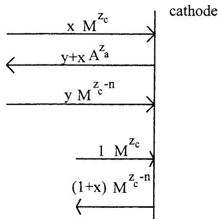
Fig.15 : Modélisation de la réduction d'un cation
