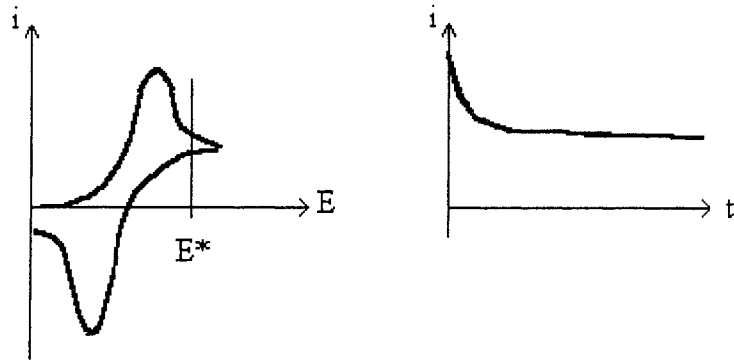
Fig.7 : Représentation des courbes théoriques i = f(E) et i = f(t) à E^* pour un régime de diffusion sphérique
