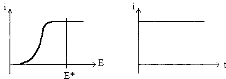
Fig.5 : Représentation des courbes théoriques pour un régime de diffusion plane stationnaire
