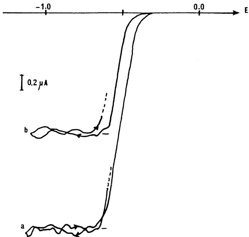
Fig.44 : courbes i-E de la réduction du \text{Cu}_2\text{SO}_4 10^{-3} M dans \text{CH}_3\text{CN} 50%, Hg goutte stationnaire, réf. ECS, (a) sans électrolyte, (b) avec \text{NaClO}_4 10^{-1} M
