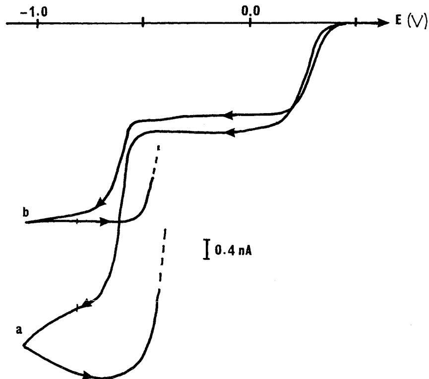
Fig.46 : Réduction du \text{CuSO}_4 10^{-3} M dans \text{CH}_3\text{CN} 50%, UME Pt, réf. ECS, 50 \text{ mV}\cdot\text{s}^{-1} , (a) sans électrolyte, (b) avec \text{NaClO}_4 10^{-1} M
