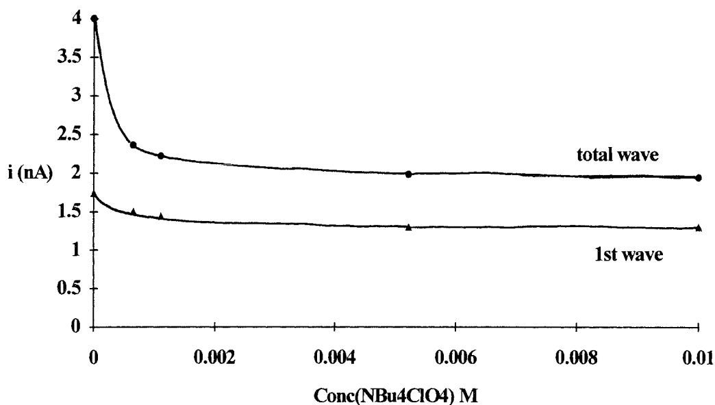
Fig.61 : Evolution des courants limites de la 1 ère à E = +0,35 V/ECS et de la 2 ème vague à E = +0,85 V/ECS de l'oxydation de \text{NBu}_4\text{I} 5, 3 \cdot 10^{-4} M en fonction de la quantité d'électrolyte [\text{NBu}_4\text{ClO}_4] ajouté.
