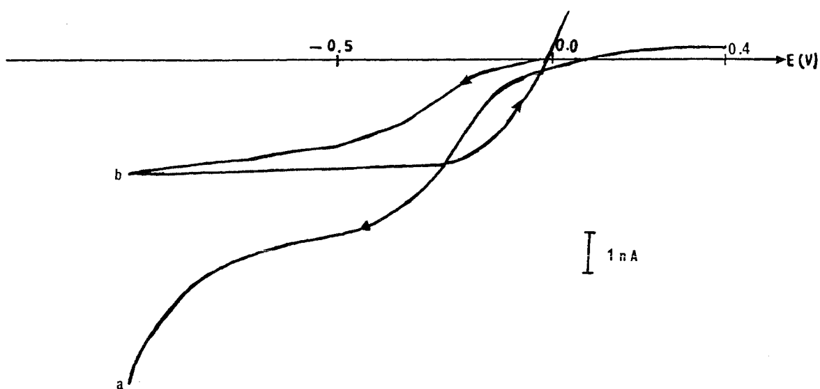
Fig.37 : tracé voltampérométrique de la réduction \text{Cu}(\text{ClO}_4)_2 10^{-3} \text{ M} dans \text{H}_2\text{O} , à une UME Pt, réf. ECS, 50 \text{ mV} \cdot \text{s}^{-1} , (a) sans électrolyte, (b) avec \text{NaClO}_4 10^{-1} \text{ M}
