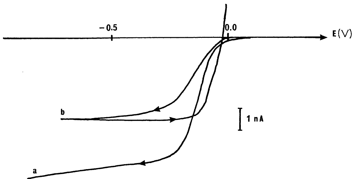
Fig.36 : tracé voltampérométrique de la réduction du \text{CuSO}_4 10^{-3} \text{ M} dans \text{H}_2\text{O} à une UME de Pt, réf. ECS, 50 \text{ mV} \cdot \text{s}^{-1} , (a) sans électrolyte, (b) avec \text{NaClO}_4 10^{-1} \text{ M}
