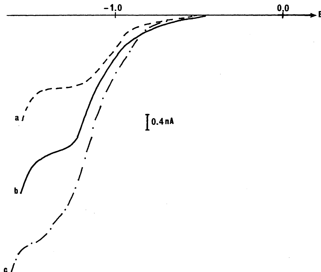
Fig.90 : Extraction de HCl par la TOA dans \text{CH}_2\text{Cl}_2 : analyse de la phase organique par UME de Pt : partie cathodique, Réf. ECS pont éthanol, 5 \text{ mV}\cdot\text{s}^{-1} , \text{N}_2 15 mn, la phase org. est diluée 83 fois (0,3 ml dans 25 ml) pour tracer le voltampérogramme, \text{Bu}_4\text{NClO}_4 10^{-2} \text{ M} , (\text{HCl})_{\text{aq}} 0,48 \text{ M} et (\text{TOA})_{\text{org}} (a) 4,3 \cdot 10^{-2} \text{ M} , (b) 7,8 \cdot 10^{-2} \text{ M} , (c) 0,13 \text{ M}
