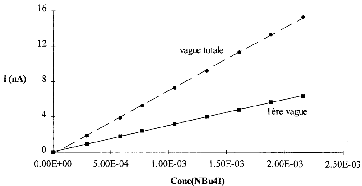
Fig.58 : Relation linéaire i_{lim} = kC pour NBu_4I dans CH_2Cl_2 sat. H_2O en absence d'électrolyte support; (—) 1 ère vague à +0,35 V/ECS, (---) vague totale à +0,85V /ECS
