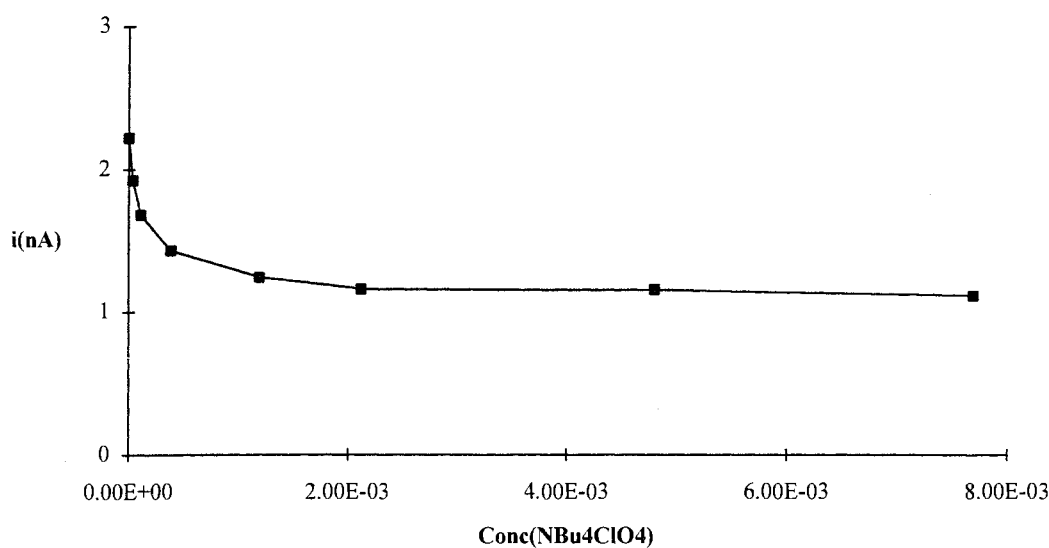
Fig.73 : Variation du courant limite (à E = +1,80 V par rapport à l'ECS) d'une solution de \text{Bu}_4\text{NPic} 2,6 \cdot 10^{-4} M, lors d'ajouts successifs de \text{Bu}_4\text{NClO}_4
