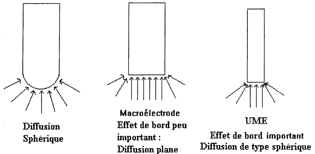
Fig.3 : Mode de diffusion sur différentes électrodes.
