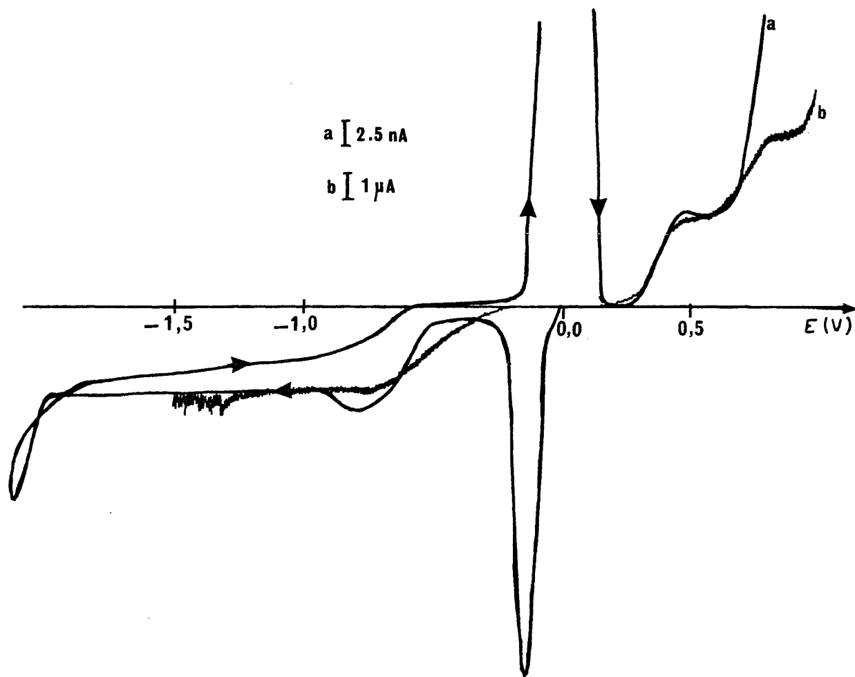
Fig.105 : Manip.2 : Extraction de \text{Pb}(\text{NO}_3)_2 3, 2 \cdot 10^{-4} M par une solution de HDEDTP 9, 9 \cdot 10^{-4} M dans \text{CH}_2\text{Cl}_2 , tracé avec une élec.Hg tombante ( 2 \text{ mV} \cdot \text{s}^{-1} ) et une UME de Hg ( 50 \text{ mV} \cdot \text{s}^{-1} ) ds la phase organique en présence de \text{Bu}_4\text{NClO}_4 1, 2 \cdot 10^{-2} M, Réf. ECS pont éthanol, \text{N}_2 15 mn
