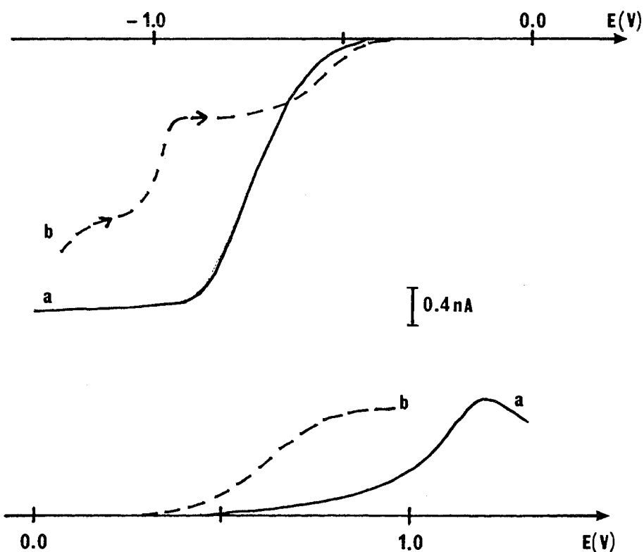
Fig.94 : Tracés cathodiques anodiques de l'addition de TOA sur une solution de HDEDTP dans CH_2Cl_2 sat. H_2O , UME Pt, N_2 après chaque ajout, 20\text{ mV}\cdot\text{s}^{-1} , Réf. ECS pont éthanol, Bu_4NClO_4 10^{-2} M, (a) HDEDTP 5\cdot 10^{-4} M, (b) HDEDTP 5\cdot 10^{-4} M + TOA 3,4\cdot 10^{-4} M
