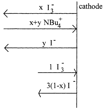
Fig.53 : Modélisation de la réduction des ions I_3^-
