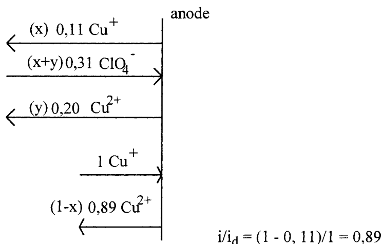
Fig.30 : Modélisation de l'oxydation du \text{Cu}^{\text{I}} milieu \text{ClO}_4^- , x = 0,11 et y = 0,20 dans \text{CH}_3\text{CN} 50%
