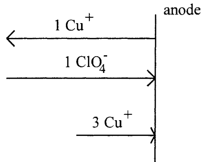
Fig.10 : Modélisation de B. Benzakour pour l'oxydation de \text{Cu}^+ en \text{Cu}^{2+} avec \text{ClO}_4^- comme contre-ion
