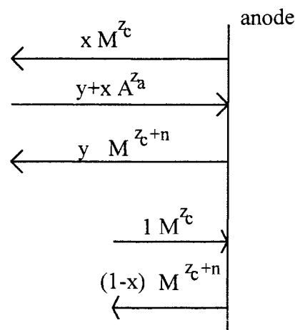
Fig.13 : Modélisation de l'oxydation de \text{M}^{z_c}
