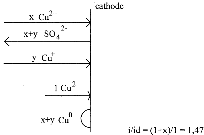
Fig.48 : modélisation de la réduction du \text{Cu}^{2+} dans \text{CH}_3\text{CN} 50%, si l'on prend en compte la migration de l'espèce formée à l'étape intermédiaire
