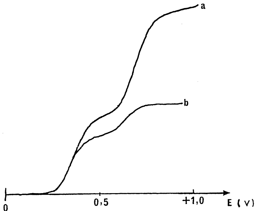
Fig.56 : Tracés voltampérométriques de Bu 4 NI 5,3.10 -4 M dans CH 2 Cl 2 sat. H 2 O (a) en absence d'électrolyte, (b) avec NBu 4 ClO 4 0, 01 M, UME Pt, 20 mV.s -1
