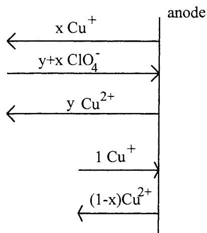
Fig.12 : Modélisation de l'oxydation du \text{CuClO}_4
