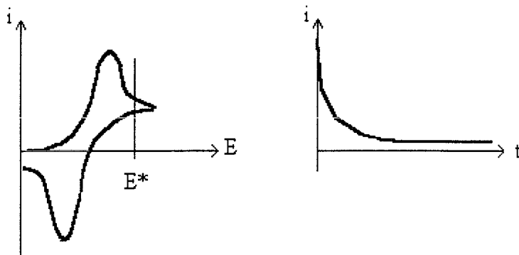
Fig.6 : Représentation des courbes théoriques i = f(E) et i = f(t) à E^* , pour un régime de diffusion plane transitoire
