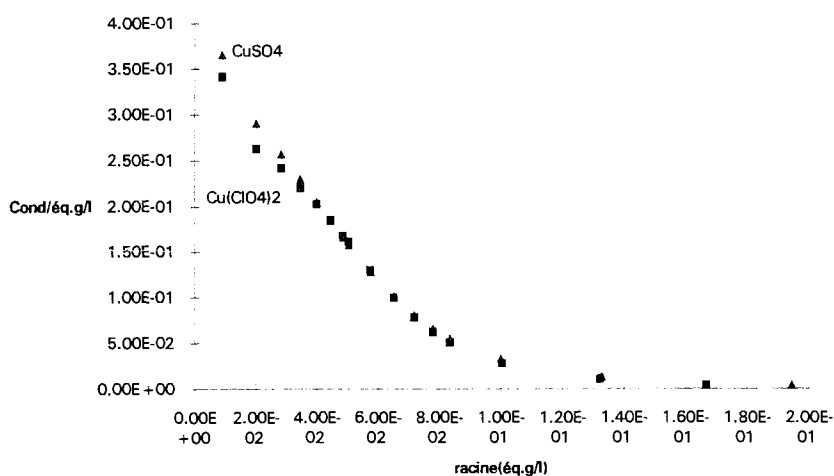
Fig.26 : Conductivité équivalente de \text{Cu}^{\text{II}} dans \text{H}_2\text{O}
