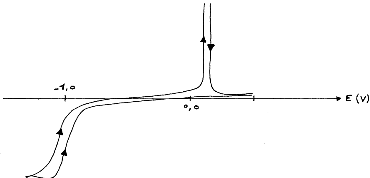
Fig.103 : Manip.1 : Extraction de \text{Pb}(\text{NO}_3)_2 3, 2 \cdot 10^{-4} M par une solution de HDEDTP 9, 7 \cdot 10^{-4} M dans \text{CH}_2\text{Cl}_2 , tracé avec UME Pt ds la phase organique en présence de \text{Bu}_4\text{NClO}_4 10^{-2} M, Réf. ECS pont éthanol, \text{N}_2 15 mn, 20 \text{ mV} \cdot \text{s}^{-1}
