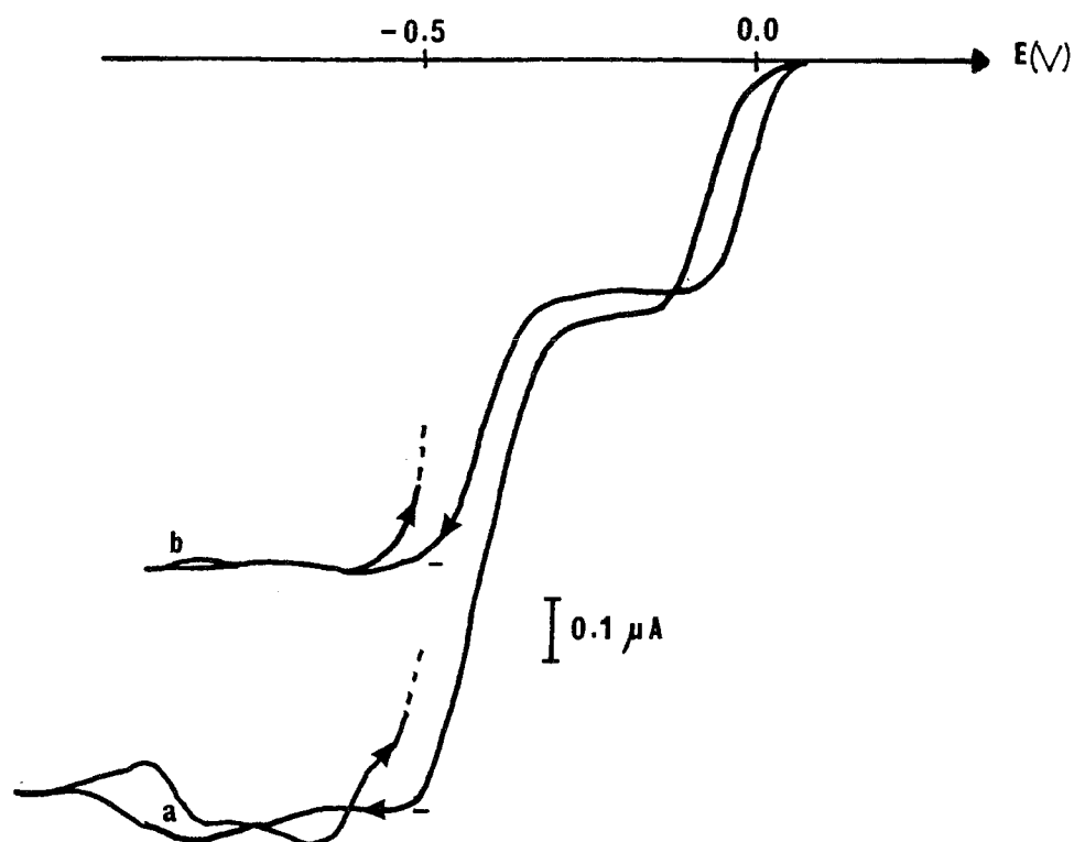
Fig.51 : Réduction de \text{CuSO}_4 5.10^{-4} M dans \text{CH}_3\text{CN-H}_2\text{O} (2-98%), Hg goutte stationnaire, réf. ECS, 2 \text{ mV}\cdot\text{s}^{-1} , (a) sans électrolyte, (b) avec \text{NaClO}_4 10^{-1} M
