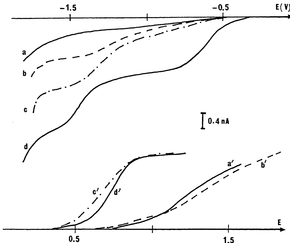
Fig.93 : Tracés cathodiques et anodiques de l'addition de HDEDTP sur une solution de TOA dans \text{CH}_2\text{Cl}_2 sat. \text{H}_2\text{O} , UME Pt, \text{N}_2 après chaque ajout, 20\text{ mV}\cdot\text{s}^{-1} , Réf. ECS pont éthanol, \text{Bu}_4\text{NClO}_4 10^{-2}\text{ M} , (a, a') TOA 6,3\cdot 10^{-4}\text{ M} , (b, b') TOA 6,3\cdot 10^{-4}\text{ M} + HDEDTP 3\cdot 10^{-4}\text{ M} , (c, c') TOA 6,3\cdot 10^{-4}\text{ M} + HDEDTP 6,1\cdot 10^{-4}\text{ M} , (d, d') TOA 6,3\cdot 10^{-4}\text{ M} + HDEDTP 8,3\cdot 10^{-4}\text{ M}
