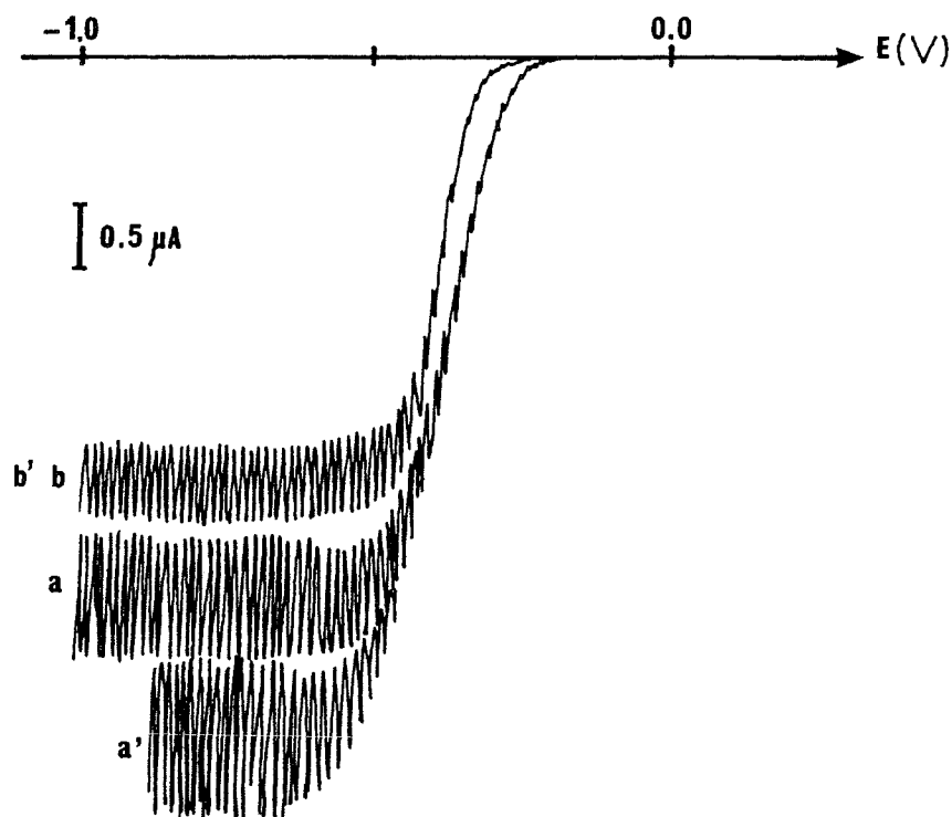
Fig.42 : courbes i-E de la réduction du \text{CuClO}_4 10^{-3} M dans \text{CH}_3\text{CN} 50%, Hg goutte tombante, réf. ECS, (a) sans électrolyte, (b) avec \text{NaClO}_4 10^{-1} M autre solution (a') sans électrolyte, (b') avec \text{NaClO}_4 10^{-1} M
