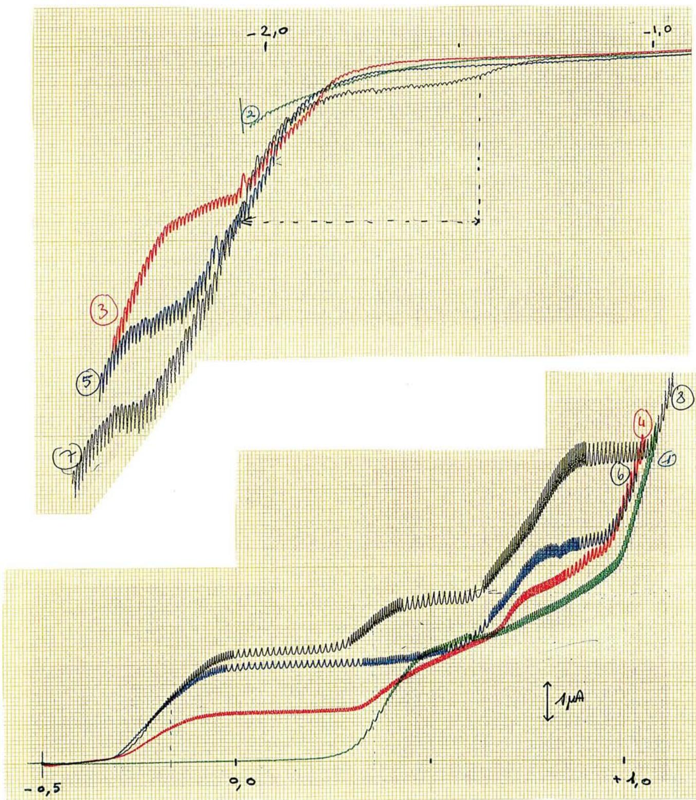
Fig. 96: Tracés anodiques et cathodiques de l'addition de HDEDTP à une solution de TOA dans \text{CH}_2\text{Cl}_2 sat. \text{H}_2\text{O} + \text{Bu}_4\text{NClO}_4 10^{-2} M sur une électrode à goutte de Hg tombante, Réf. ECS pont éthanol, 5 \text{ mV}\cdot\text{s}^{-1} , (1-2) TOA 6,5 \cdot 10^{-4} M, (3-4) TOA 6,5 \cdot 10^{-4} M + HDEDTP 3 \cdot 10^{-4} M, (5-6) TOA 6,5 \cdot 10^{-4} M + HDEDTP 6 \cdot 10^{-4} M, (7-8) TOA 6,5 \cdot 10^{-4} M + HDEDTP 8,3 \cdot 10^{-4} M
