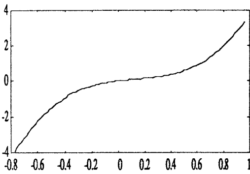
Figure 3.14 : caractéristique NL
