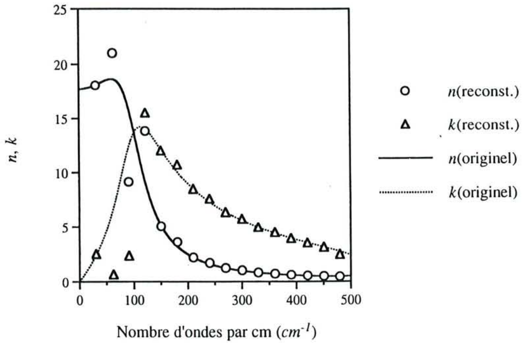
Fig. II-7-a. Constantes optiques originelles et reconstituées de SrTiO 3 jusqu'à 500 cm -1 .
