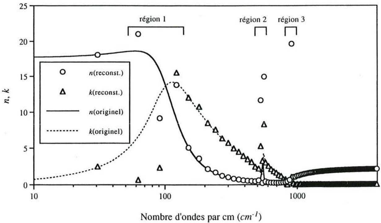
Fig. II-7-b. Constantes optiques originelles et reconstituées de SrTiO 3 jusqu'à 4000 cm -1 . (échelle logarithmique)
