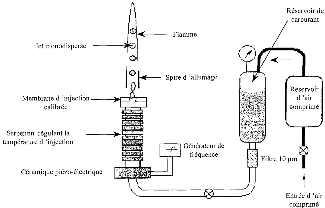
Figure IV-6 : Dispositif d'injection.
