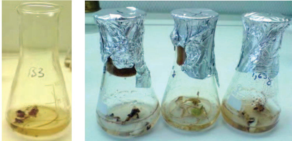
Figure 66 : Des cultures témoins et trois répétitions pour chaque concentration de précurseur deutéré.
