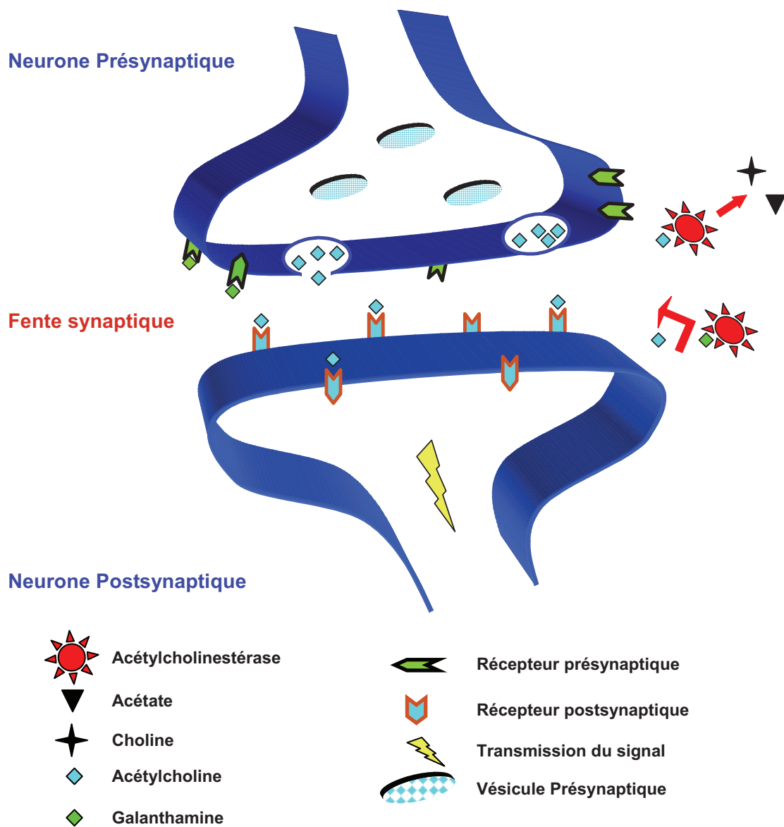
Figure 1: Mode d'action de la galanthamine : Inhibition de l'AChE, modulation allostérique des récepteurs nicotiniens et correction du déficit cholinergique.
