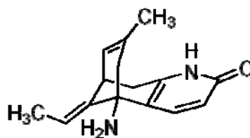
Figure 3 : Structure chimique de l'hupérezine A.
