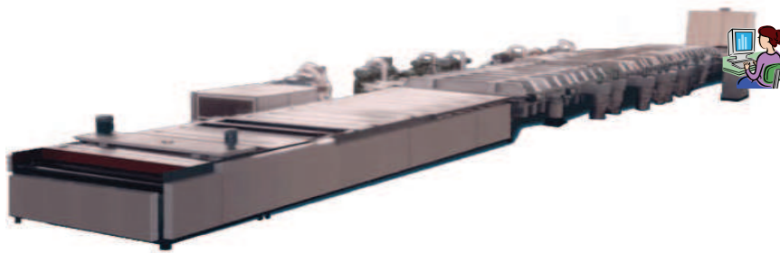
FIG. 2.8 – b/ Exemple de ligne de production industrielle de pulvérisation magnétron pour l'industrie du verre ( ETA Film Technology Inc. , Taiwan).
