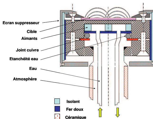
FIG. 3.9 - Schéma du magnétron modifié avec écran suppresseur en aluminium et jupe extérieure de fer doux pour guider les lignes de champ magnétique.
