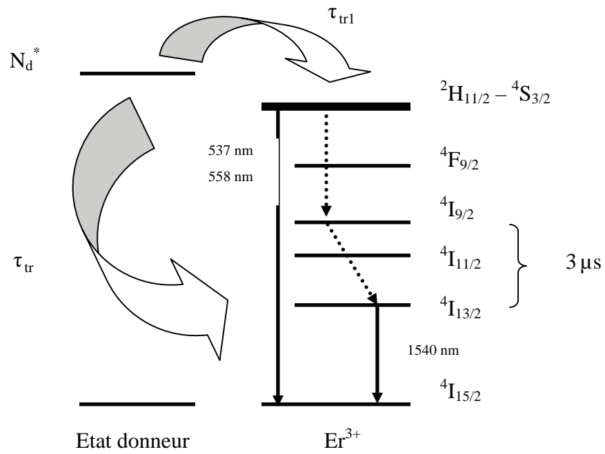
FIG. 4.22 – Modèle de transfert de l'énergie via des états électroniques de l'erbium d'énergie supérieure à celle du niveau 4\text{I}_{13/2} .
