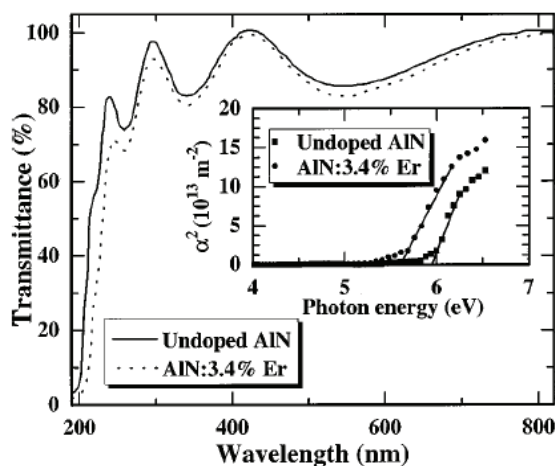
FIG. 1.6 - Les spectres de transmission optique de l'AlN non dopé et dopé Er. L'insert montre \alpha^2 en fonction de l'énergie des photons pour les mêmes films [88].
