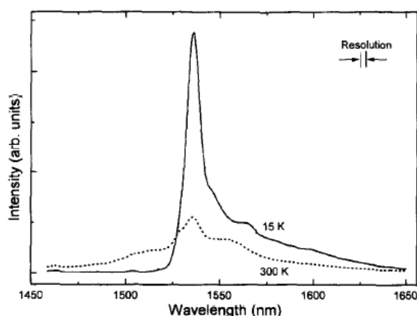
FIG. 1.13 - Spectres de photoluminescence de films d'AlN dopés Er à 15 and 300K [91].
