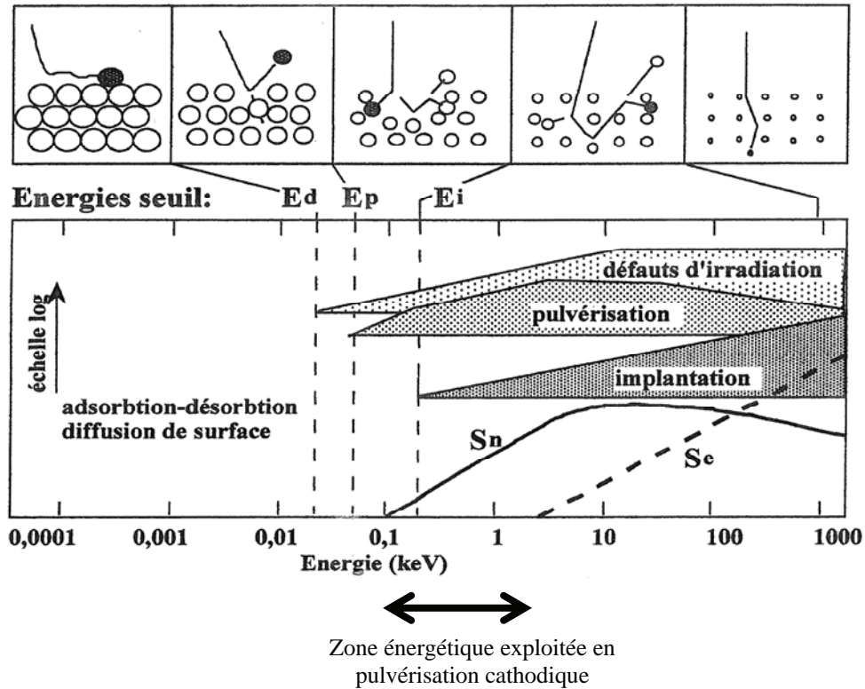
FIG. 2.2 – Mécanismes élémentaires intervenant lors de l'interaction d'un ion avec une surface solide. Ed : Energie seuil de déplacement, Ep : Energie seuil de pulverisation, Ei : Energie seuil d'implantation, Sn : Ralentissement nucléaire, Se : Ralentissement électronique.
