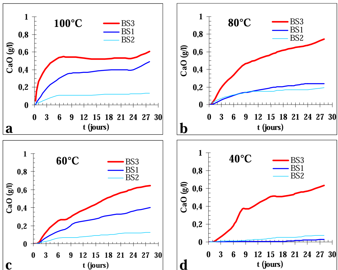
Fig. 3. 7 : Concentration de la chaux dans le bain aqueux en fonction de la teneur en chaux libre/temps
