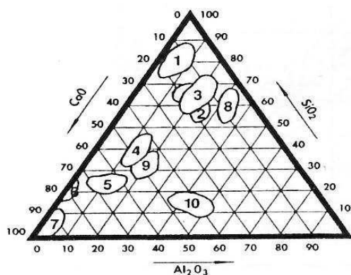
Fig. 1. 11 : Diagramme ternaire CaO - SiO 2 - Al 2 O 3
