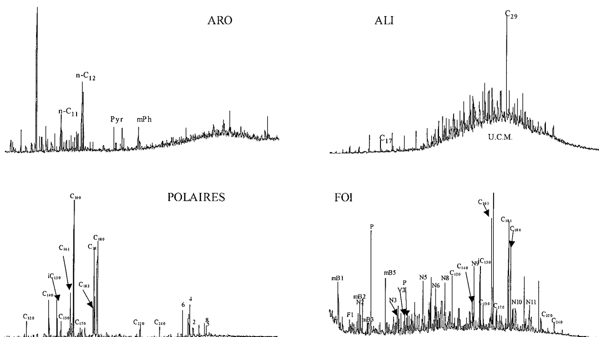
Figure III.3.3. Chromatogrammes des fractions aromatiques, aliphatiques, polaires et pyrogramme du résidu solide de l'échantillon U1.
