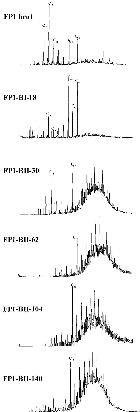
Figure III.3.12 Chromatogrammes des n-alcane ( m/z = 85 ) de la boue de laiterie FP1 (de FP1 brut à FP1-BII-140)
