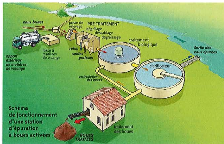
Figure I.3. Schéma de fonctionnement d'une station d'épuration à boues activées (d'après « les boues d'épuration municipales et leur utilisation en agriculture » élaboré par le Comité Technique Permanent sur l'épandage des boues d'épuration et édité par l'ADEME)
