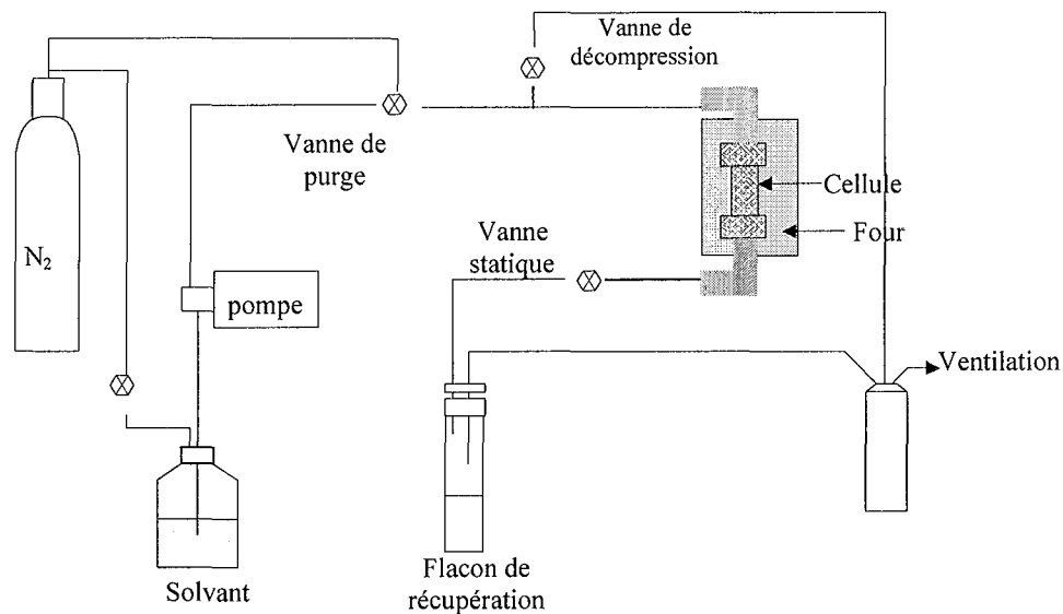
Figure II.1. Appareillage mis en œuvre pour l'extraction accélérée par solvants
