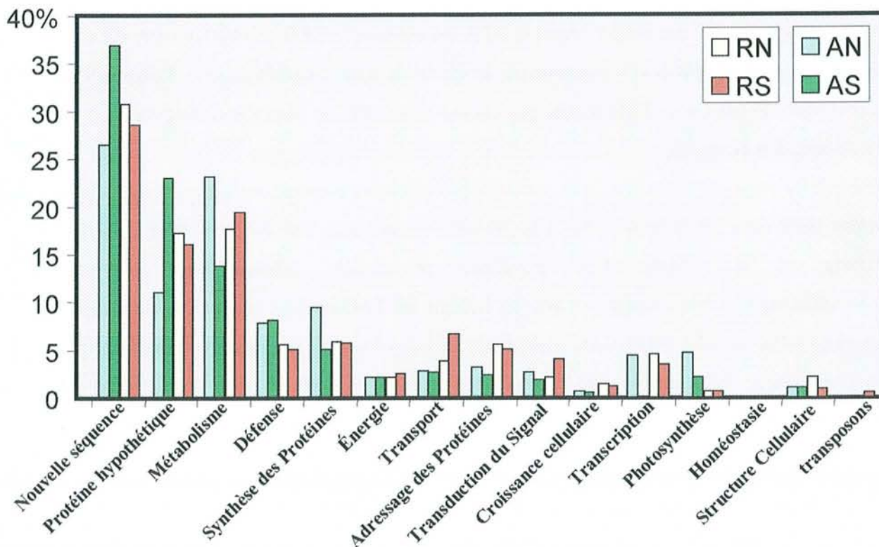
Figure 19 : Classement des différentes EST séquencées provenant de chacune des quatre banques d'ADNc (A: aiguilles, R: racines, S: stressées, N: non-stressées) selon leur fonction cellulaire. (Classement selon Bohnert et al., http://stress-genomics.org/ ; séquences: J-M Frigerio, non publiées ).
