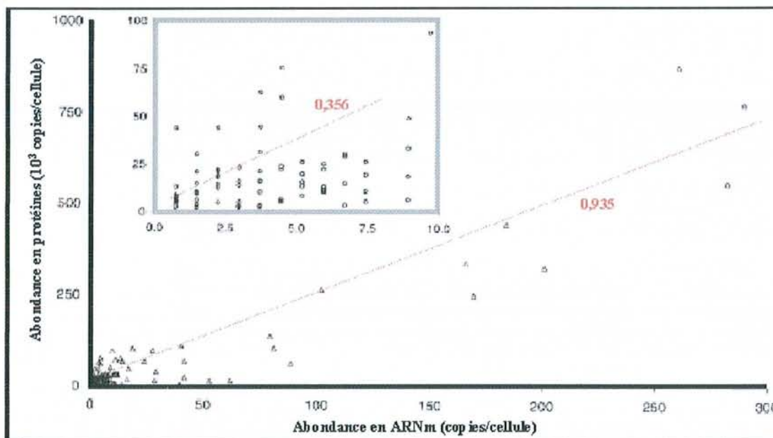
Figure 20 : Corrélation entre les niveaux d'accumulation de protéines et d'ARNm pour 106 gènes de levure en phase exponentielle de croissance (d'après Gygi et al., 1999). Les protéines analysées ont été isolées par 2-DE et choisies sur toute la gamme de poids moléculaire et de point isoélectrique. Dans l'encadré sont représentées les variations de 69% des gènes analysés dans le graphique principal. Les droites en pointillés rouges représentent les coefficients de corrélation de Pearson, dans chacun des 2 cas.
