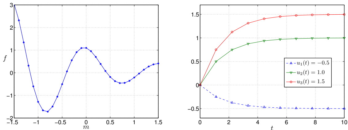
Figure 1.4 – Élément statique non linéaire (à gauche) et réponses impulsionnelles de l'élément dynamique linéaire (à droite)
