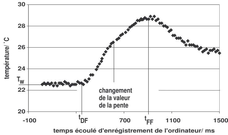
FIG. B.4 – Signal émis par le thermocouple lors d'une mesure du flux à l'aide du komef.
