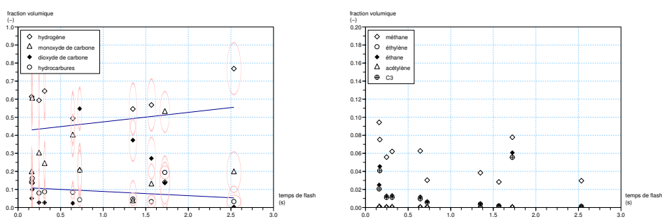
FIG. 4.22 – Composition de gaz pour la lignine Kraft Borregaard .
