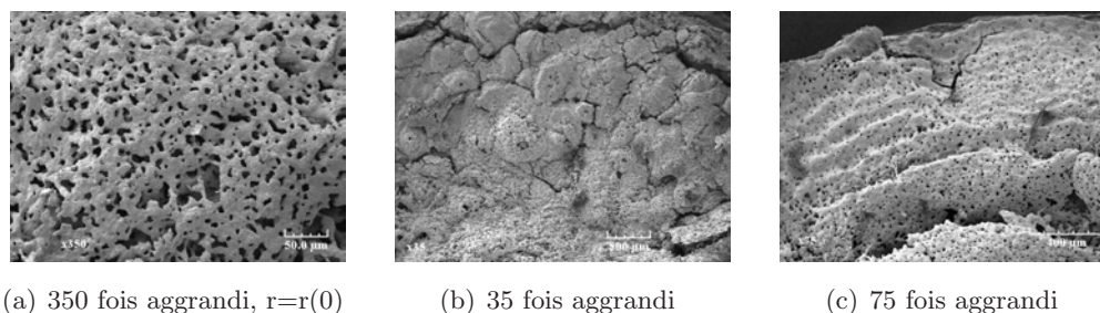
FIG. 4.12 – Pyrolyse complète d'une pastille de xylane.
