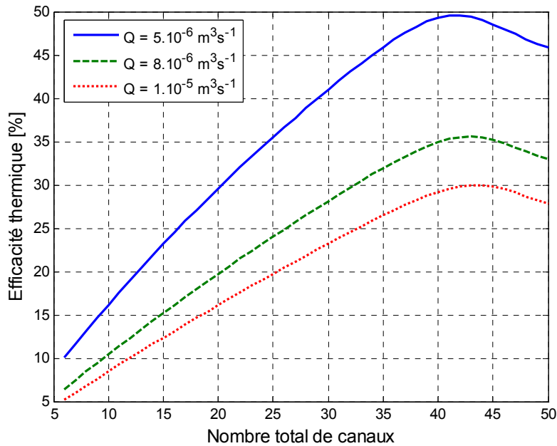
Figure IV.5. Efficacité globale calculée pour différentes configurations à deux échelles présentant la même surface d'échange à différents débits d'entrée.
