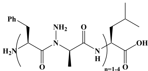
Figure 49 Formule générale des oligomères
