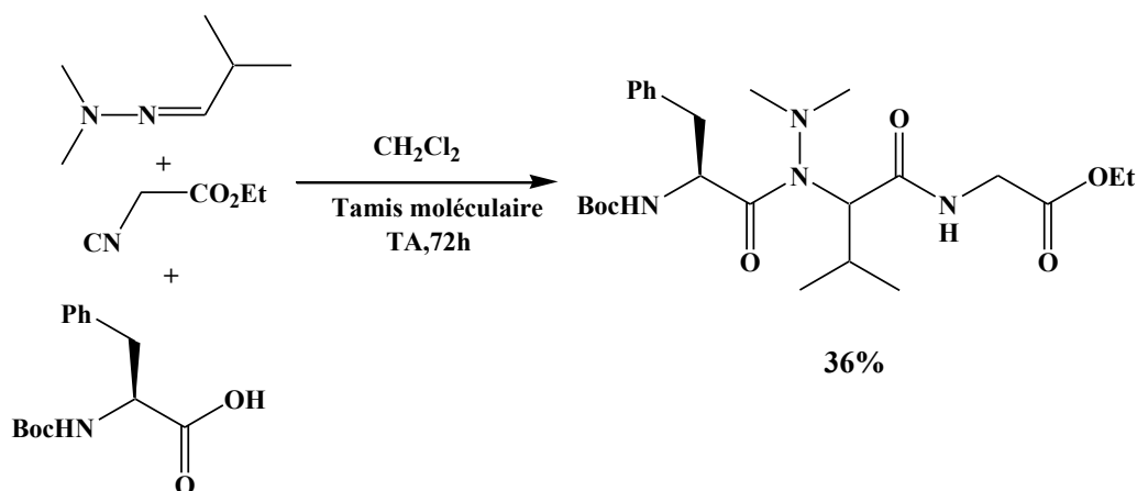
Schéma 5 Synthèse d'un N -aminotriptide
