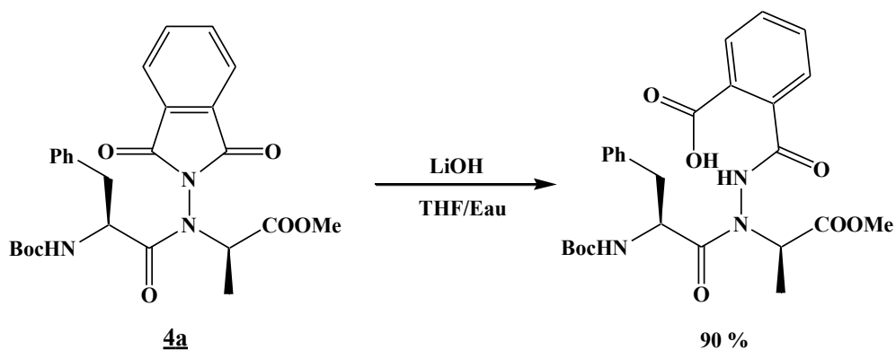
Schéma 20 Ouverture du phtalimide d'un N -aminodipeptide
