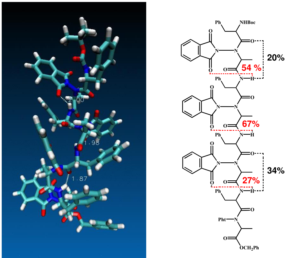
Figure 117 Une structure 3D de l'octamère 13b obtenue par dynamique moléculaire avec la distance O-H et pourcentage de probabilité de présence des liaisons hydrogène
