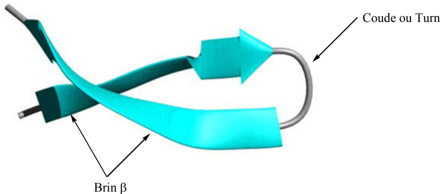
Figure 19 Représentation 3D d'un \beta -hairpin
