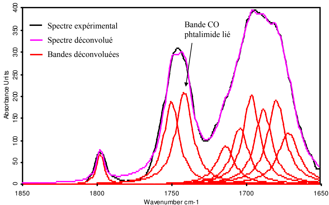
Figure 134 Spectre IR déconvolué de la zone CO du composé 31
