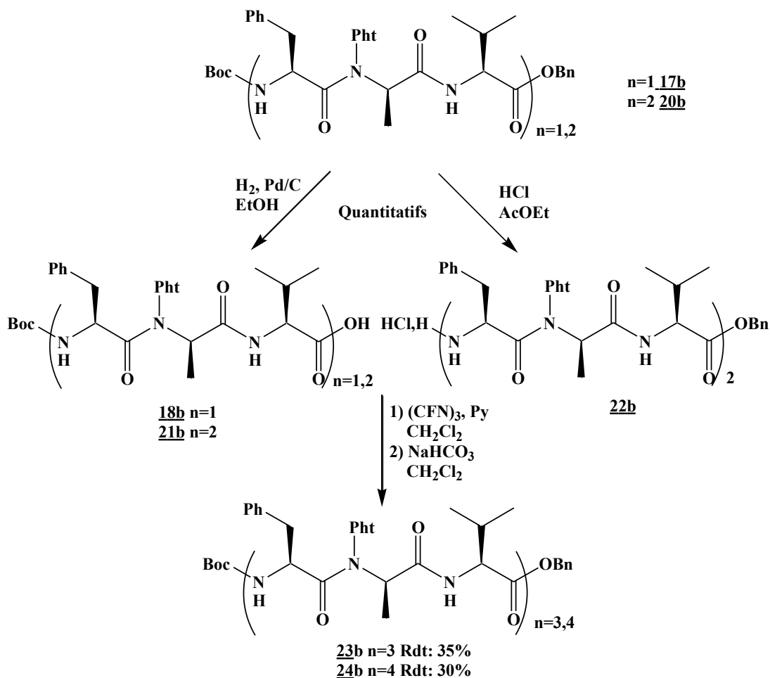
Schéma 39 Synthèse des 2:1 [α/α-N-amino]mères à 9 et 12 résidus
