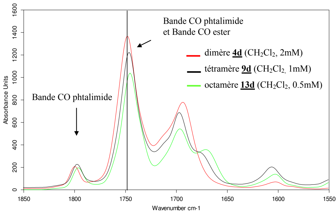
Figure 105 Spectre IR: zone des vibrateurs CO des oligomères 4d , 9d et 13d
