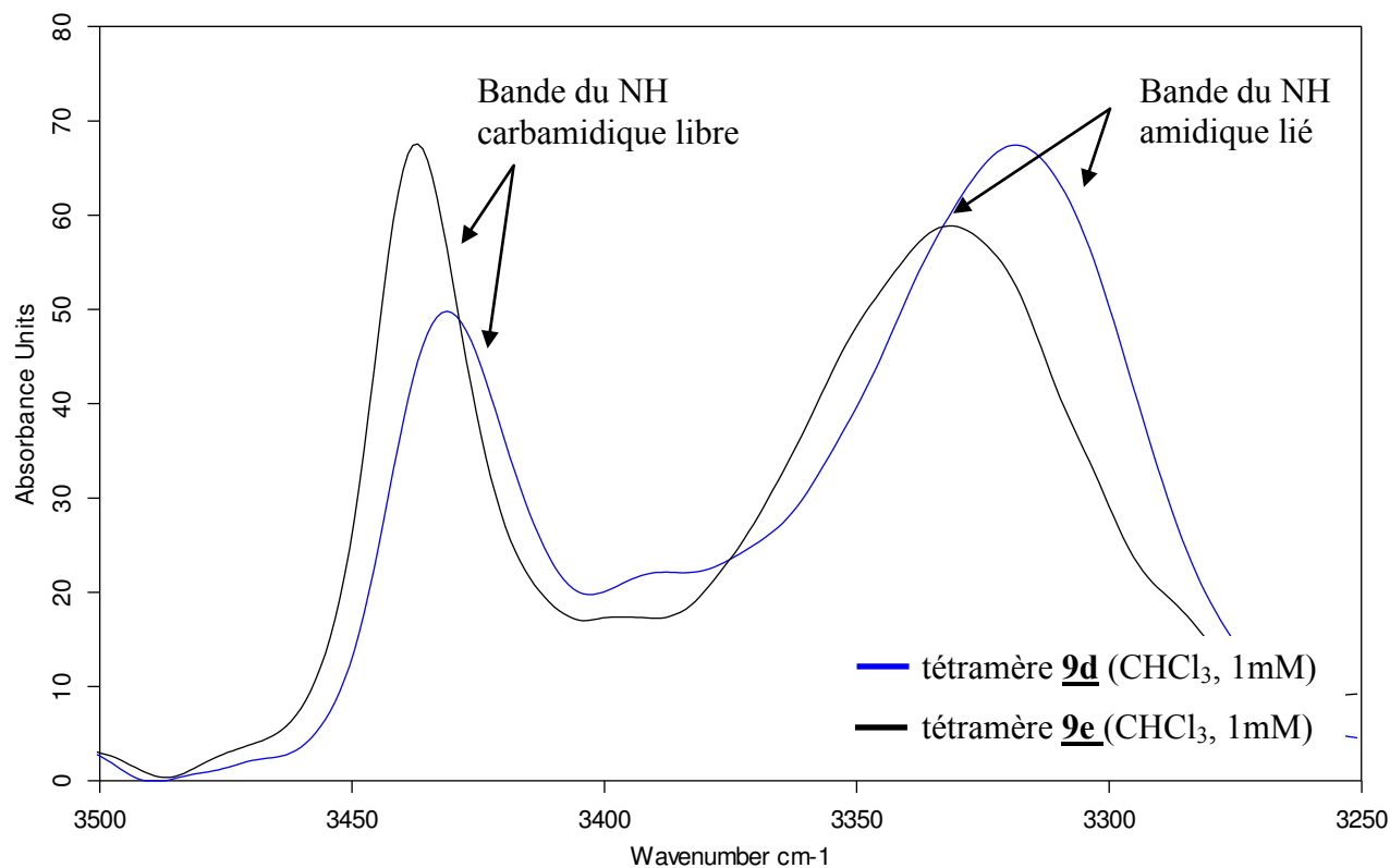
Figure 70 Spectres IR: zone des vibrateurs NH des tétramères 9d et 9e
