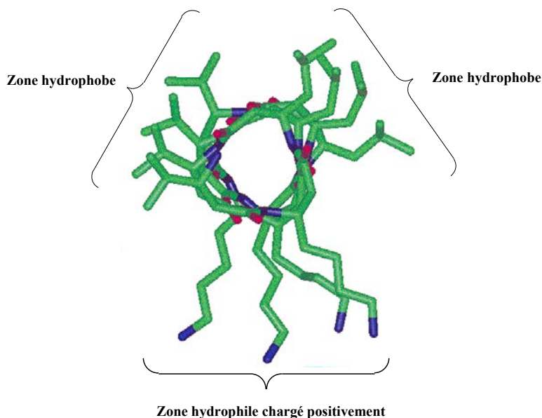
Figure 32 Modèle moléculaire de l'hélice 3 14 (Leucine, Valine, Lysine)
