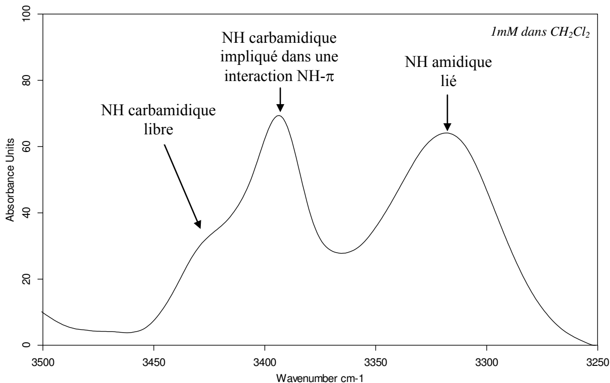
Figure 72 Spectre IR: zone des vibrateurs NH du tétramère 9b
