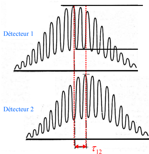
Figure 4.4 Mesure du déphasage de deux bouffées Doppler
