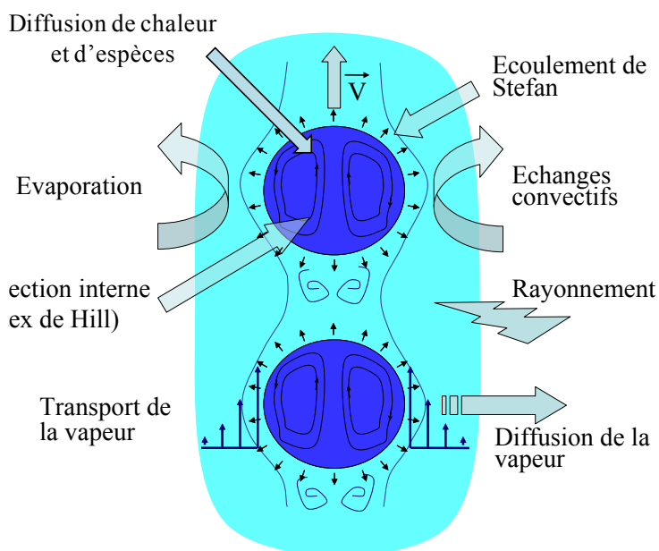
Figure 1.1 Phénomènes intervenant dans l'évaporation de gouttes
